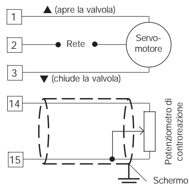
Fig. 8 COLLEGAMENTO DELL'USCITA PER SERVOMOTORE
