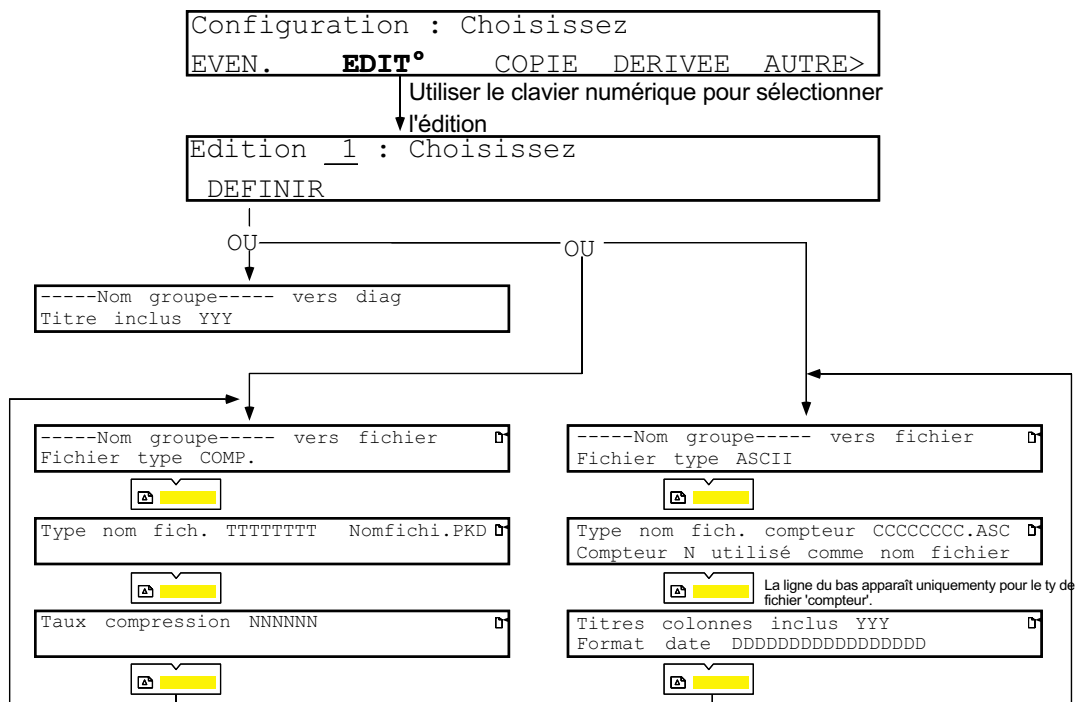
Figure 4.8 Configuration d'éditions
