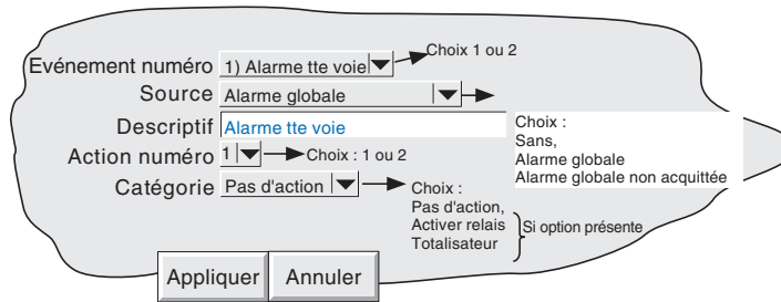
Figure 4.3.5 Menu de configuration d'événement
