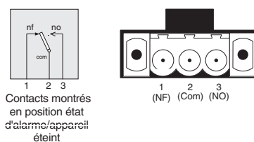
Figure 2.2.1c Emplacement des connecteurs - 180 mm
