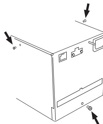
Figure 7.3.2b Emplacement des vis
