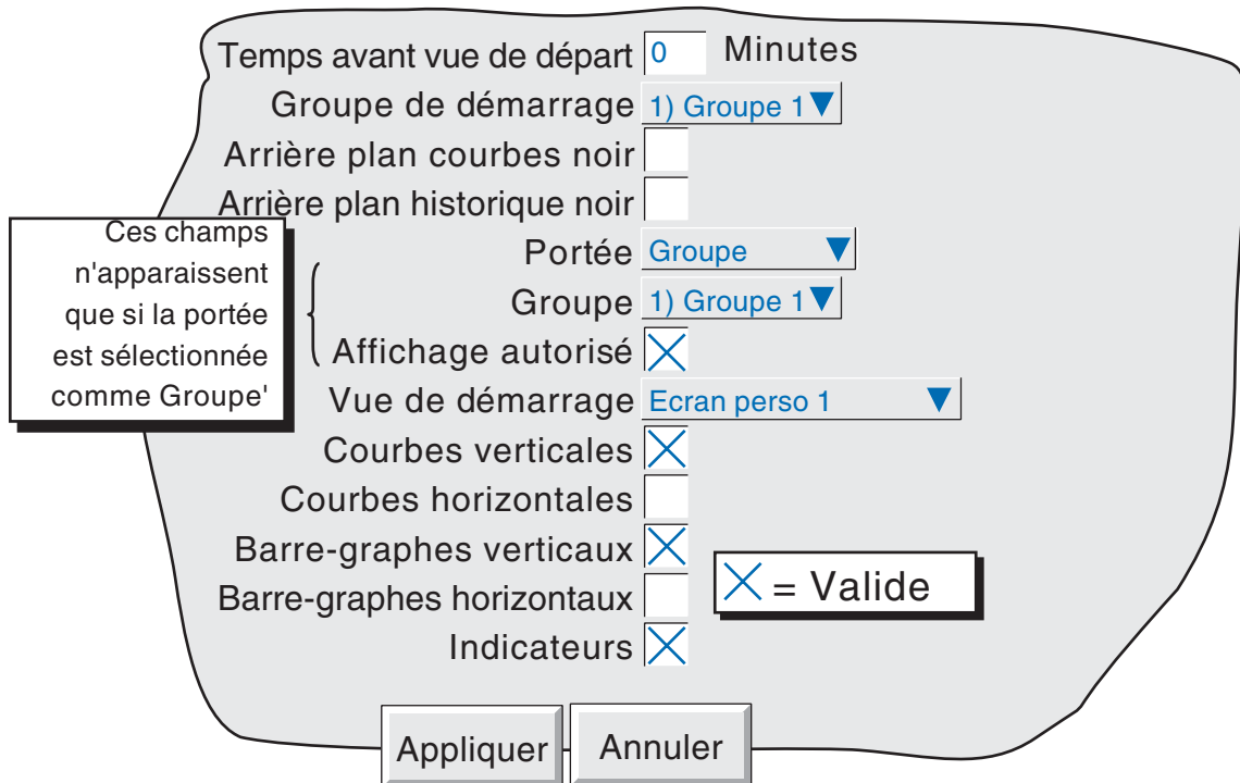
Figure 4.3.4 Menu de configuration des vues
