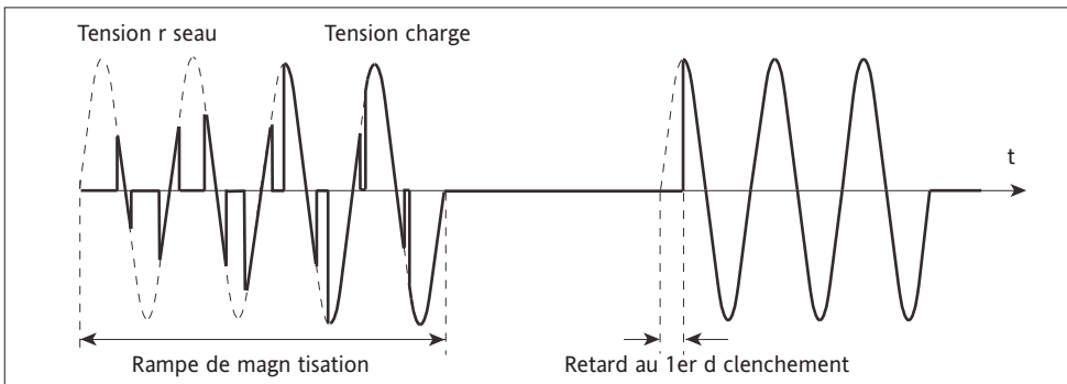
Figure 3-8 Mise sous tension des primaires des transformateurs en «Train d'ondes» (option XFMR)
