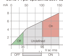
Curva V-I per operatività 230V ca
