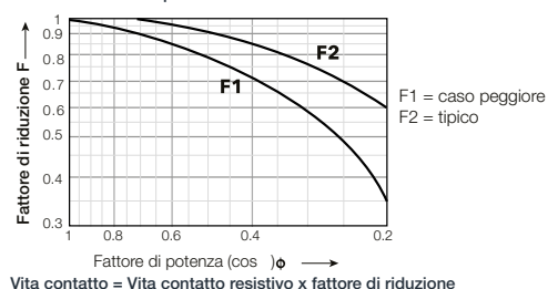
Fattore di riduzione per carichi CA resistivi
