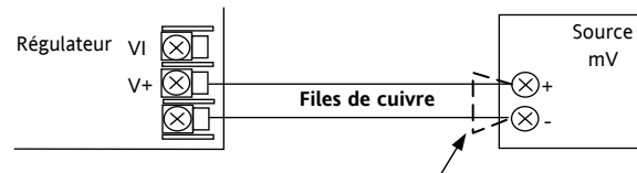
Figure 1: Connexions pour la calibration de l'entrée mV
