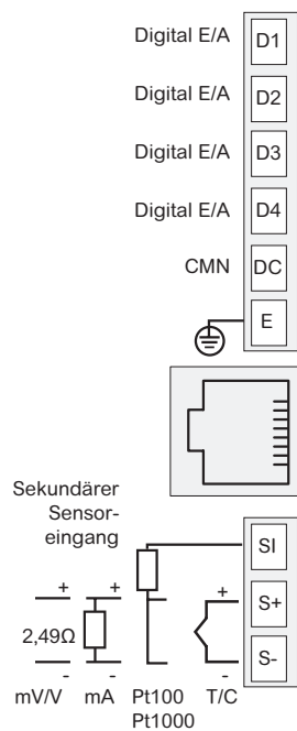
Prozesswerteingang Ethernet 4 x Digitaleingang/ Digitalausgang
