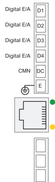
Ethernet 4 x Digitaleingang/ Digitalausgang
