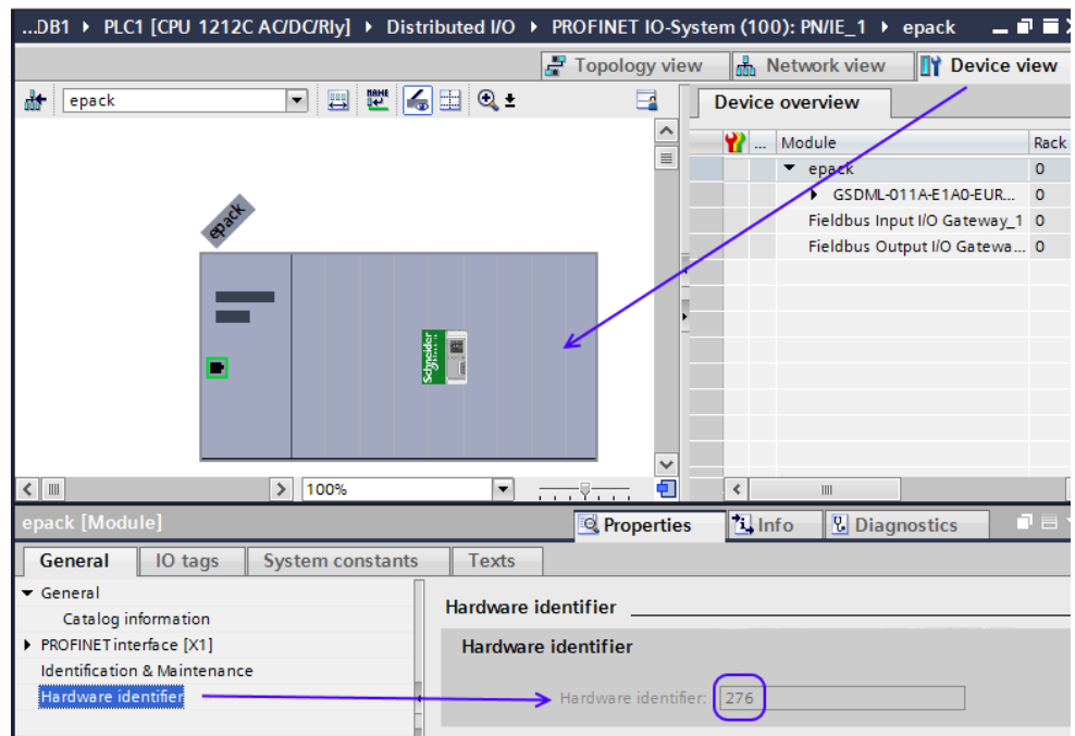
Figure 51 Valeur d'identifiant du matériel
