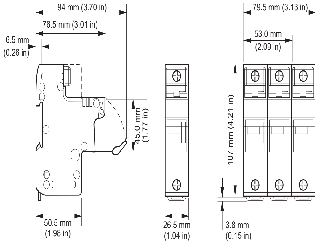
Figure 146 Dimensions des porte-fusibles : US141 (14x51 mm)
