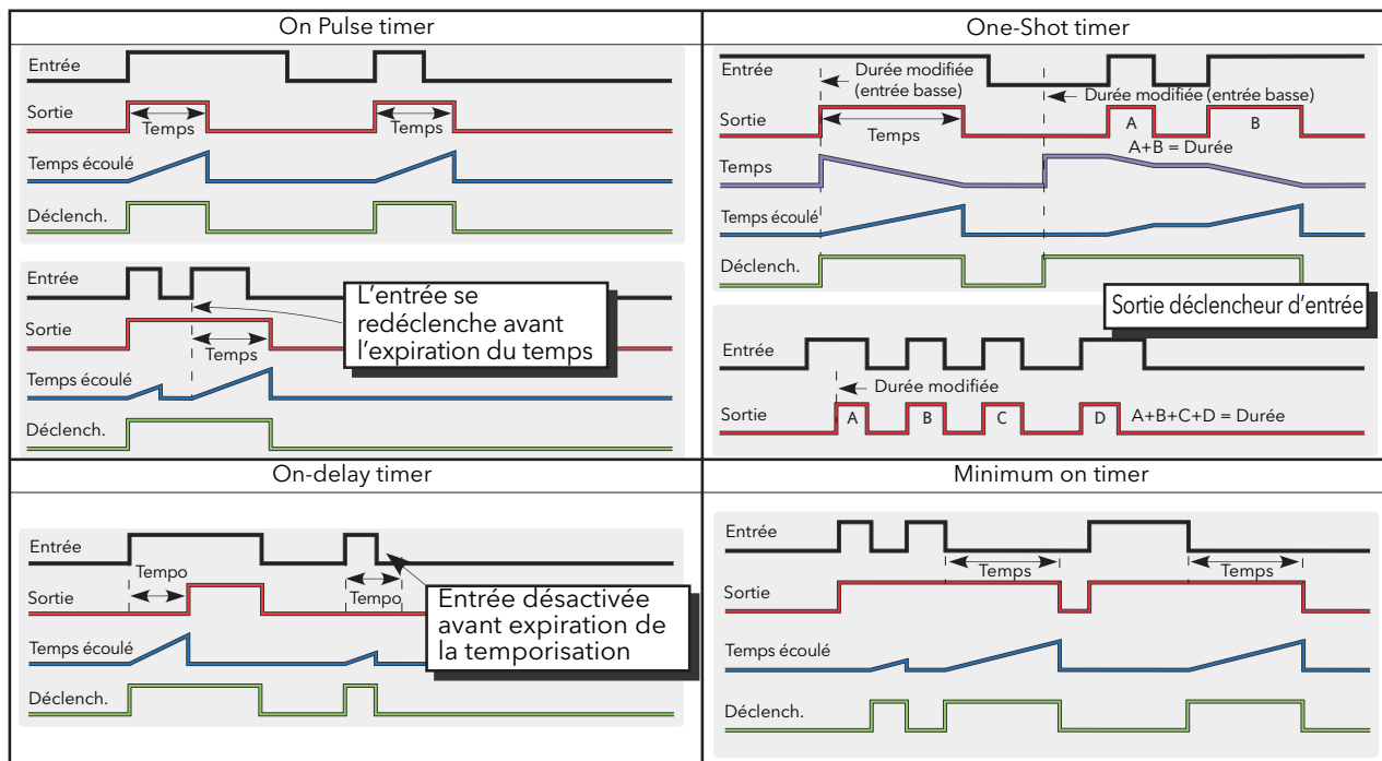
Figure 118 Exemples de temporisateur
