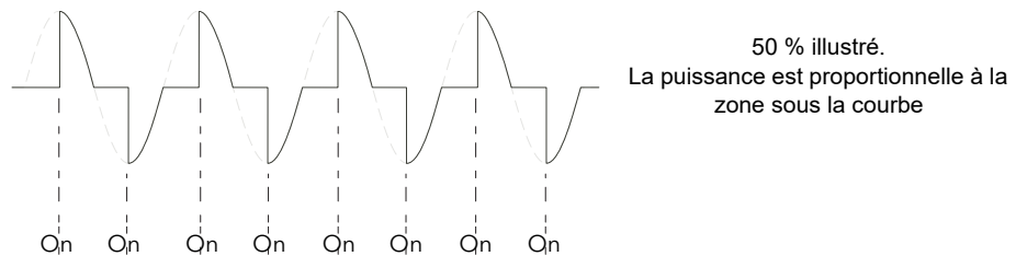
Figure 18 Mode en angle de phase
