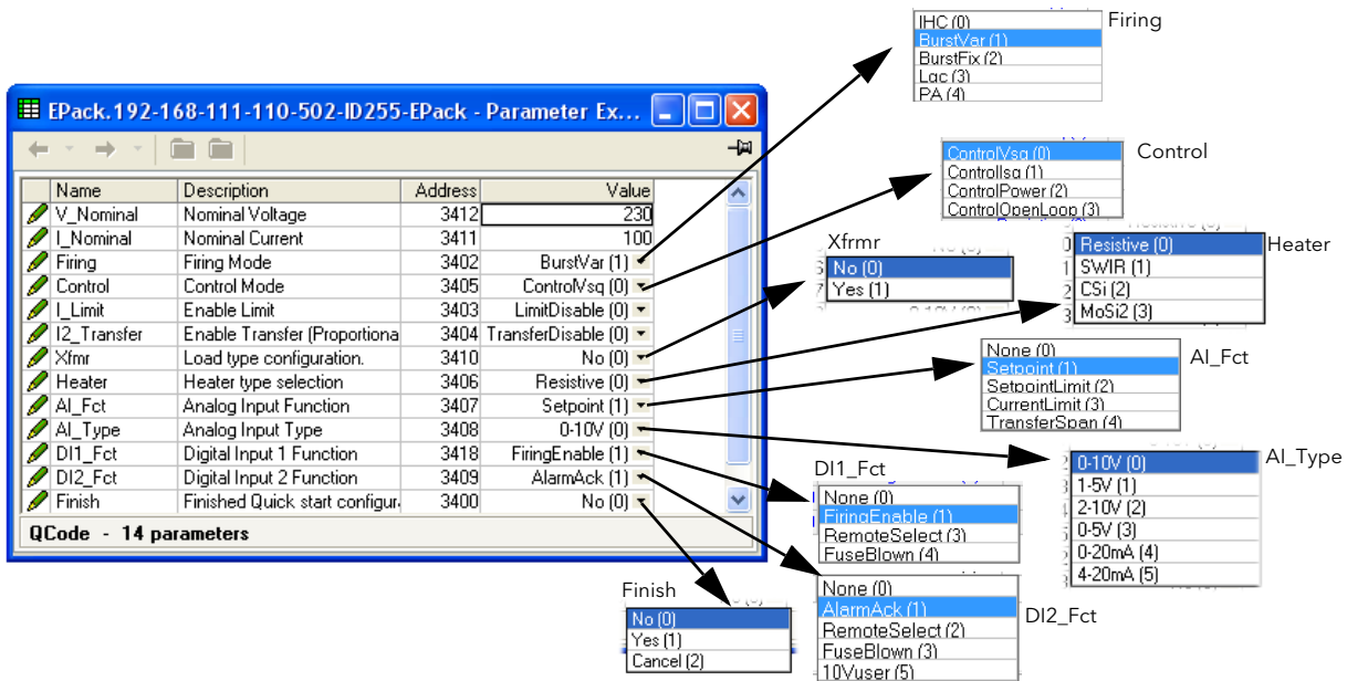
Figure 115 Paramètres Quick code
