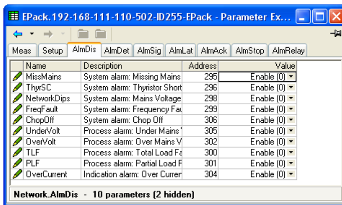
Figure 114 Page des alarmes réseau
