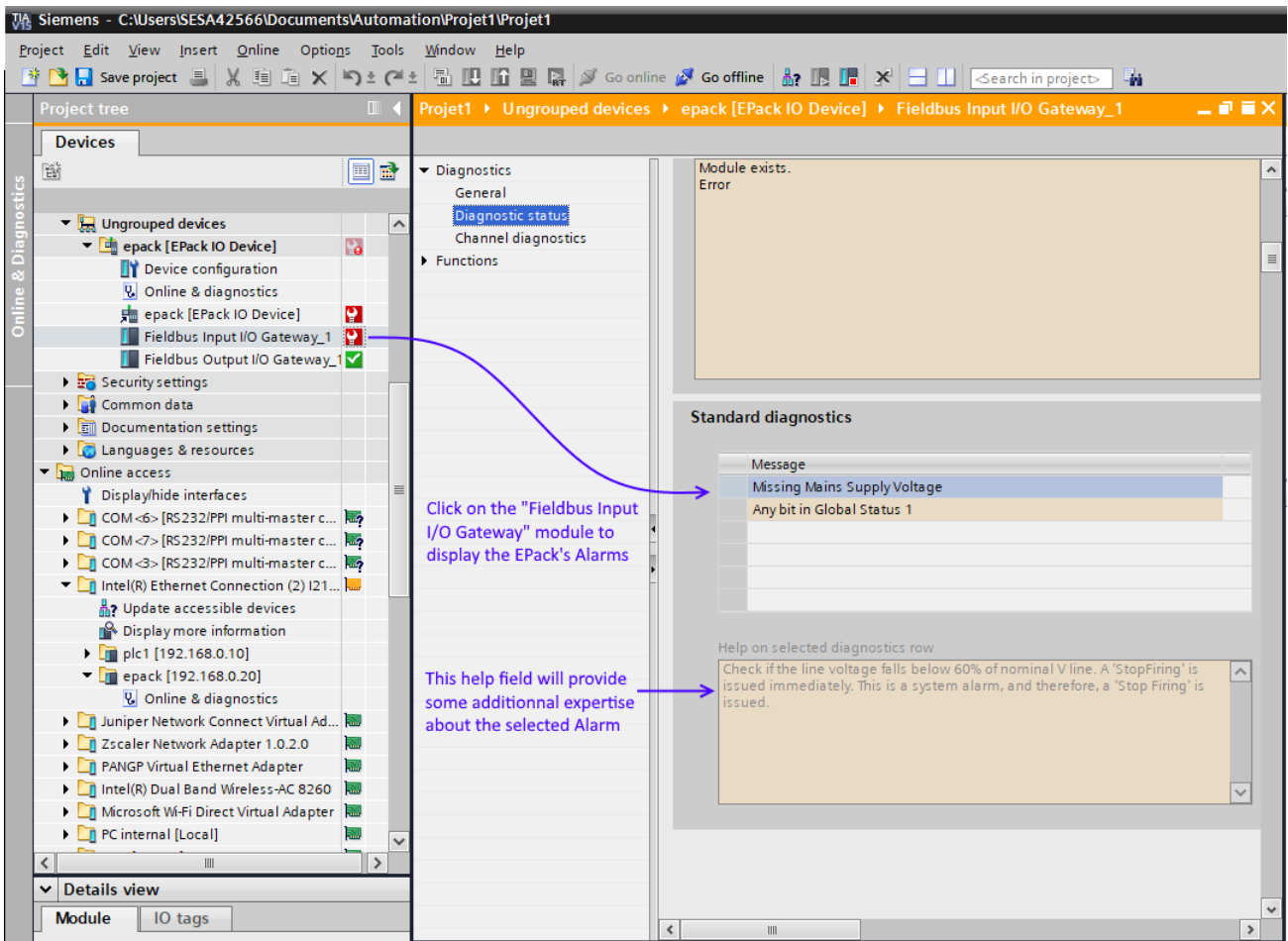
Figure 52 Capture d'écran du portail TIA représentant une alarme EPack
