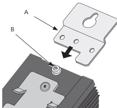
Figure 1 Installation de la fixation de montage en fond d'armoire (contrôleur 32 A présenté ; contrôleurs 63 A similaires)
