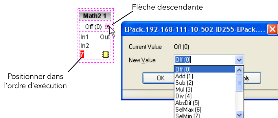
Figure 128 Exemple de bloc fonction
