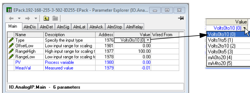
Figure 92 Page de l'entrée analogique iTools
