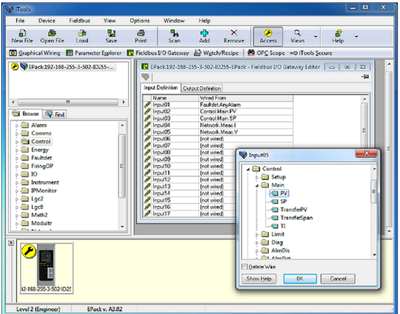
Figure 24 Sélection d'une valeur d'entrée et exemple de liste d'entrées
