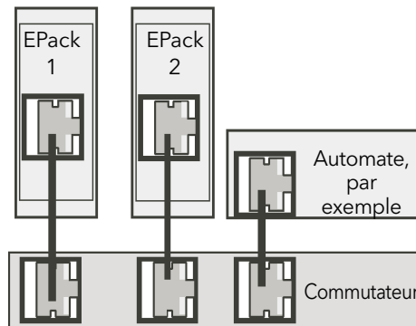
Figure 39 CÂBLAGE Profinet - Plusieurs contrôleurs
