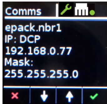
Figure 45 Affichage du nom de l'appareil sur l'EPack (par ex. « epack.nbr1 »).
