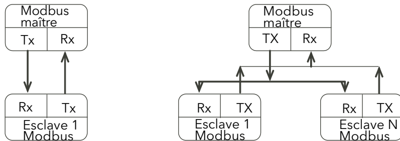
Figure 37 Connexion série simple et Connexion série multipoints
