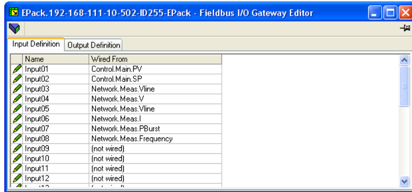
Figure 140 Liste typique des paramètres de la passerelle Fieldbus
