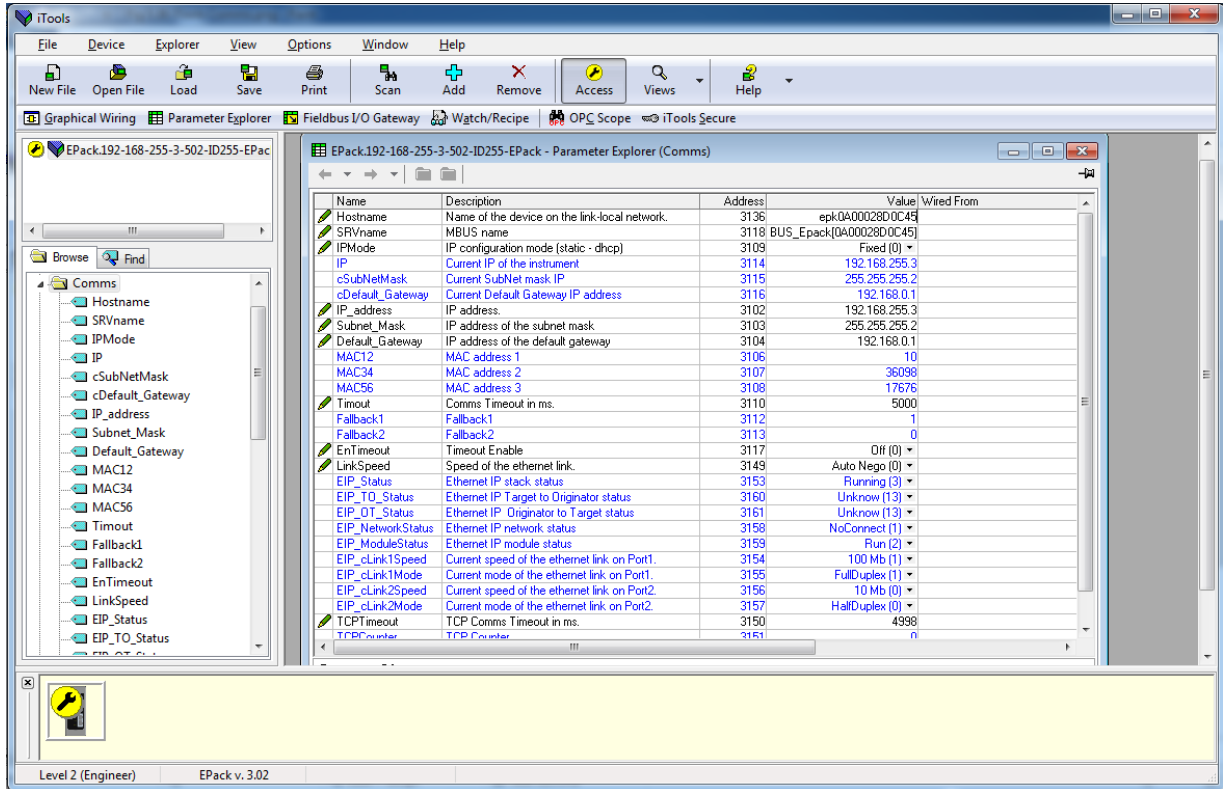
Figure 22 Paramètres de configuration Comms Utilisateur EtherNet/IP
