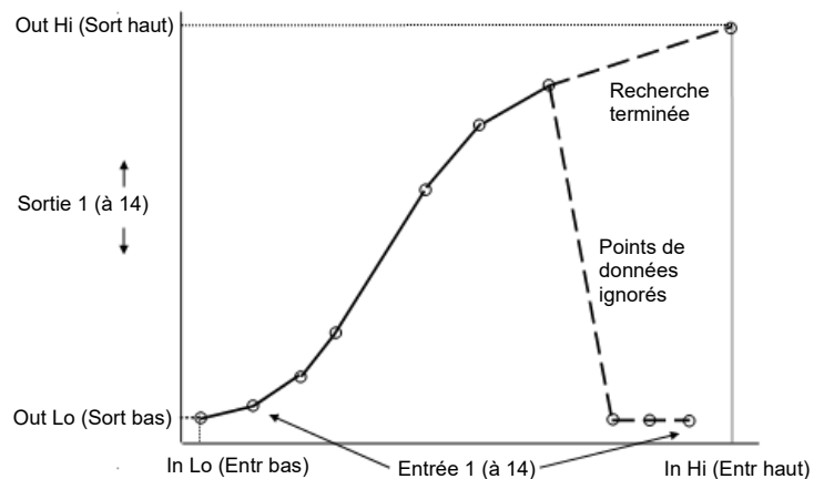
Figure 107 Exemple de linéarisation
