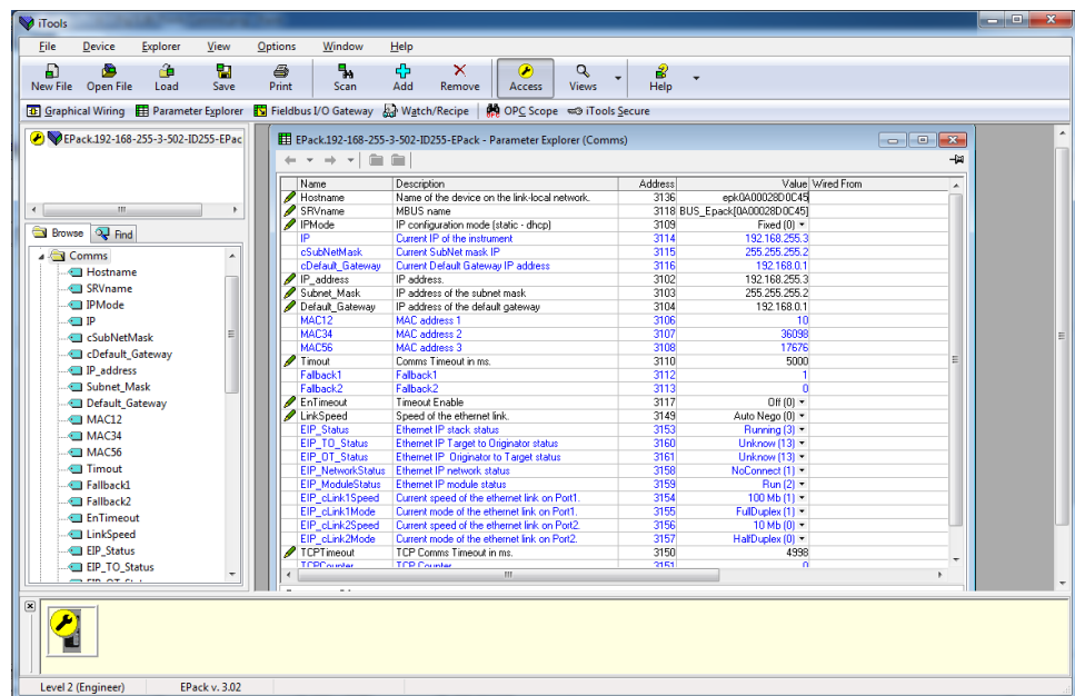
Figure 38 iTools - Paramètre de communication Ethernet
