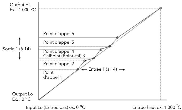
Figure 109 Compensation des discontinuités du capteur
