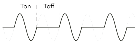
Figure 19 Mode demi-période intelligente : Période de conduction de 50 %
