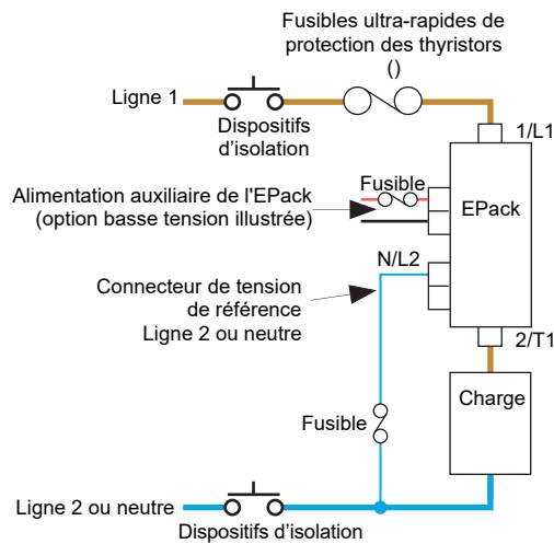
Figure 8 Détails de la connexion de puissance d'alimentation et de charge (produits 16 A à 63 A).
