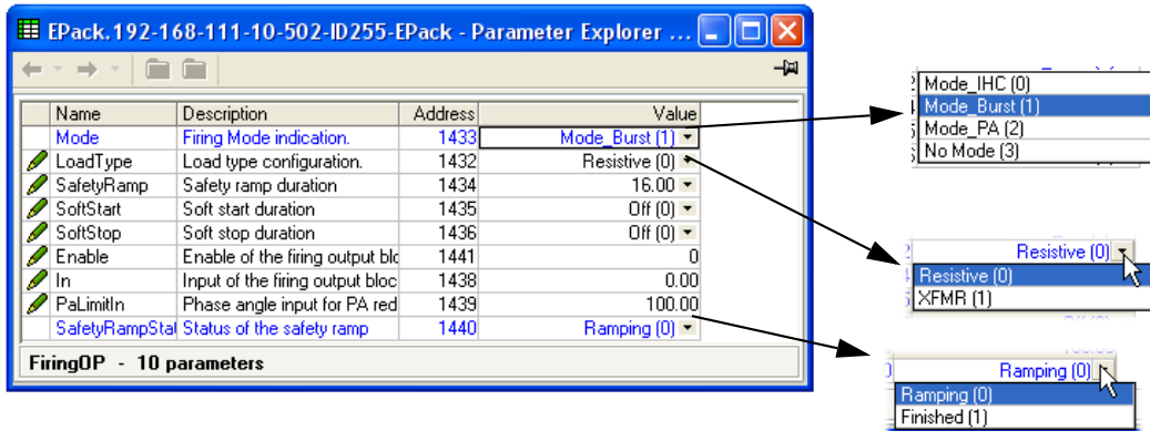
Figure 87 Page de la configuration de la sortie de conduction iTools
