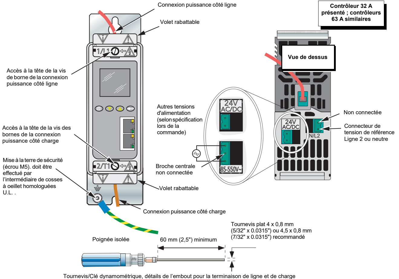
Tournevis/Clé dynamométrique, détails de l'embout pour la terminaison de ligne et de charge
