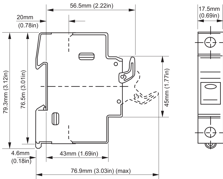
Figure 145 Dimensions du porte-fusible : CUS101 (10x38 mm)
