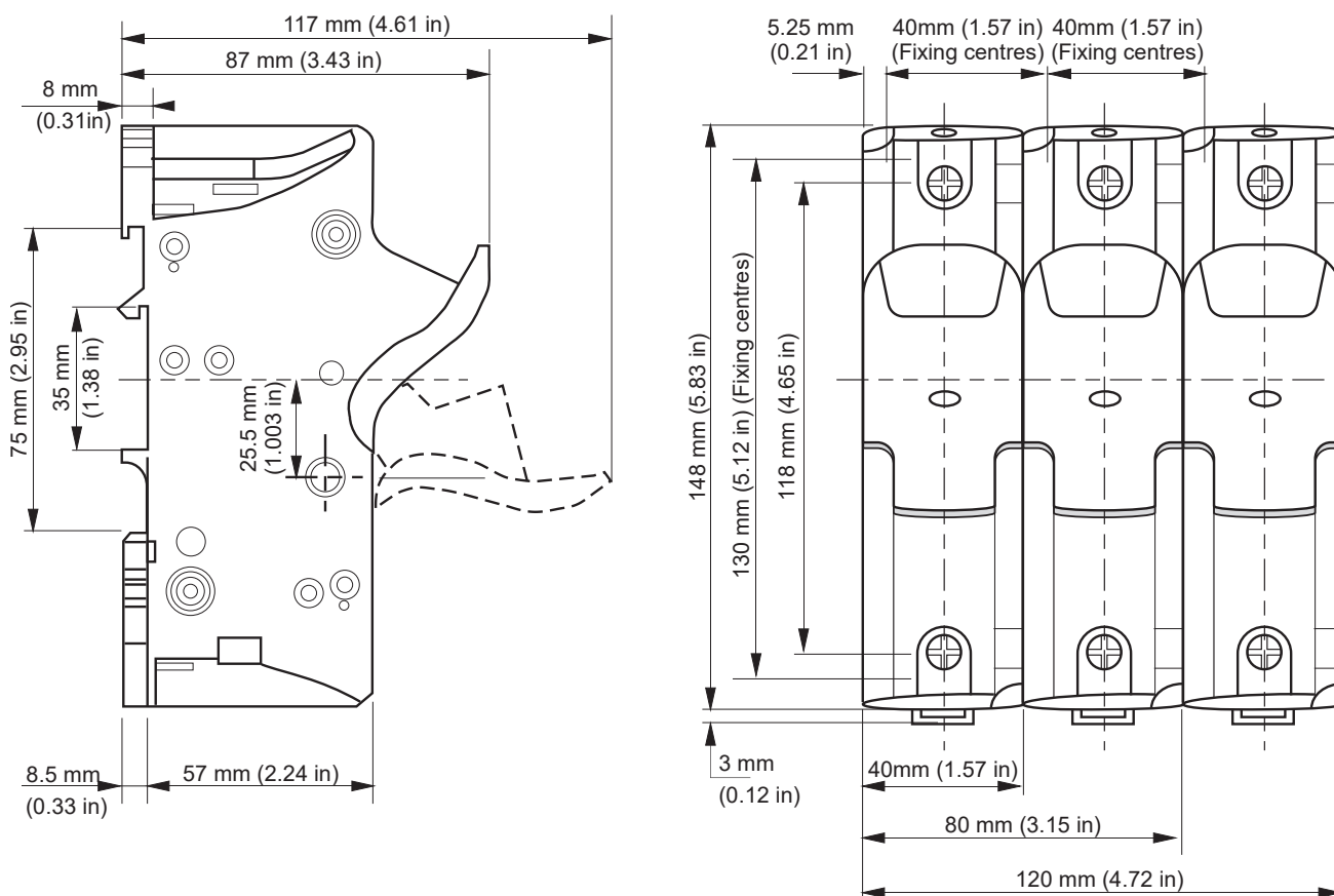
Figure 148 Dimensions des porte-fusibles : US271 (27x60 mm)
