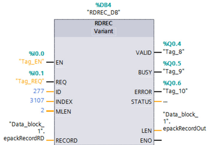
Figure 50 Lecture d'un paramètre de l'EPack, en utilisant le bloc fonction RDREC de STEP 7
