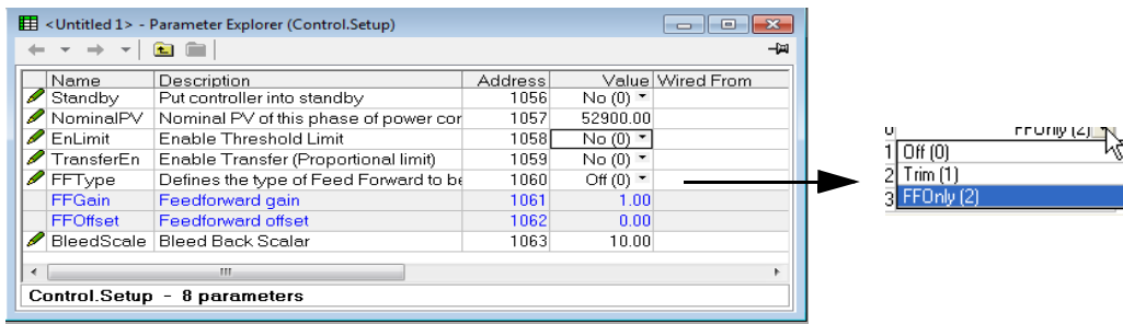
Figure 72 Page des paramètres de commande
