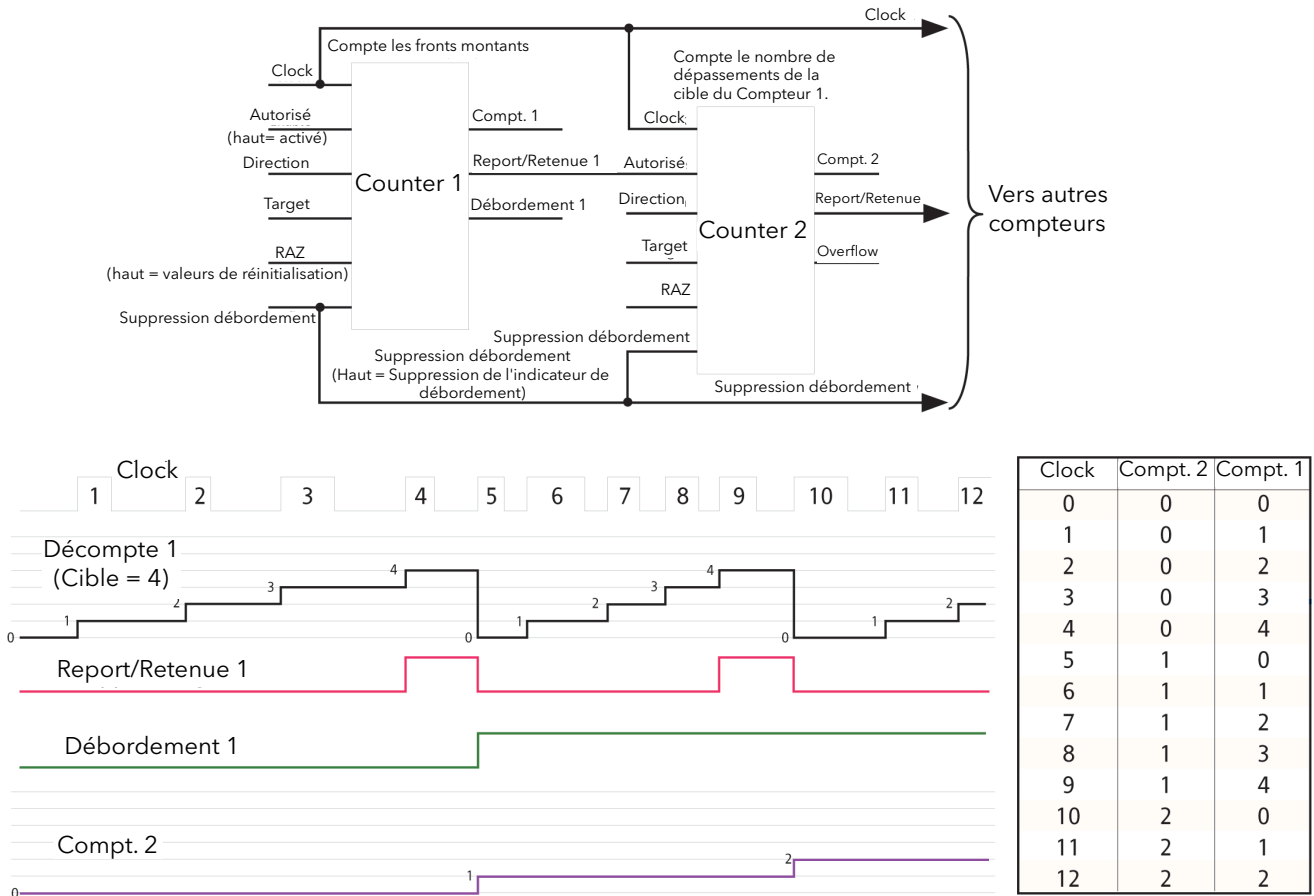
Figure 84 Mise en cascade des compteurs
