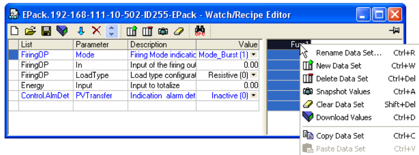
Figure 143 Fenêtre Éditeur Tableau/Recette (avec menu contextuel)
