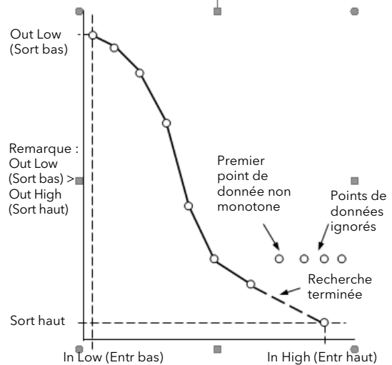
Figure 108 Manière dont une courbe inversée met fin à la recherche lorsqu'elle détecte des données non monotones
