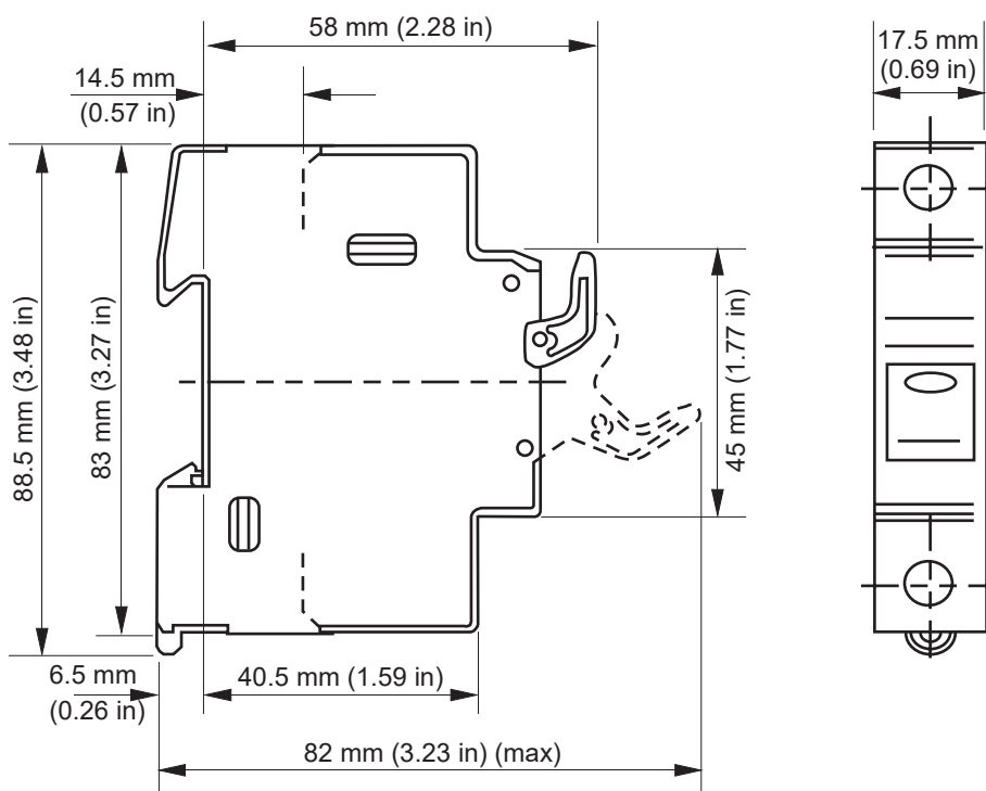
Figure 144 Dimensions des porte-fusibles : US101 (10x38 mm)
