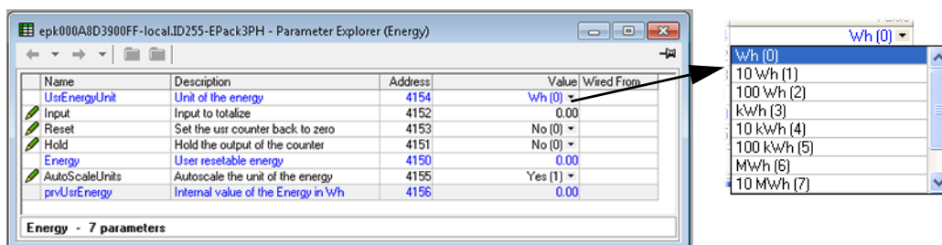
Figura 92 Pagina di configurazione dei consumi energetici
