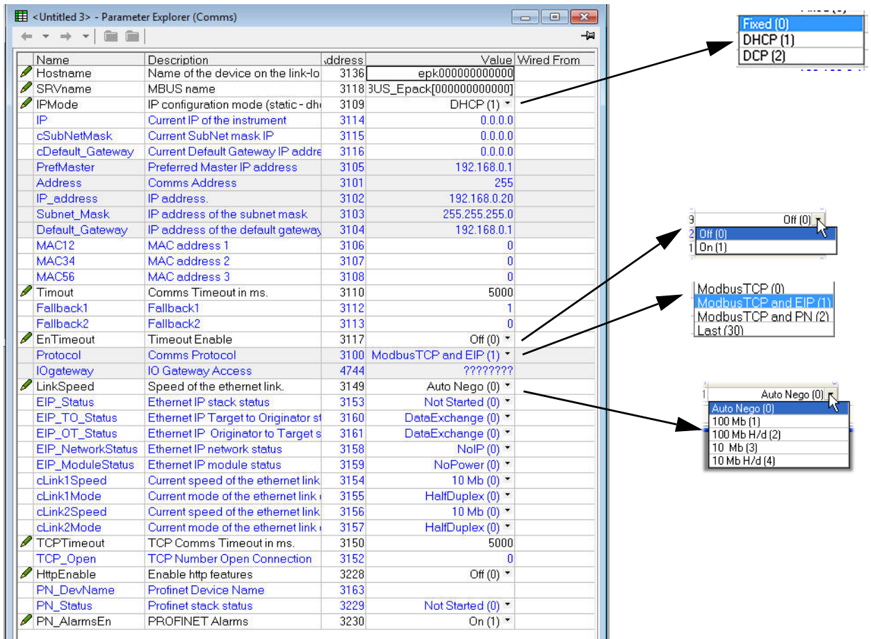
Figura 77 Pagina Comms (Comunicazioni) di iTools
