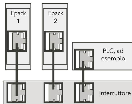
Figura 43 CABLAGGIO PROFINET - Regolatori multipli
