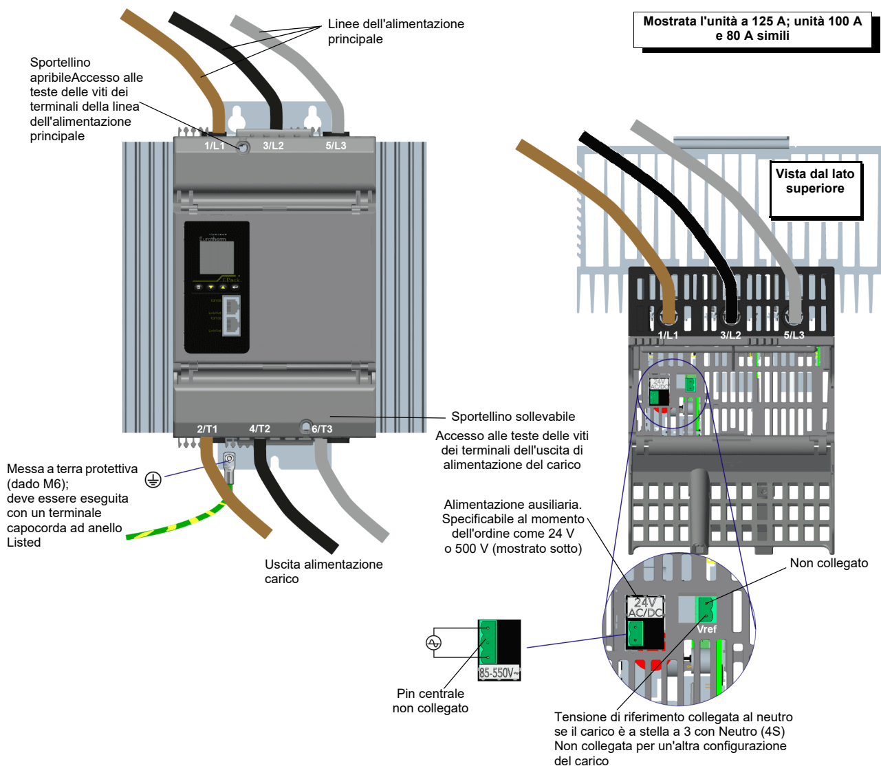
Figura 9 Dettagli su alimentazione e collegamento del carico (unità da 80 A a 125 A)(125 A visualizzata).
