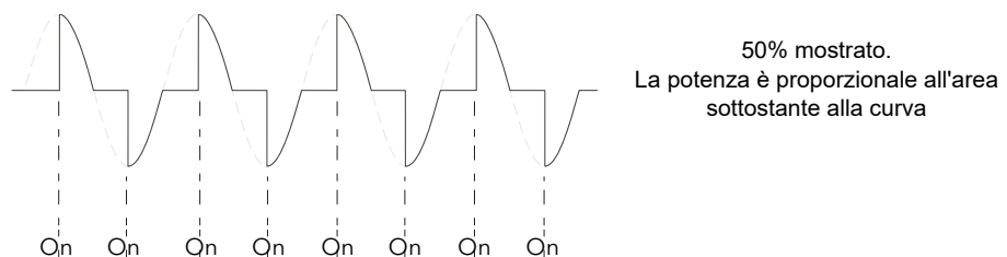
Figura 22 Accensione ad angolo di fase
