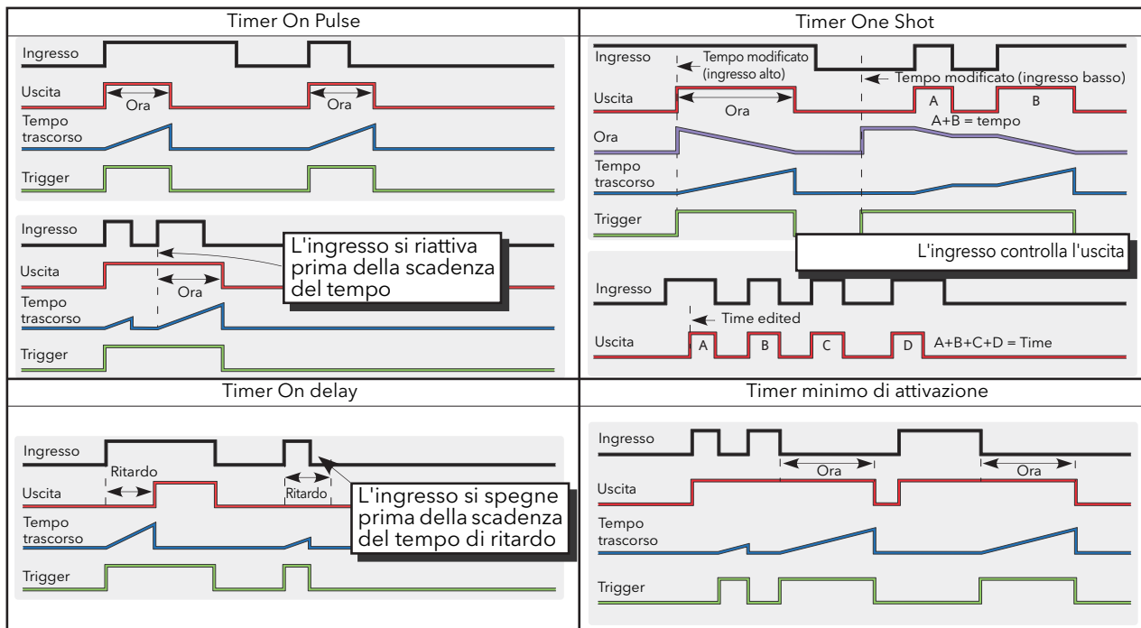
Figura 127 Esempi di timer
