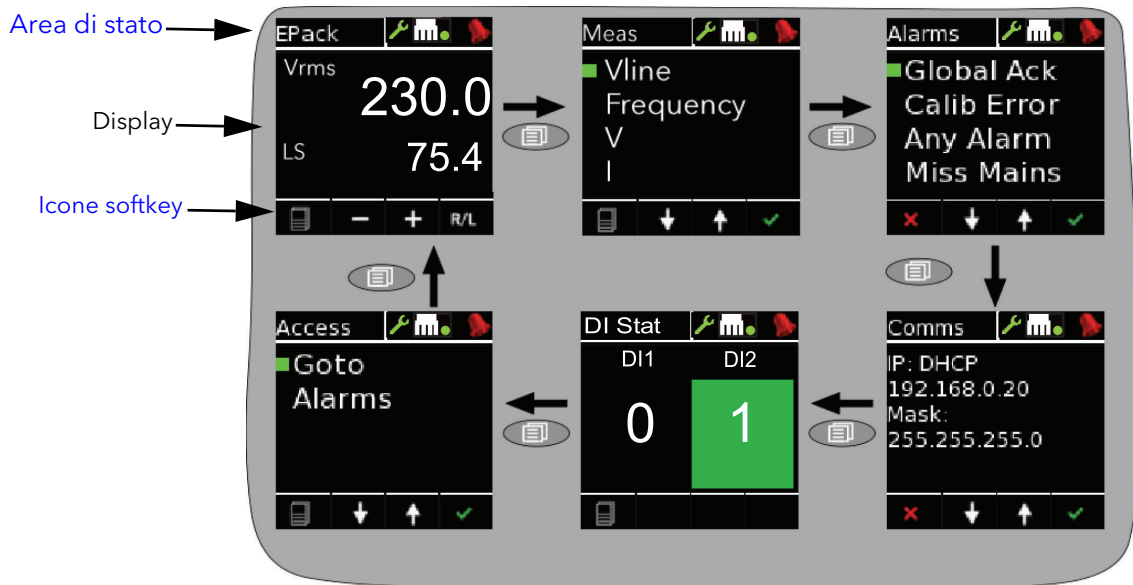
Figura 16 Interfaccia operatore
