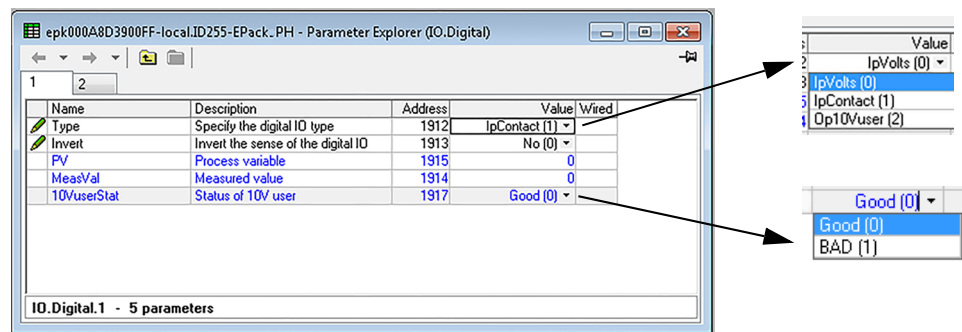
Figura 103 Pagina di configurazione degli ingressi digitali di iTools (ingresso digitale 2 visualizzato)
