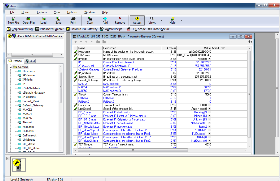
Figura 42 iTools - Parametro di comunicazione Ethernet
