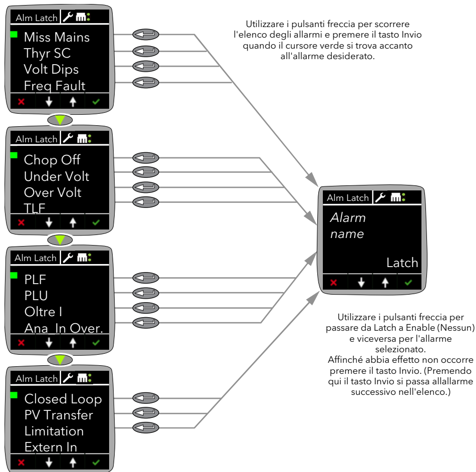
Figura 67 Menu Alarm Latch (Ritenuta allarme)
