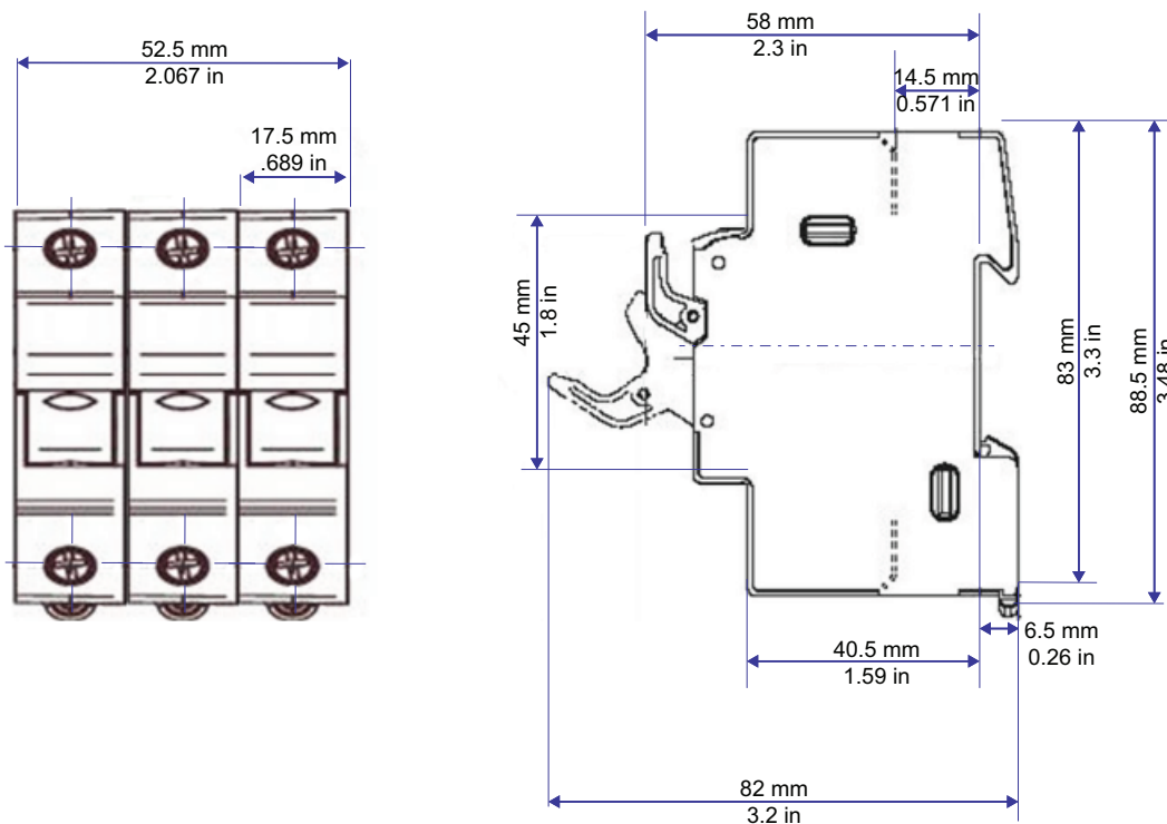
Figura 150 Dimensioni dei portafusibili: US103 (10x38 mm)
