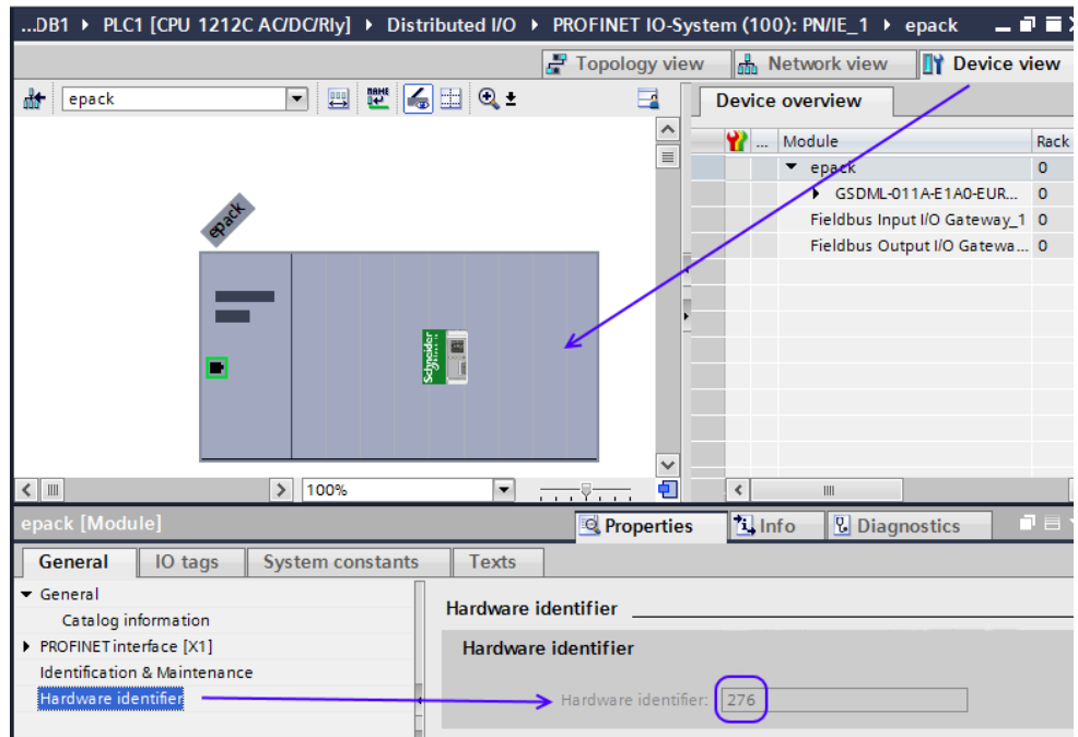
Figura 55 Valore identificativo hardware
