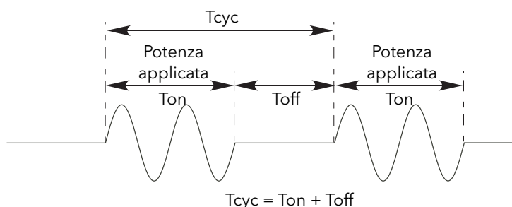
Figura 20 Modalità accensione fissa a treno di impulsi
