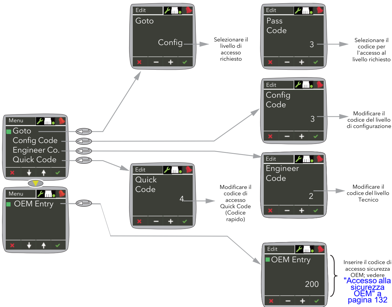
Figura 72 Menu Access (Accesso)
