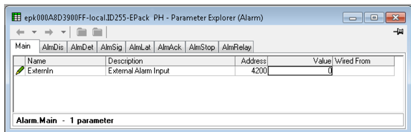
Figura 76 Configurazione degli allarmi
