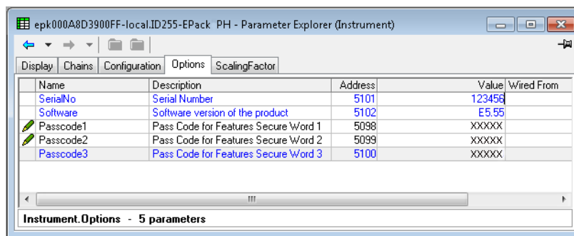
Figura 108 Pagina di configurazione dello strumento
