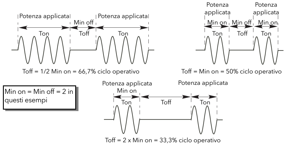
Figura 21 Accensione variabile a treno di impulsi
