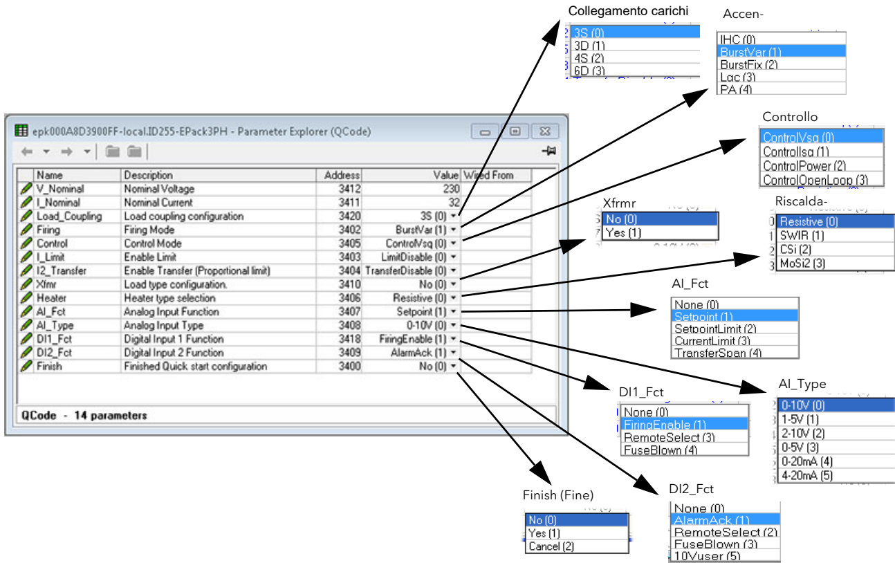
Figura 124 Parametri Quick Code
