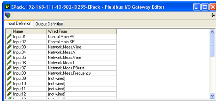
Figura 146 Tipico elenco di parametri di gateway fieldbus
