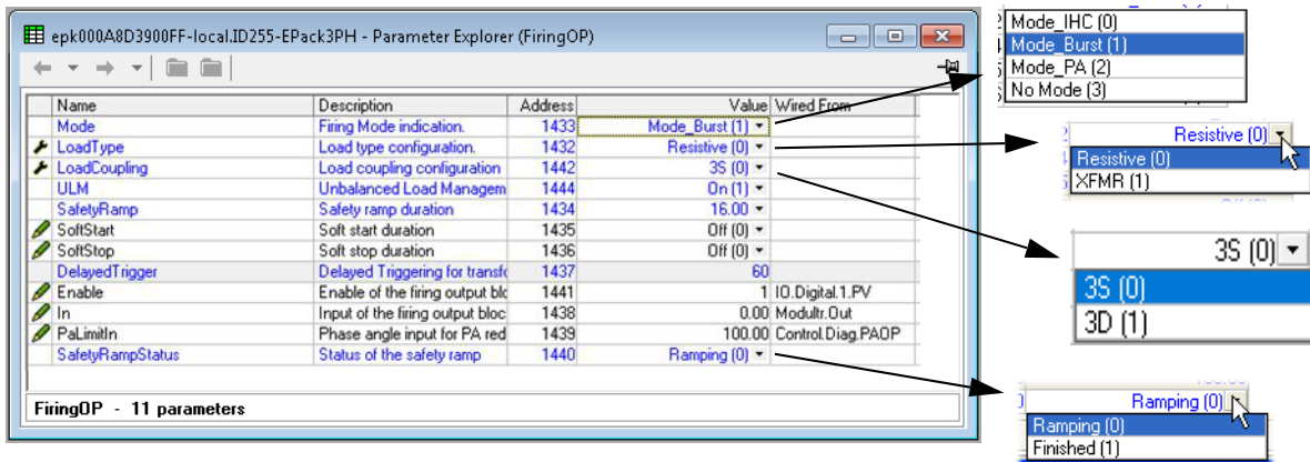
Figura 94 Pagina di configurazione dell'uscita di accensione di iTools
