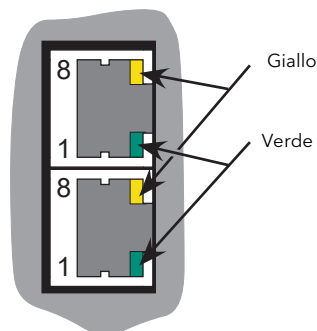
Figura 15 Morsettiere EPack
