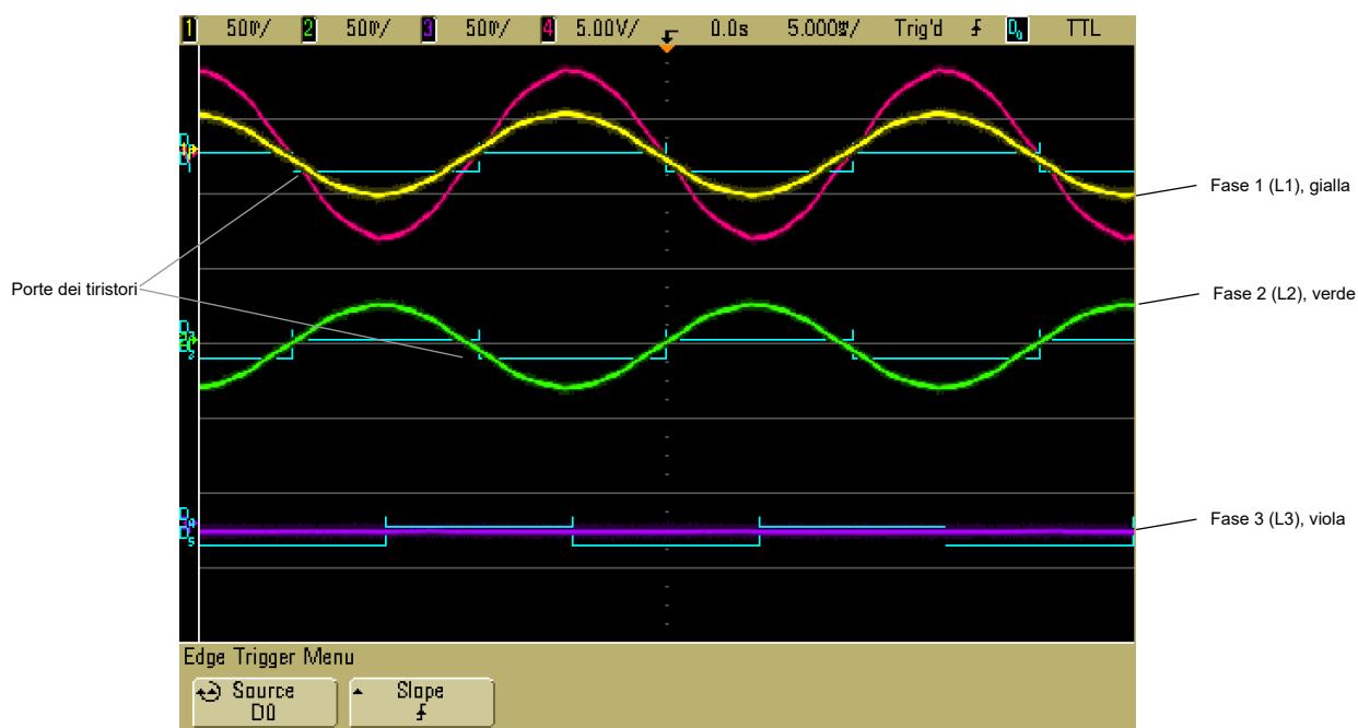
Figura 99 Forma d'onda, carico non bilanciato (circuitto aperto del carico L3), opzione ULM attiva, bilancia automaticamente le porte a tiristori e le rimanenti fasi 1 e 2
