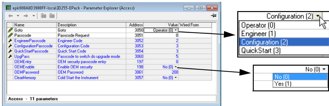
Figura 75 Menu di accesso iTools
