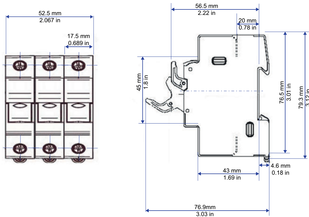
Figura 151 Dimensioni dei portafusibili: CUS103 (10x38 mm)
