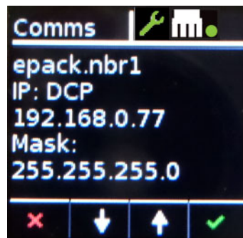
Figura 49 Visualizzazione del Nome dispositivo su Epack (ad es. "epack.nbr1")
