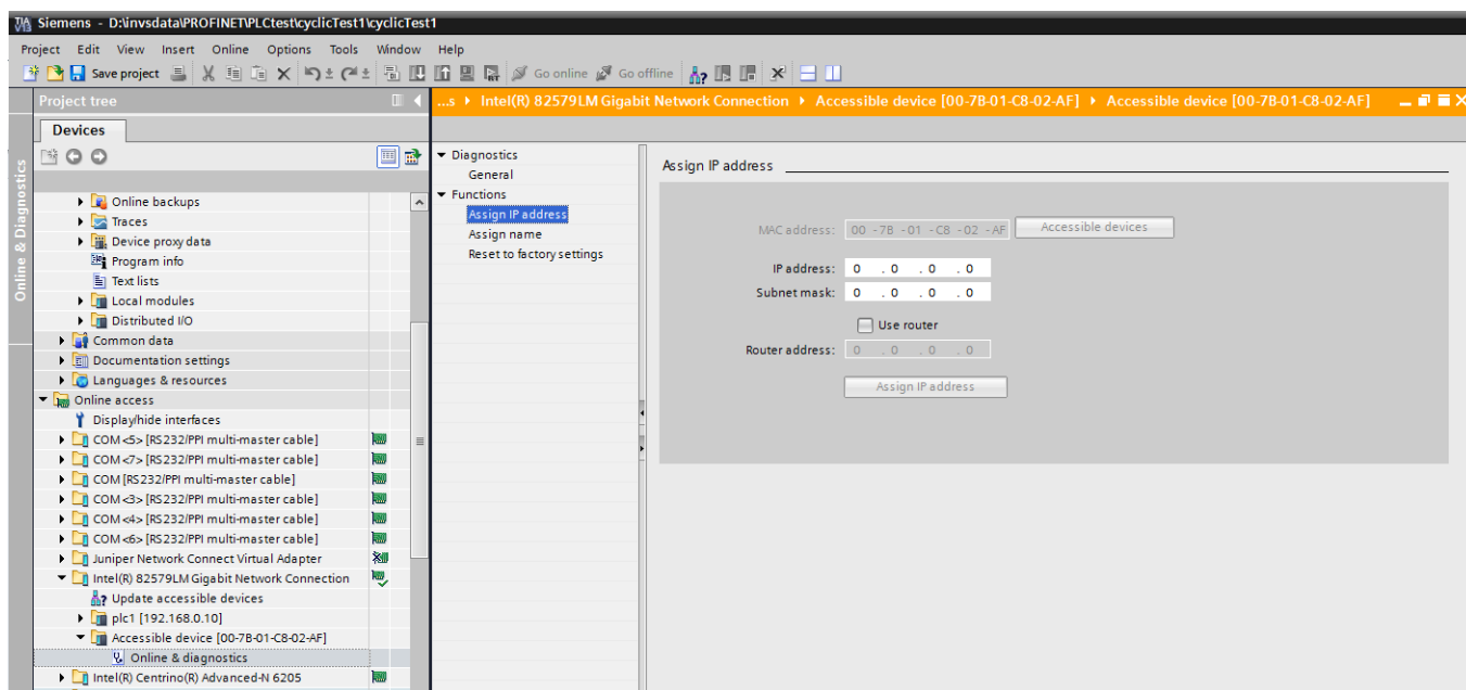
Figura 47 Assegnazione di configurazione IP e Nome dispositivo con "TIA Portal"
