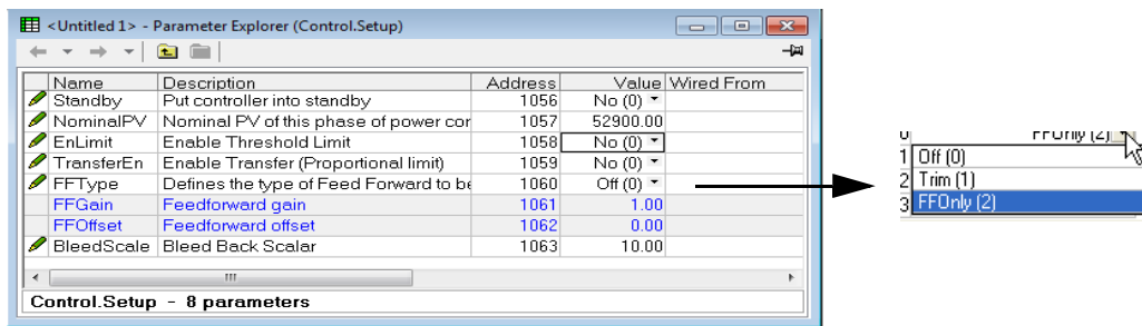
Figura 79 Pagina Control Setup (Configurazione controllo)
