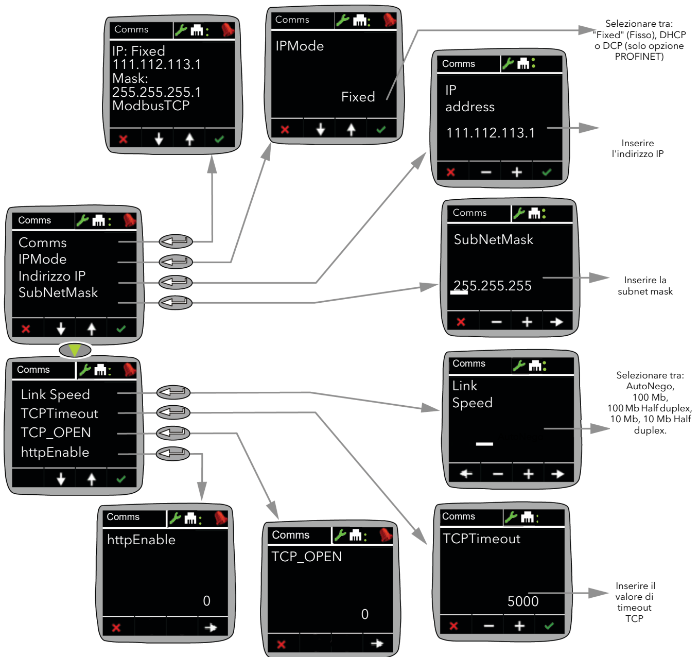
Figura 59 Menu Comms (Comunicazioni)
