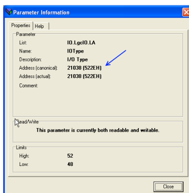
Figura 53 Accesso ai parametri tramite l'editor del cablaggio grafico.
