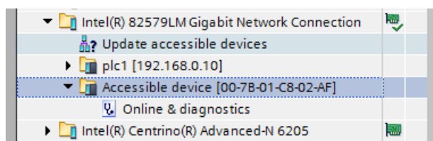
Figura 46 Esempio di indirizzo MAC di Epack (non ancora messo in servizio) che usa DCP
