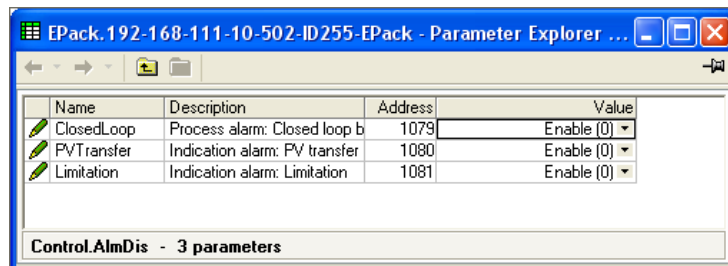
Figura 83 Pagina di disabilitazione dell'allarme
