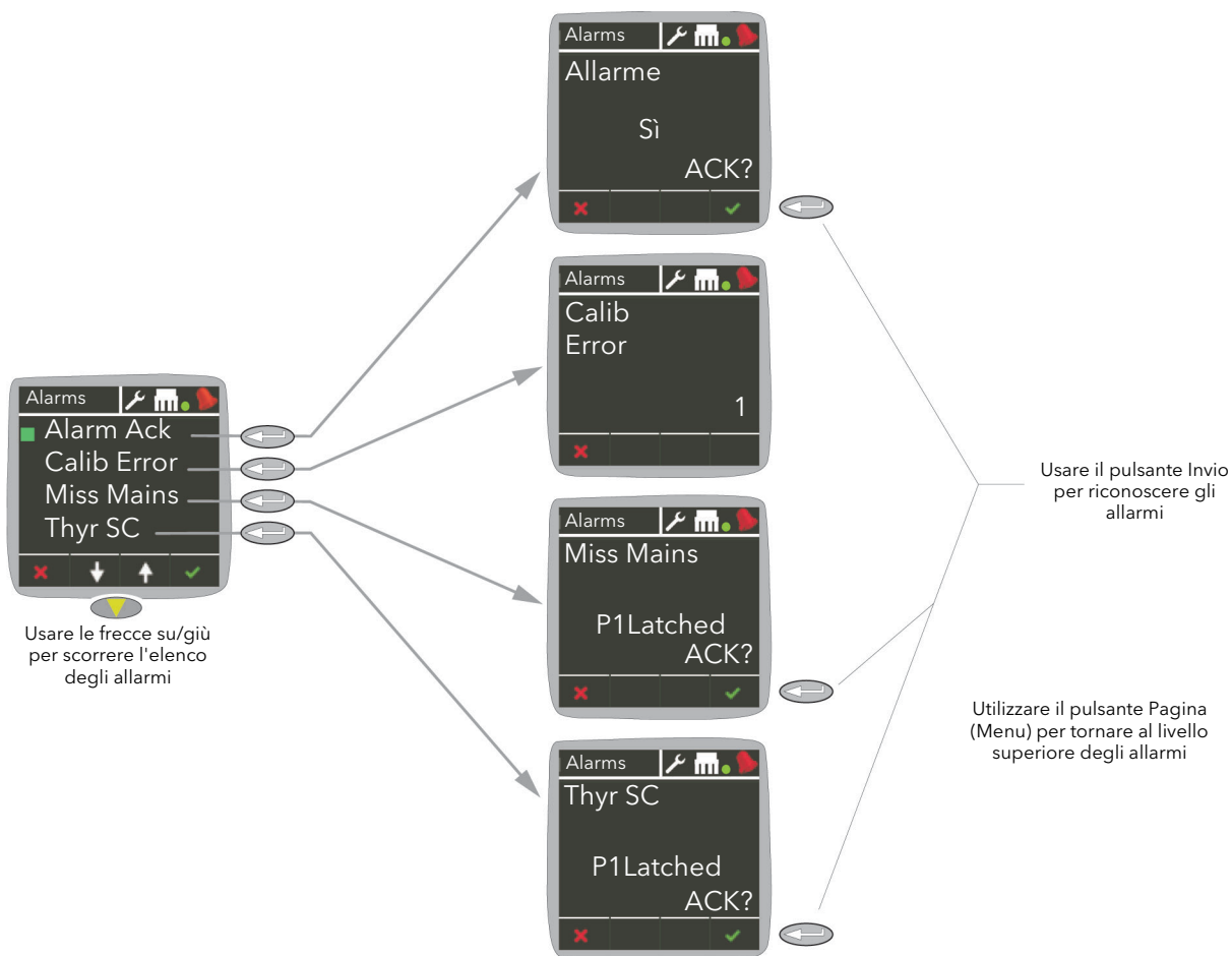
Figura 65 Menu Alarms (Allarmi)
