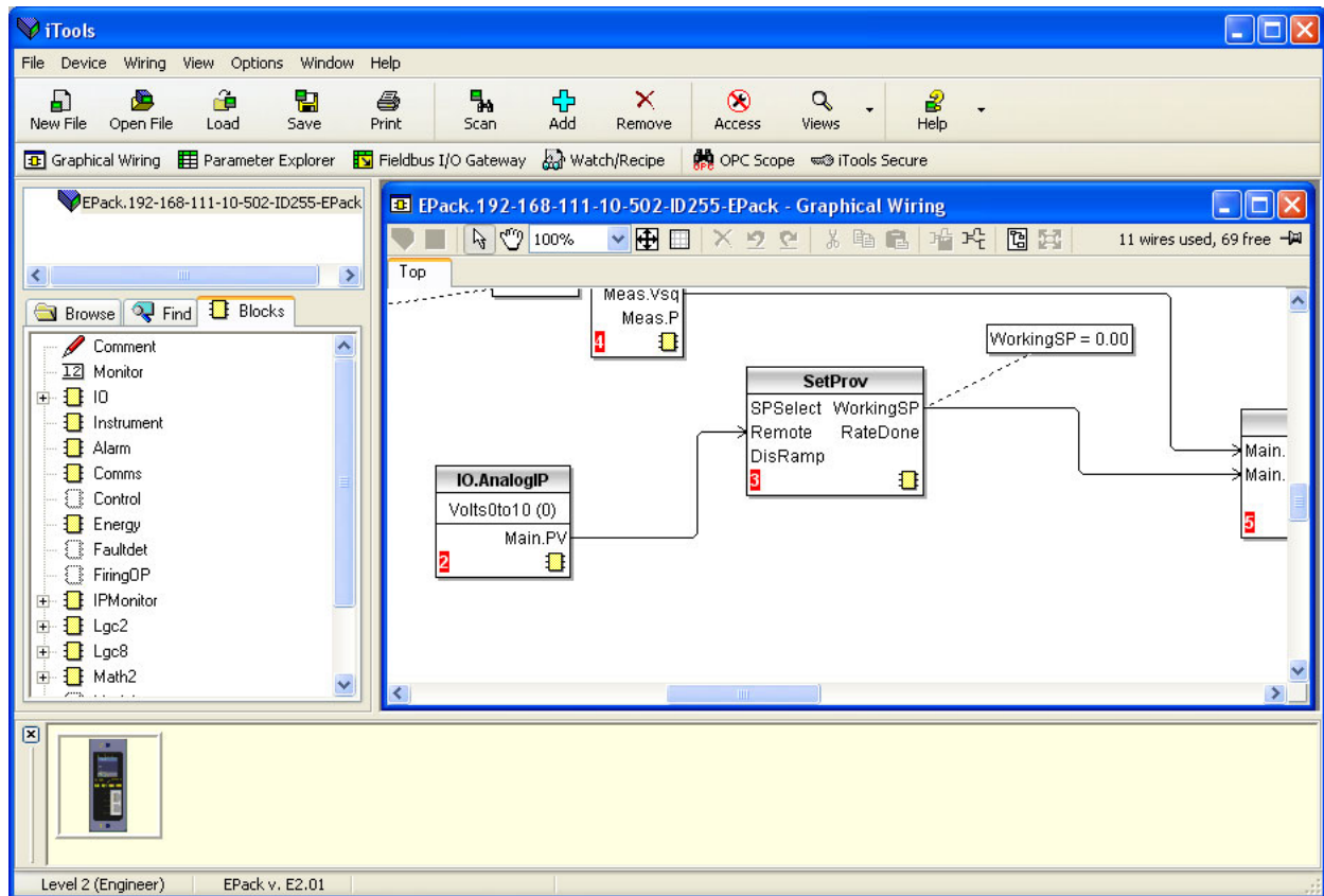
Figura 133 Editor del cablaggio grafico
