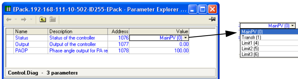
Figura 82 Menu di diagnostica iTools
