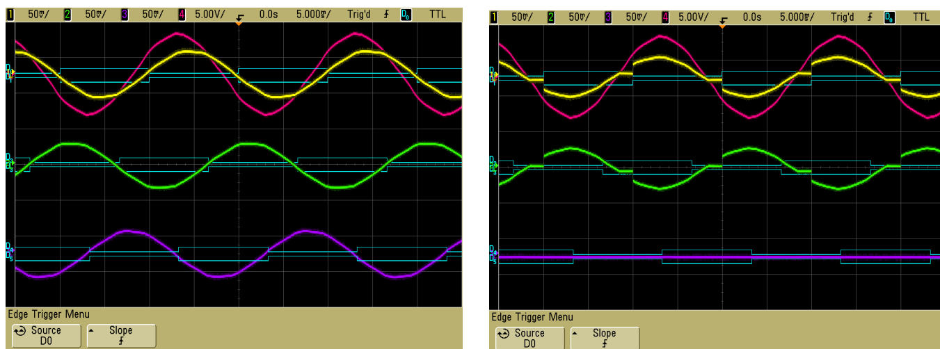
Figura 98 Forme d'onda; carico bilanciato a sinistra, carico non bilanciato a destra (ULM spento)
