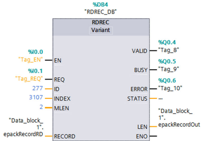
Figura 54 Lettura di un parametro di EPack tramite il blocco funzione RDREC di STEP 7
