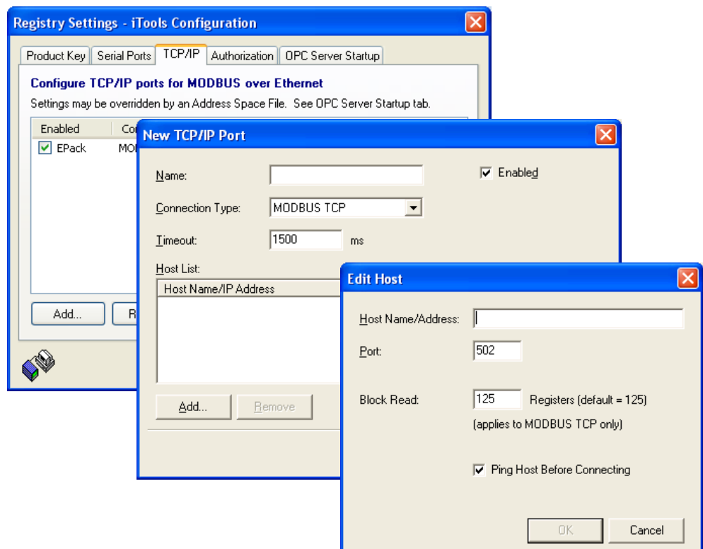
Figura 131 Aggiunta di una nuova porta Ethernet
