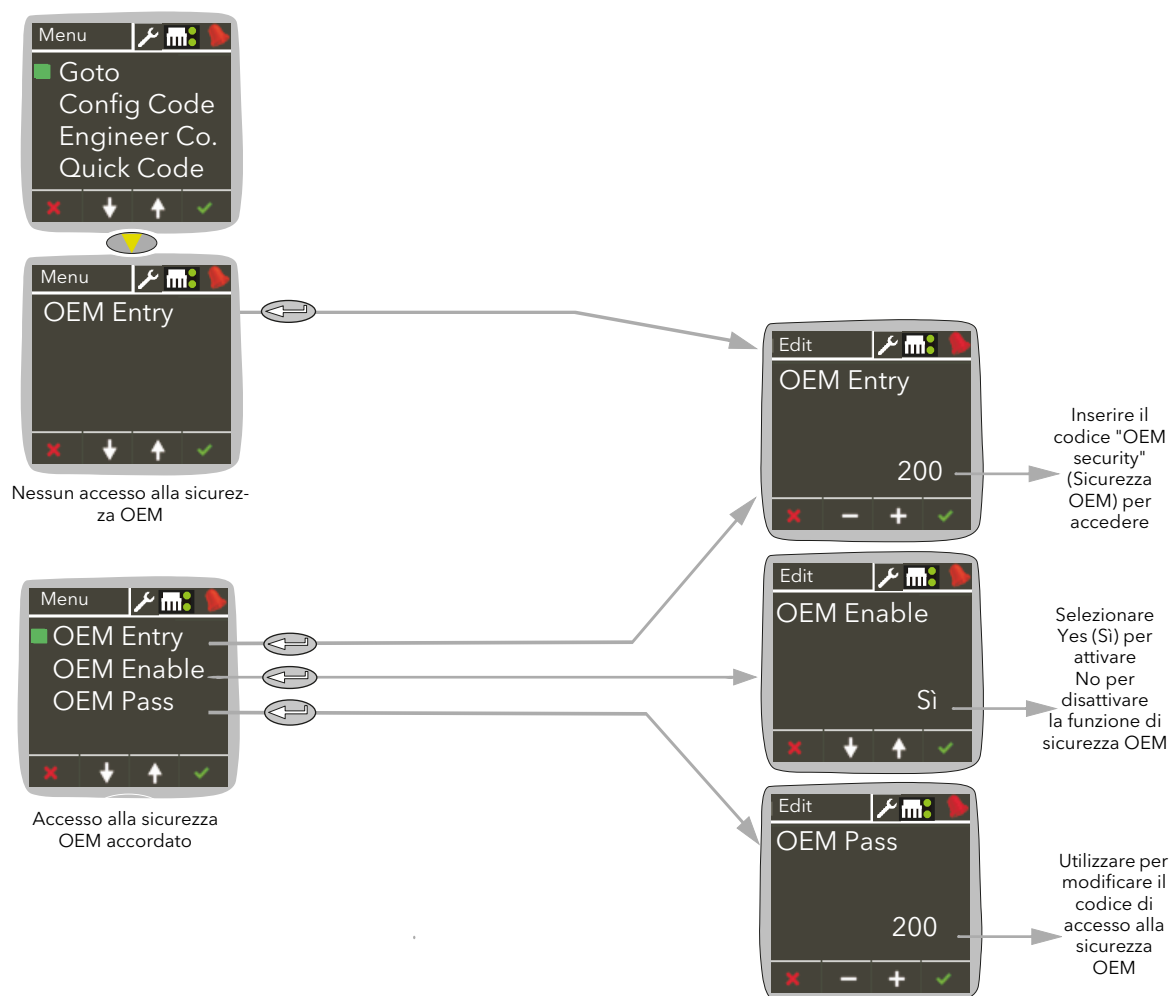
Figura 73 Accesso ai menu della sicurezza OEM
