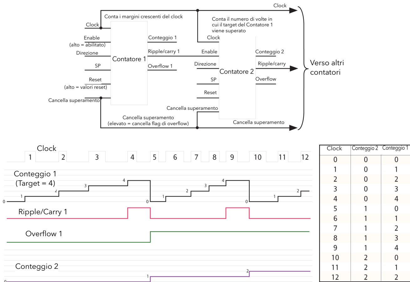
Figura 91 Contatori crescenti a cascata
