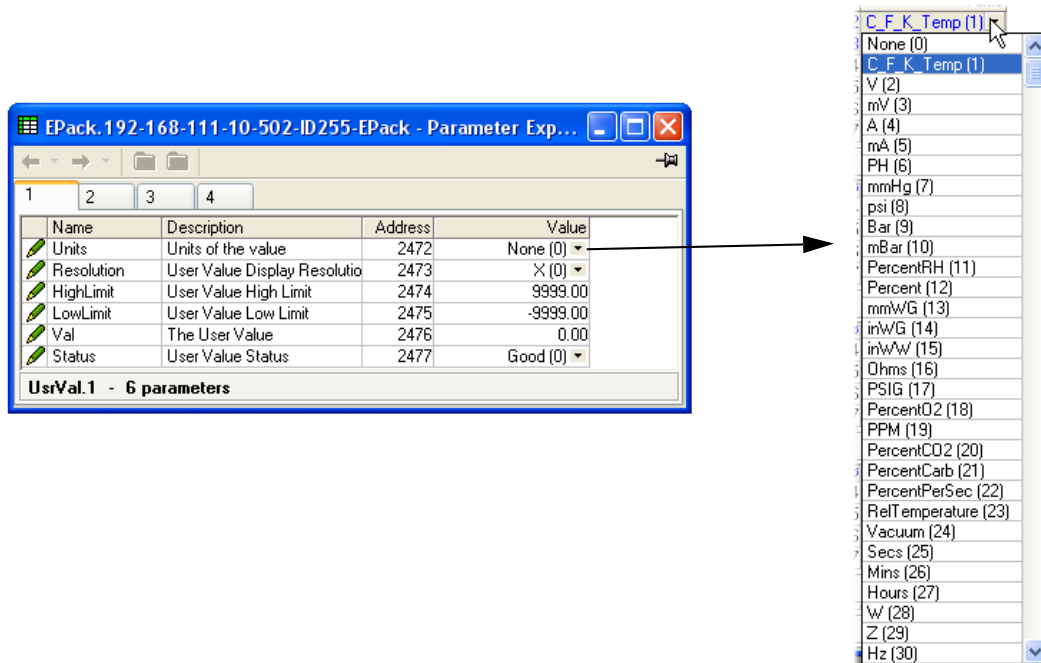
Figura 129 Pagina UseVal di livello superiore
