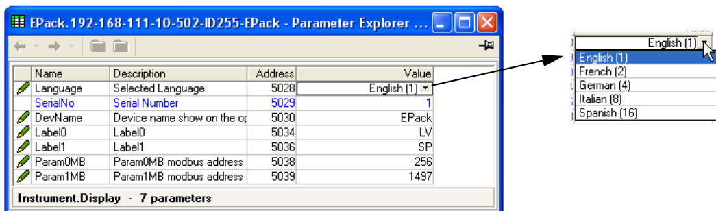
Figura 106 Pagina di configurazione del display strumento
