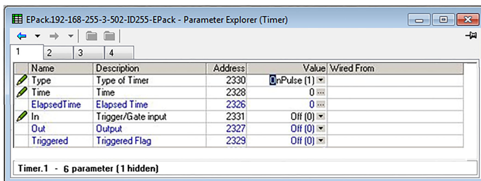
Figura 126 Configurazione del timer di iTools
