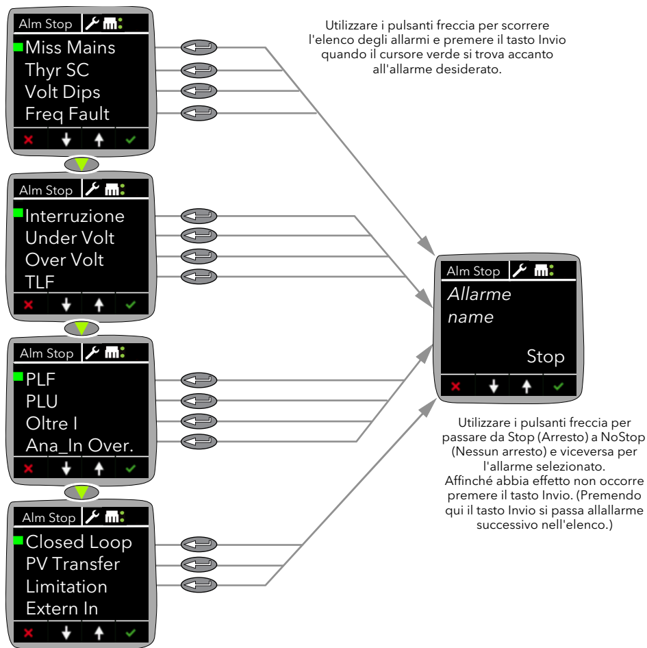
Figura 68 Menu Alarm Stop (Arresto allarme)
