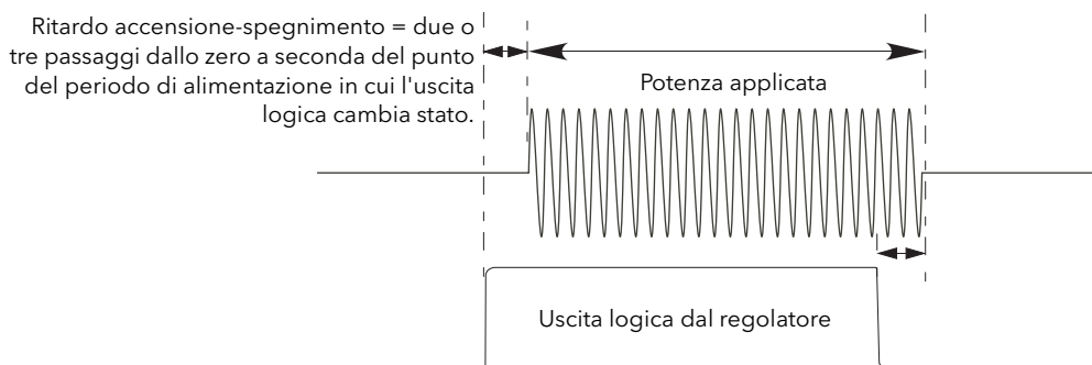
Figura 19 Modalità accensione logica
