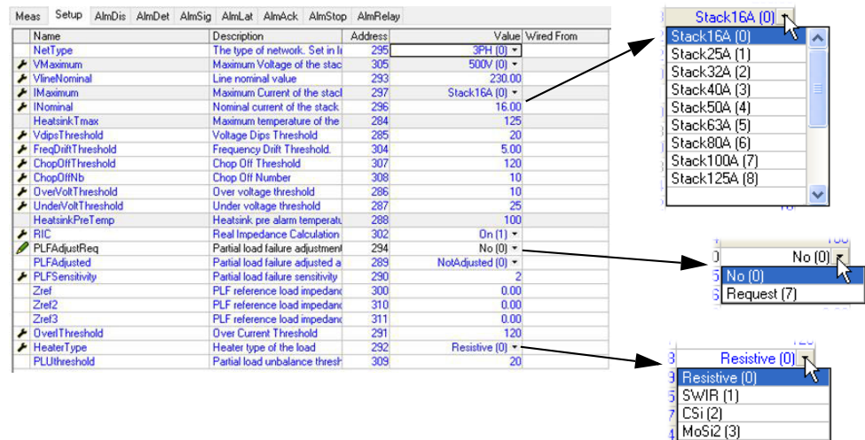
Figura 122 Pagina della configurazione di rete
