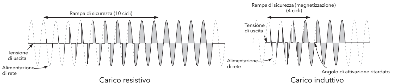
Figura 95 Esempi di rampa di sicurezza (accensione a treno di impulsi)
