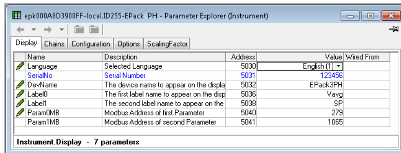
Figura 105 Menu di configurazione di livello superiore
