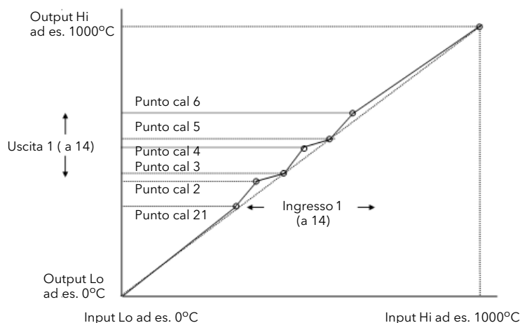
Figura 118 Compensazione in caso di discontinuità del sensore
