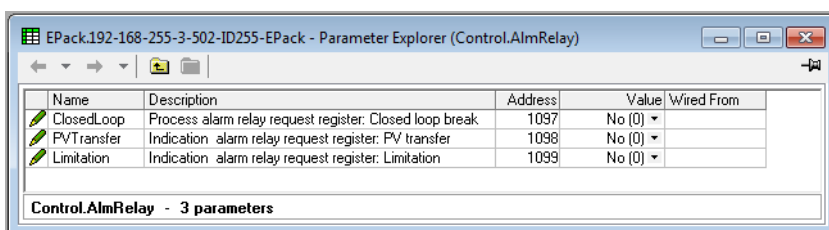
Figura 89 Pagina del relè dell'allarme di controllo di iTools
