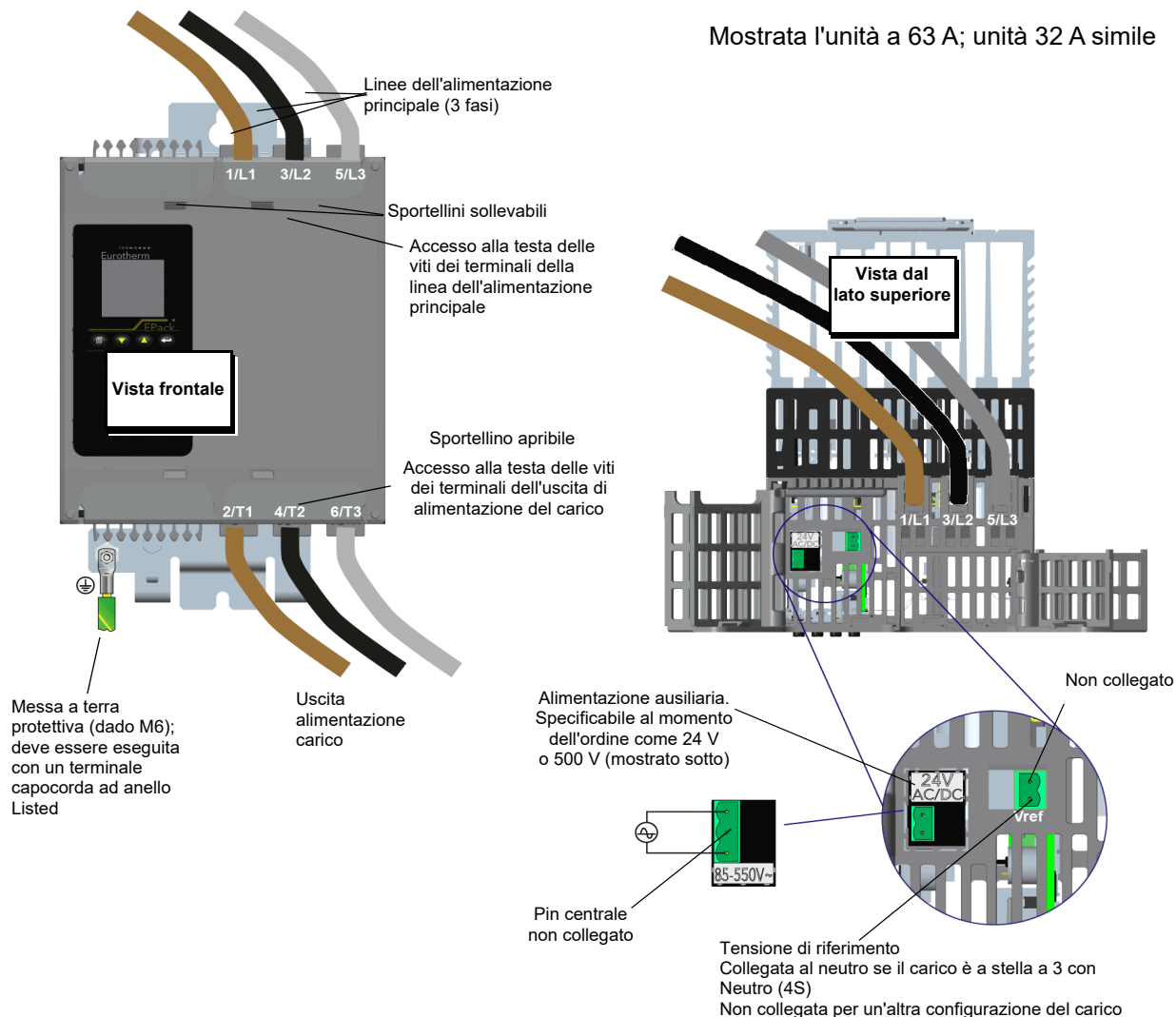
Figura 8 Dettagli su alimentazione e collegamento del carico (unità da 16 A a 63 A)
