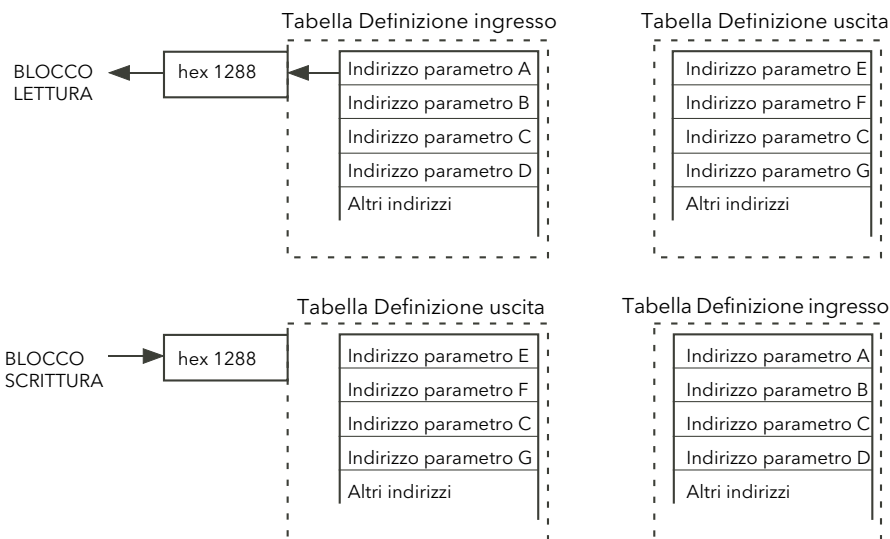
Figura 148 Blocco lettura e blocco scrittura (nota 3)
