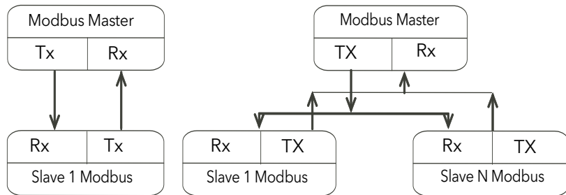
Figura 41 Collegamento seriale singolo e collegamento seriale multi-drop
