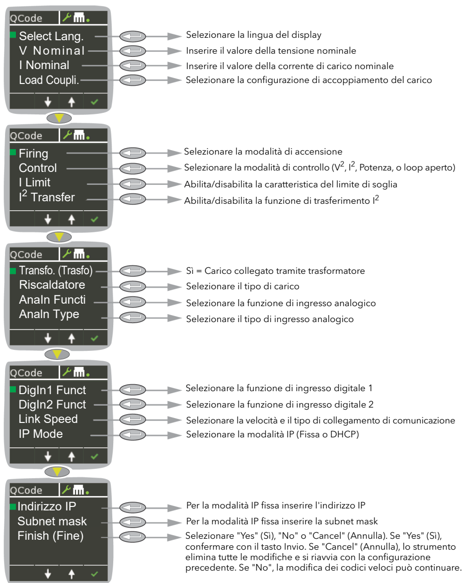
Figura 17 Menu Quick Code (Codice rapido) tipico
