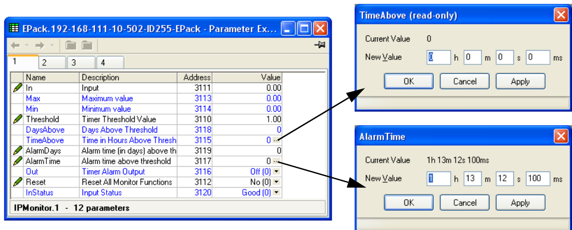
Figura 100 Pagina del monitor di ingresso di iTools (IPMon1)
