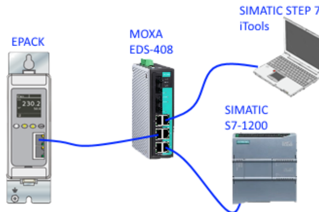
Figura 40 Collegamenti allo strumento di configurazione
