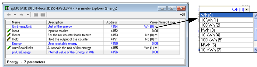
Figura 84 Pagina di configurazione dei consumi energetici
