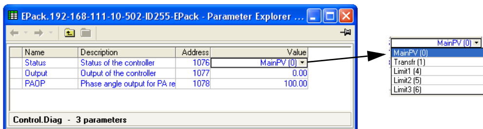
Figura 74 Menu di diagnostica iTools
