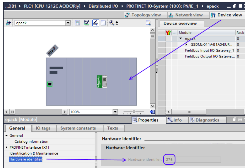
Figura 51 Valore identificativo hardware
