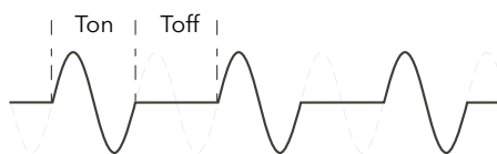
Figura 19 Modalità accensione a mezzo periodo intelligente: ciclo operativo al 50%
