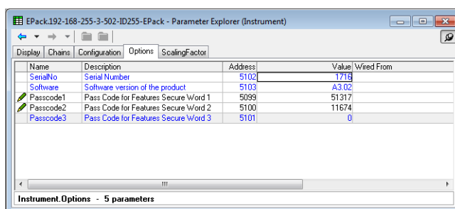
Figura 149 Configurazione opzioni strumento
