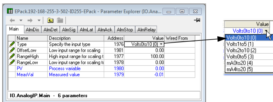
Figura 91 Pagina dell'ingresso analogico di iTools
