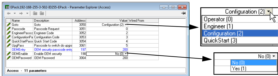
Figura 67 Menu di accesso iTools
