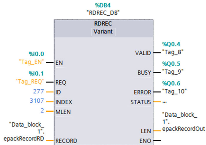
Figura 50 Lettura di un parametro di EPack tramite il blocco funzione RDREC di STEP 7
