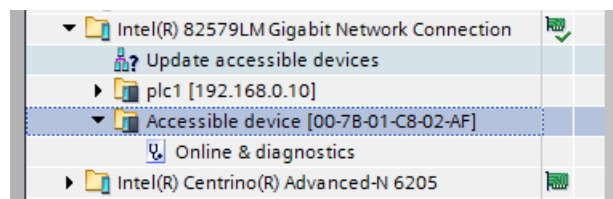
Figura 42 Esempio di indirizzo MAC di Epack (non ancora messo in servizio) che usa DCP
