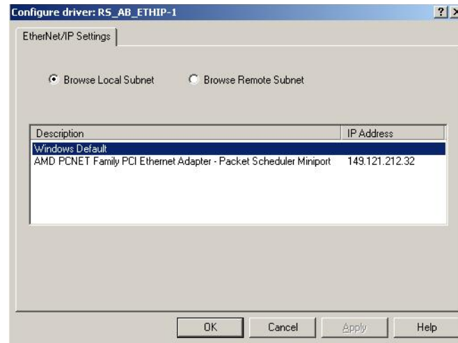
Figura 35 Impostazioni Ethernet/IP di configurazione del driver di RSLinx Classic Adesso è possibile navigare all'interno della rete e individuare EPack.
