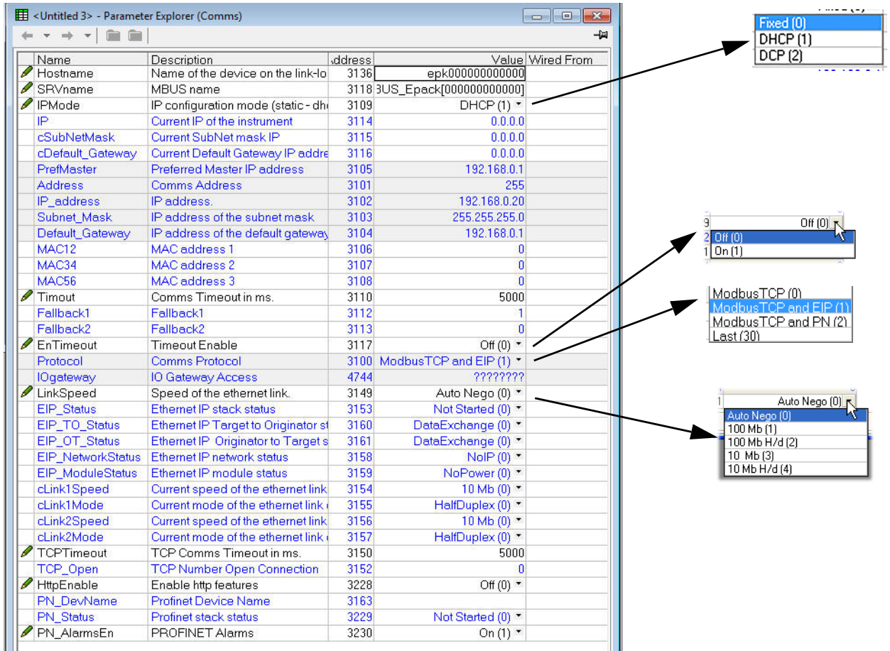
Figura 69 Pagina Comms (Comunicazioni) di iTools
