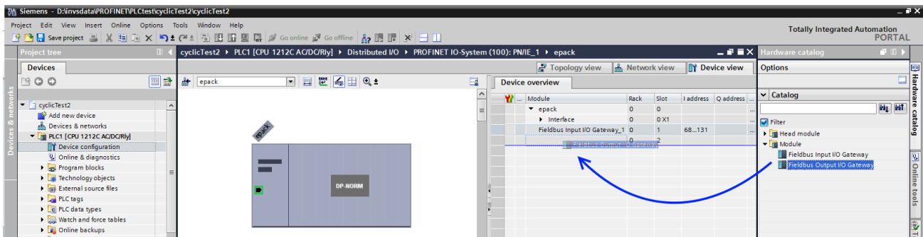
Figura 47 "Drag and Drop" dei moduli I/O
