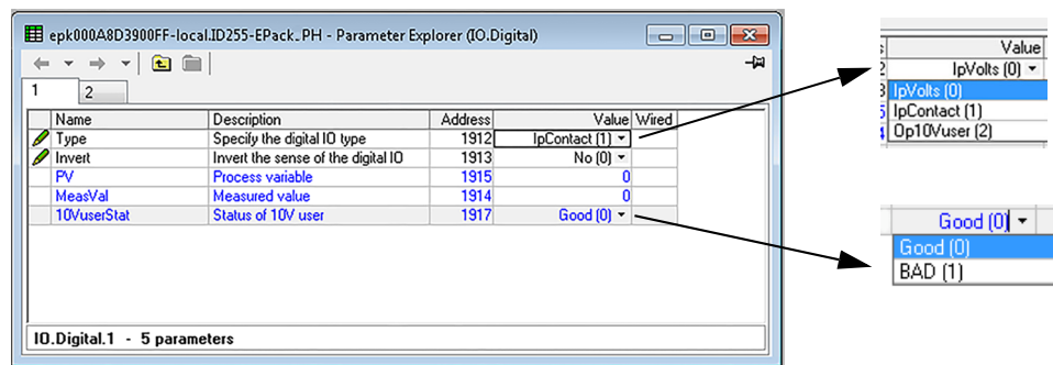
Figura 93 Pagina di configurazione degli ingressi digitali di iTools (ingresso digitale 2 visualizzato)
