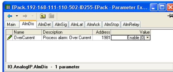
Figura 92 Esempio di AlmDis
