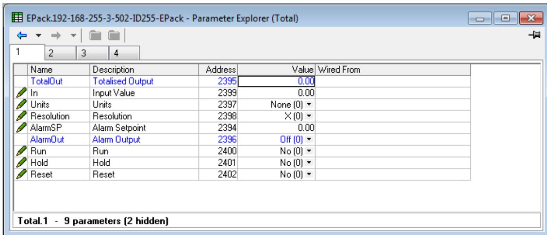
Figura 118 Pagina del totalizzatore di iTools
