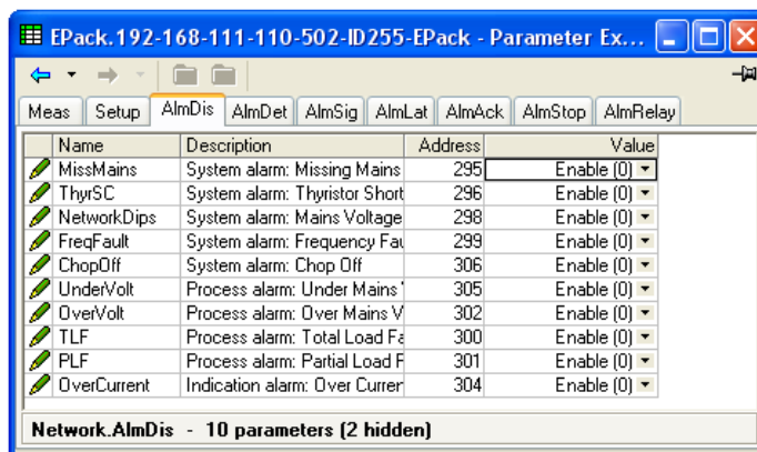
Figura 113 Pagina degli allarmi di rete
