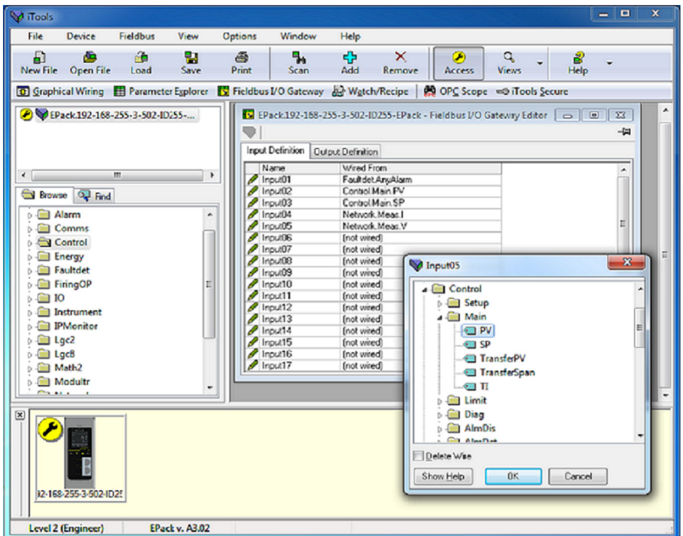
Figura 24 Selezione di un valore di ingresso ed esempio di un elenco ingresso
