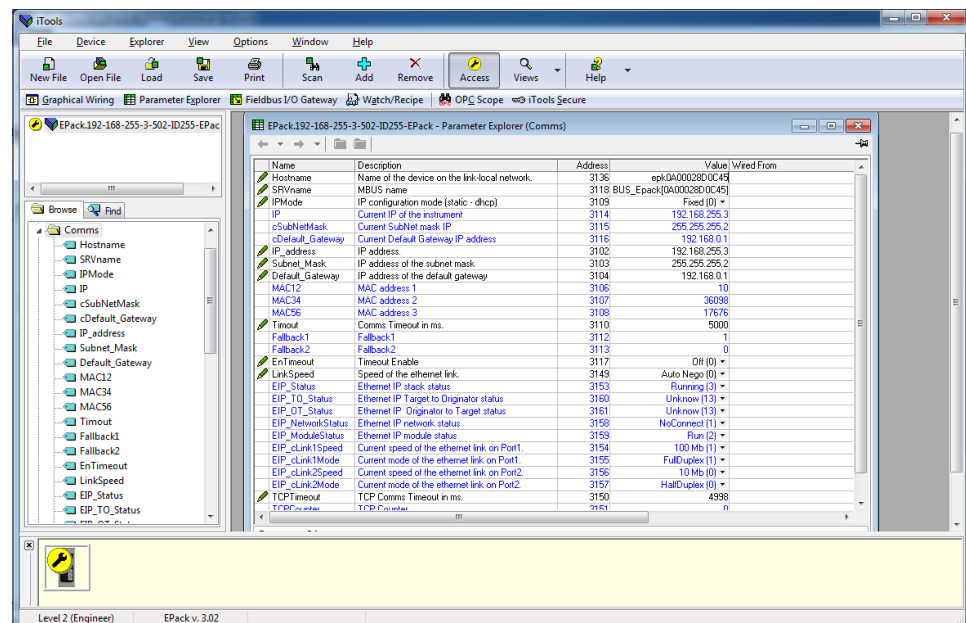
Figura 38 iTools - Parametro di comunicazione Ethernet
