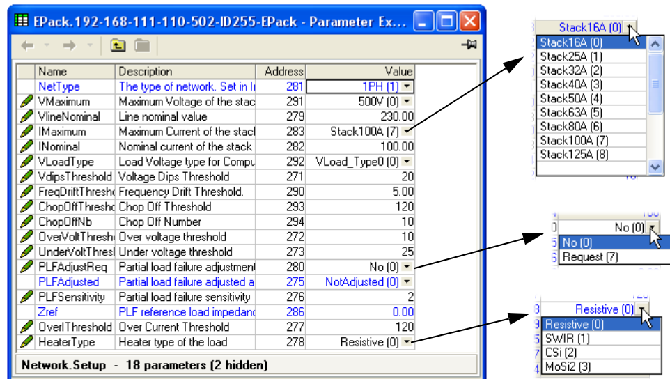
Figura 112 Pagina della configurazione di rete
