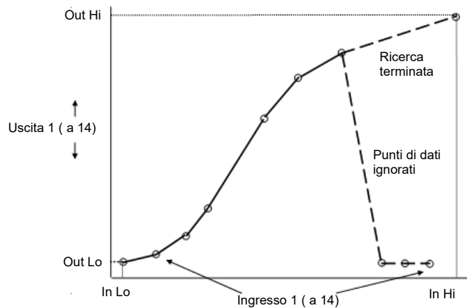
Figura 106 Esempio di linearizzazione
