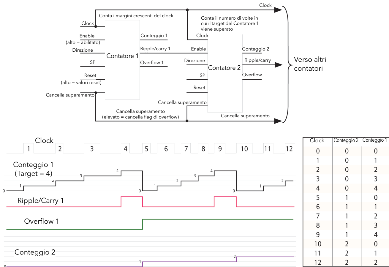
Figura 83 Contatori crescenti a cascata
