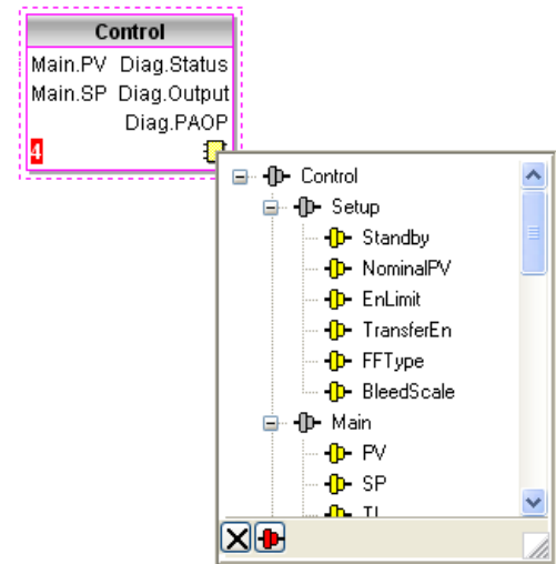
Figura 129 Finestra di dialogo di selezione dell'uscita
