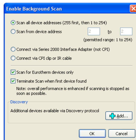
Figura 124 Abilitazione dell'intervallo di scansione
