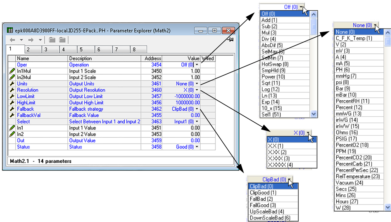
Figura 109 Pagina di configurazione delle funzioni matematiche 2
