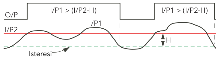
Figura 102 Isteresi
