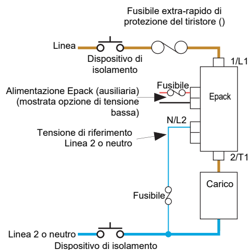
Figura 8 Dettagli su alimentazione e collegamento del carico (unità da 16 A a 63 A)
