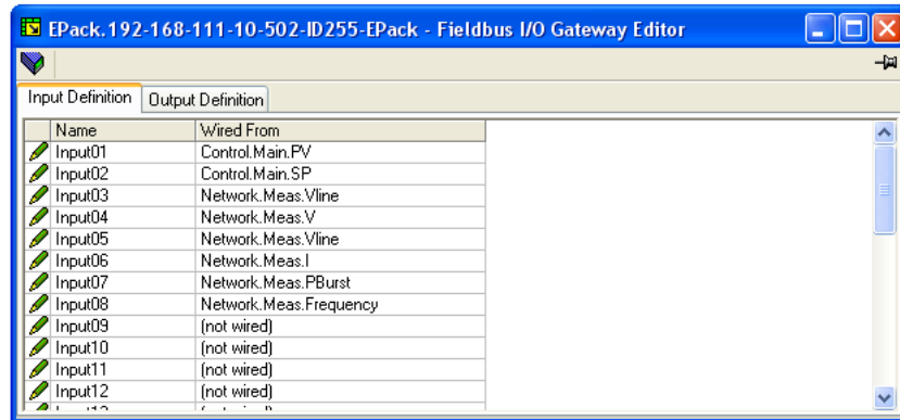
Figura 139 Tipico elenco di parametri di gateway fieldbus
