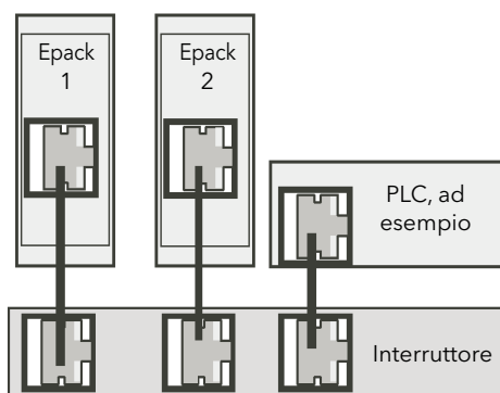
Figura 39 CABLAGGIO PROFINET - Regolatori multipli
