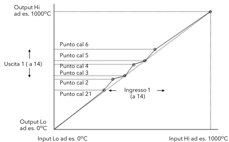
Figura 108 Compensazione in caso di discontinuità del sensore
