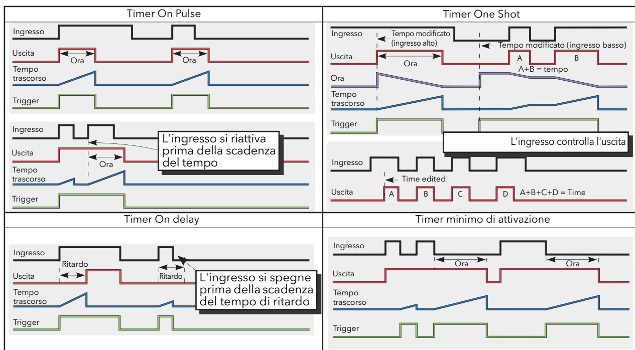
Figura 117 Esempi di timer
