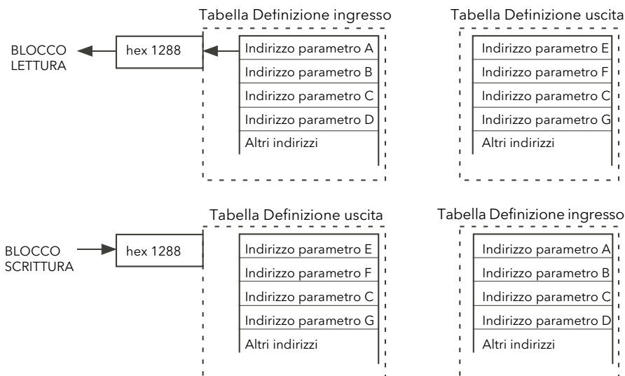
Figura 141 Blocco lettura e blocco scrittura (nota 3)
