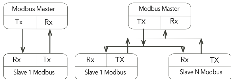
Figura 37 Collegamento seriale singolo e collegamento seriale multi-drop
