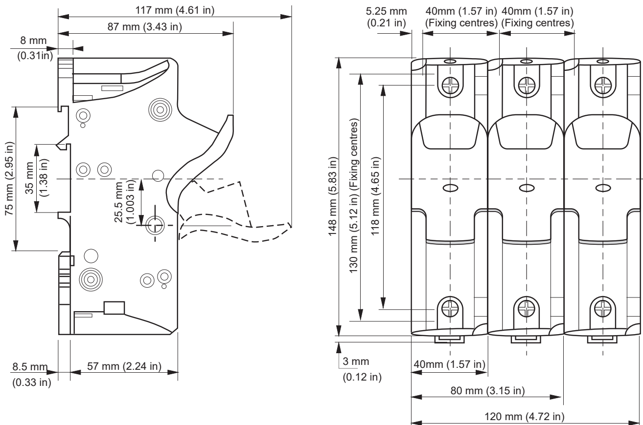
Figura 146 Dimensioni dei portafusibili: US271 (27x60 mm)
