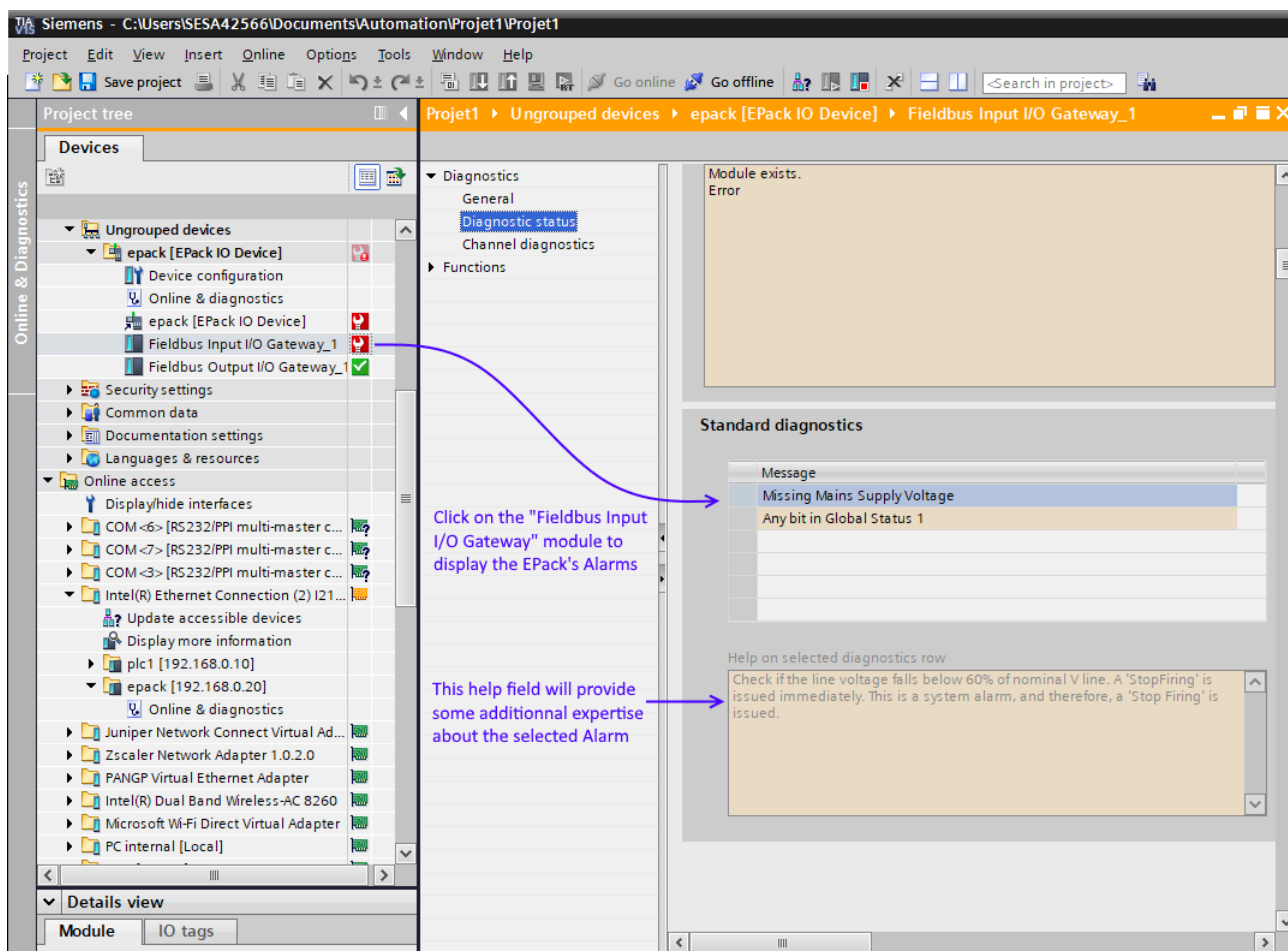
Figura 52 Screenshot di TIA Portal che mostra una rappresentazione degli allarmi EPack
