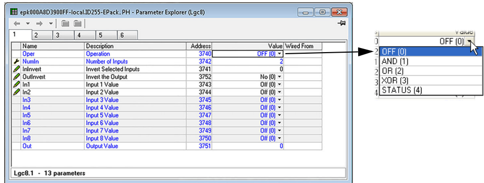
Figura 104 Pagina di configurazione Lgc8
