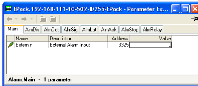
Figura 68 Configurazione degli allarmi
