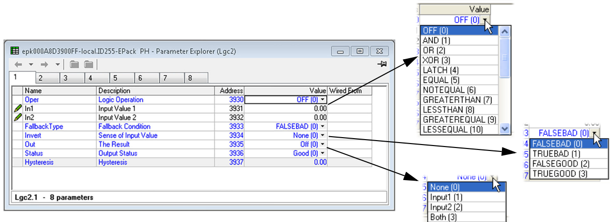
Figura 101 Pagina Lgc2 (Lgc2 1)
