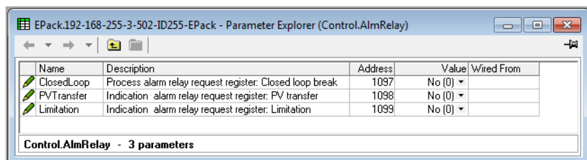
Figura 81 Pagina del relè dell'allarme di controllo di iTools
