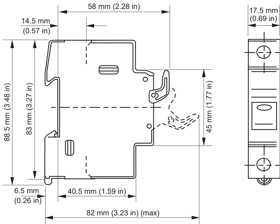
Figura 143 Dimensioni dei portafusibili: US101 (10x38 mm)
