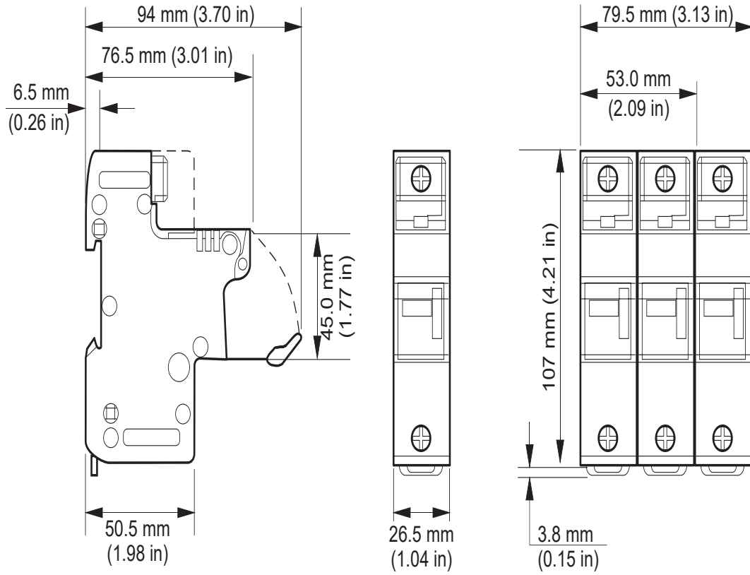
Figura 145 Dimensioni dei portafusibili: US141 (14x51 mm)
