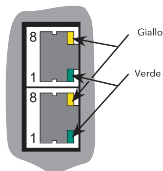
Figura 11 Morsettiere EPack
