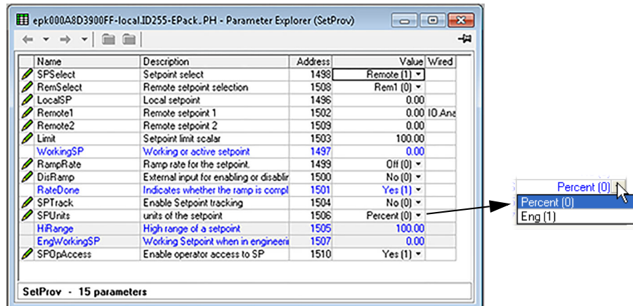
Figura 115 Pagina di configurazione SetProv
