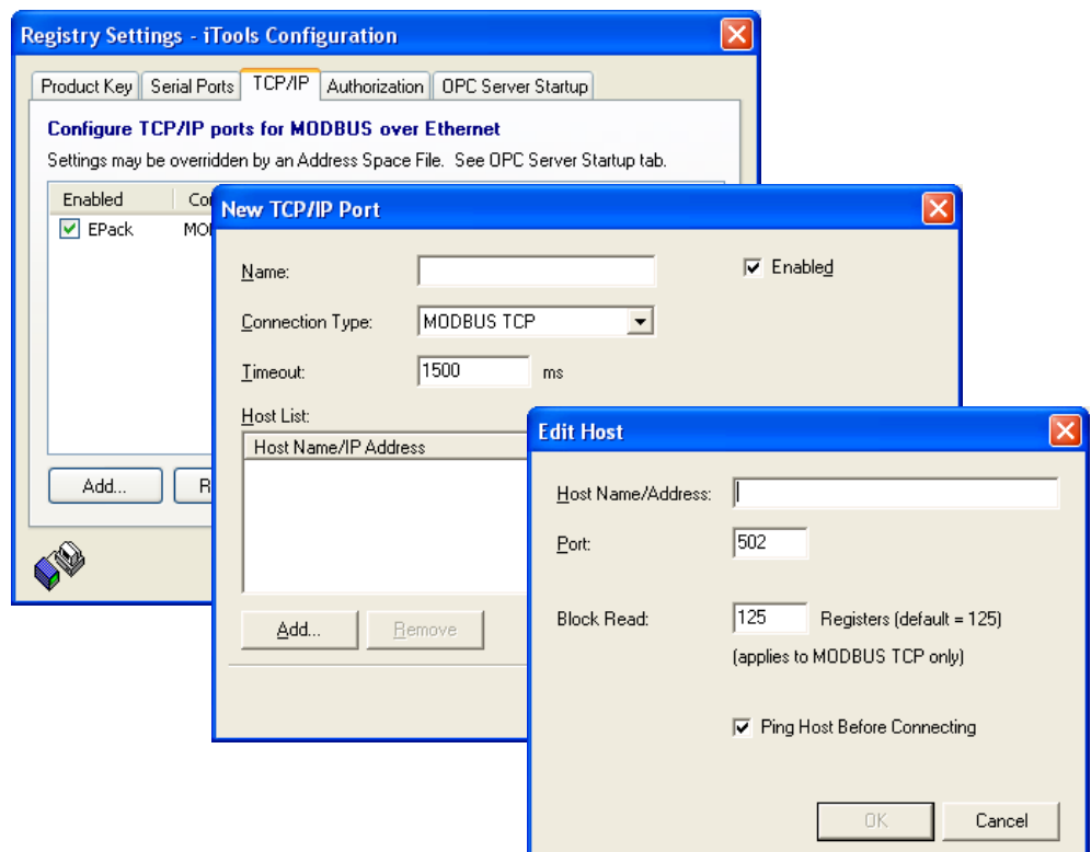
Figura 121 Aggiunta di una nuova porta Ethernet
