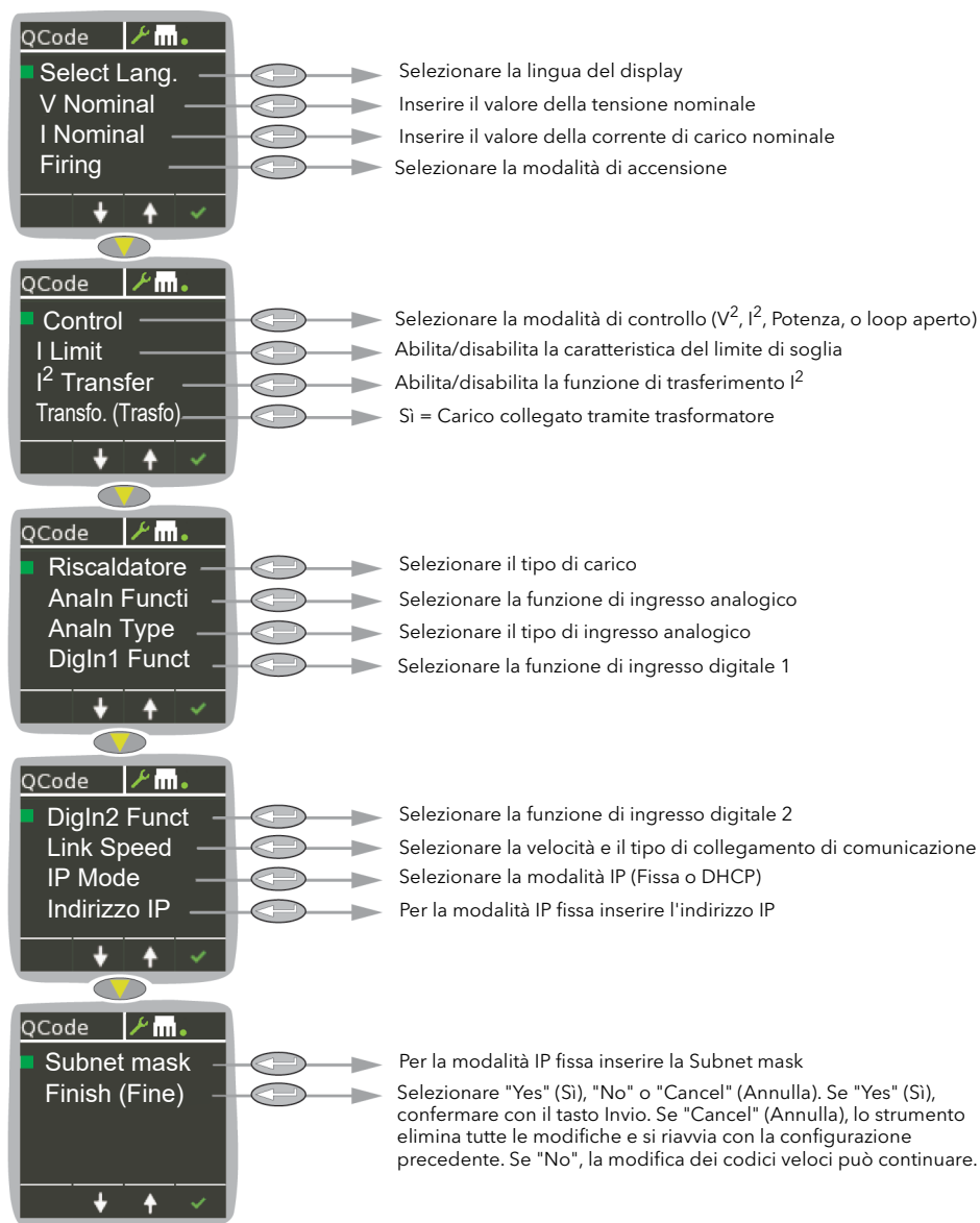
Figura 13 Menu Quick Code (Codice rapido) tipico
