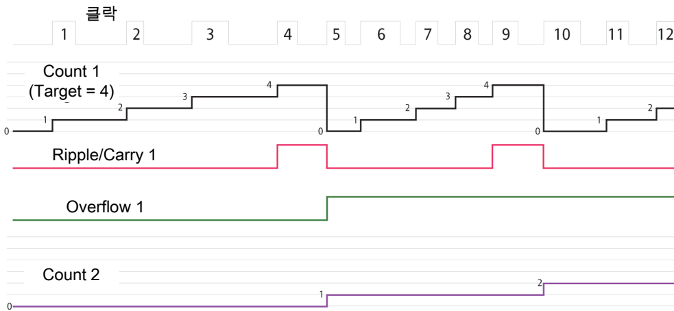
그림 85 연쇄 업카운터
