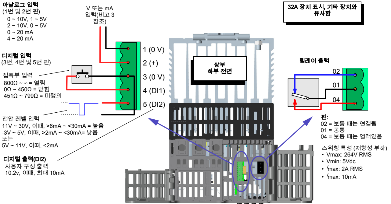
그림 12 I/O 세부 사항
