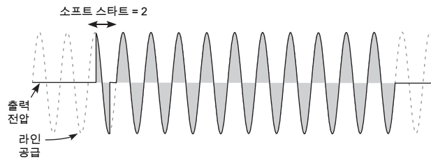
그림 90 소프트 스타트 예시
