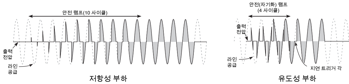
그림 89 안전 램프(버스트 점호) 예시
