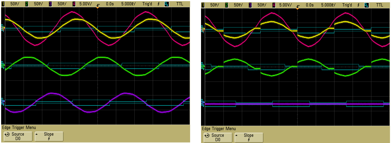
그림 92 파형: 왼쪽 균형 부하 및 오른쪽 불균형 부하(ULM 꺼짐)
