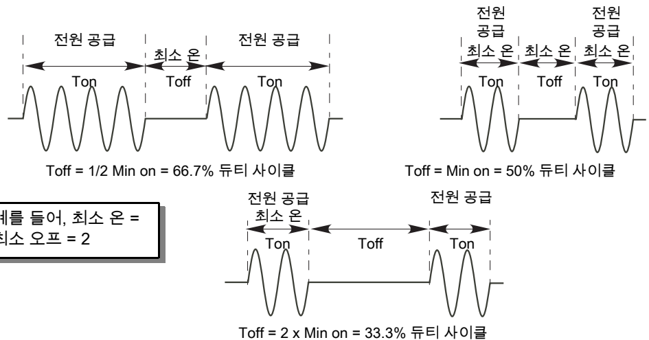
그림 19 버스트 가변 점호
