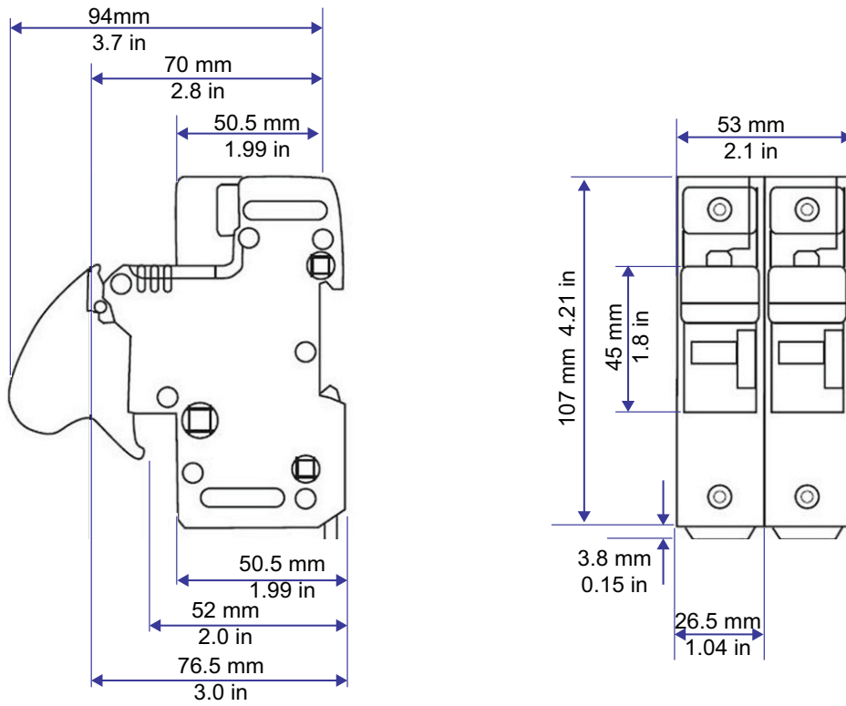
그림 146 퓨즈 홀더 치수: US142 (14x51mm)
