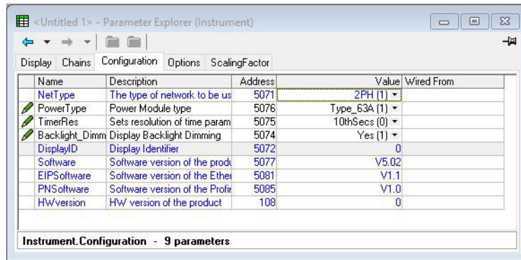
그림 101 기기 구성
