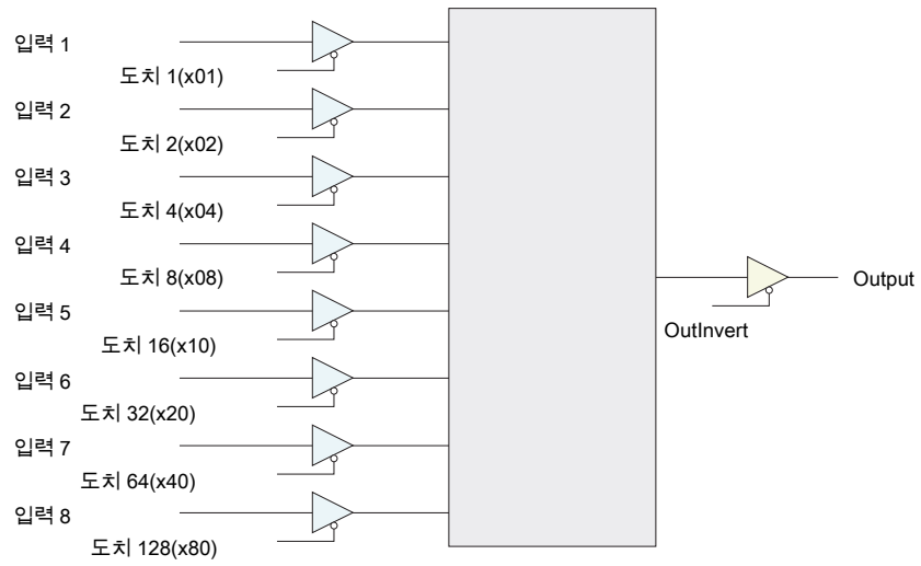
그림 109 LGC8 도해
