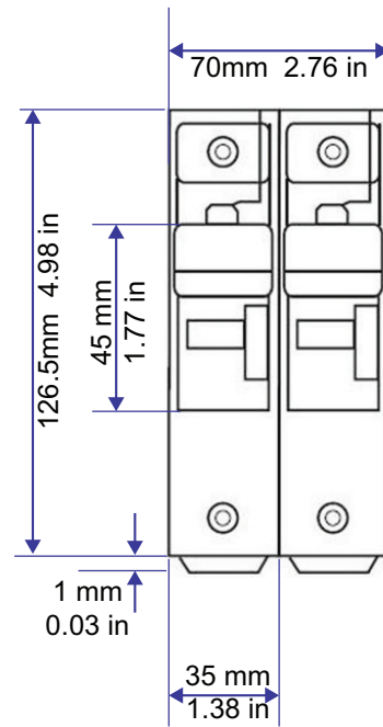
그림 147 퓨즈 홀더 치수: US222 (22x58mm)
