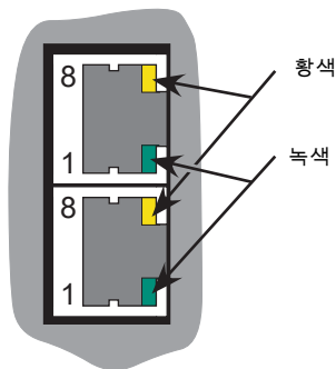
그림 13 EPack 핀 배치
