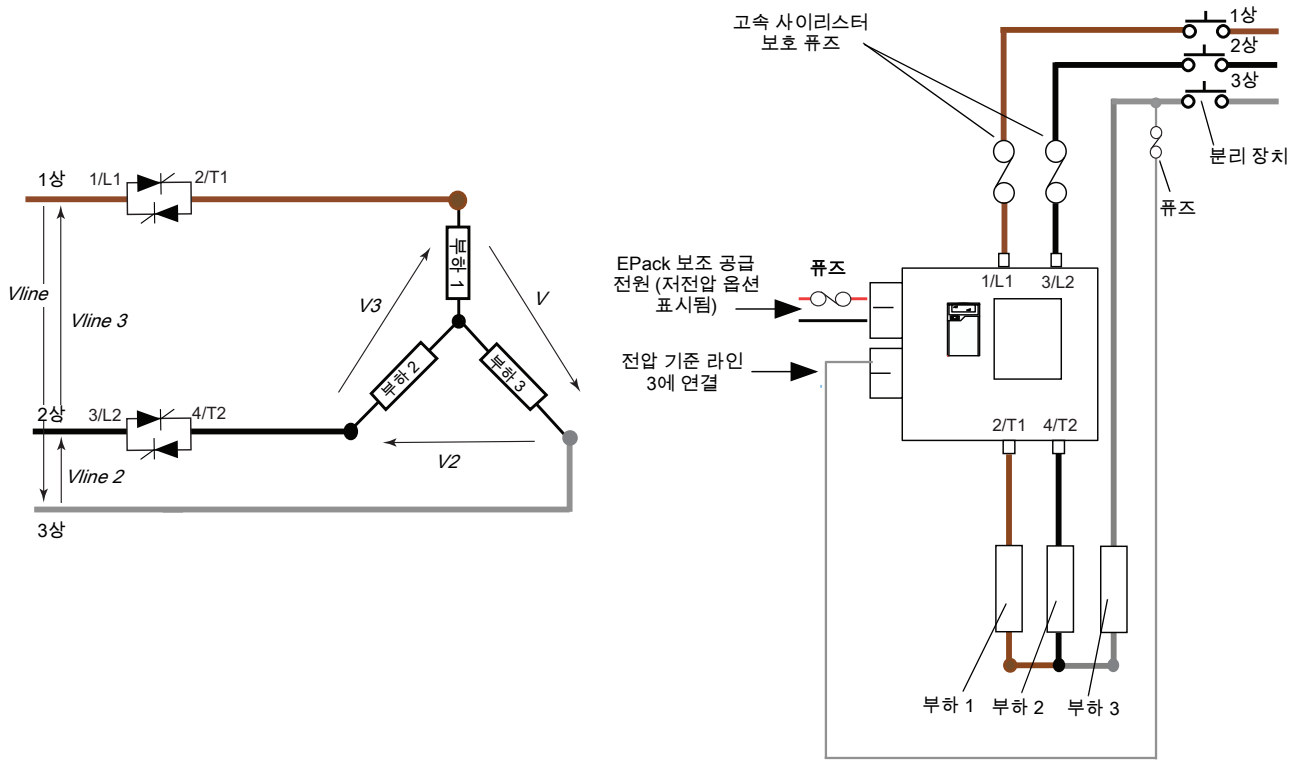
그림 11 2 phase 비중성 별 배선 도해/부하 구성
