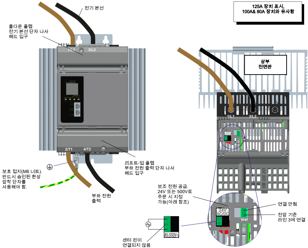
그림 9 공급 전원 및 부하 연결 세부 사항(80A ~ 125A 장치).
