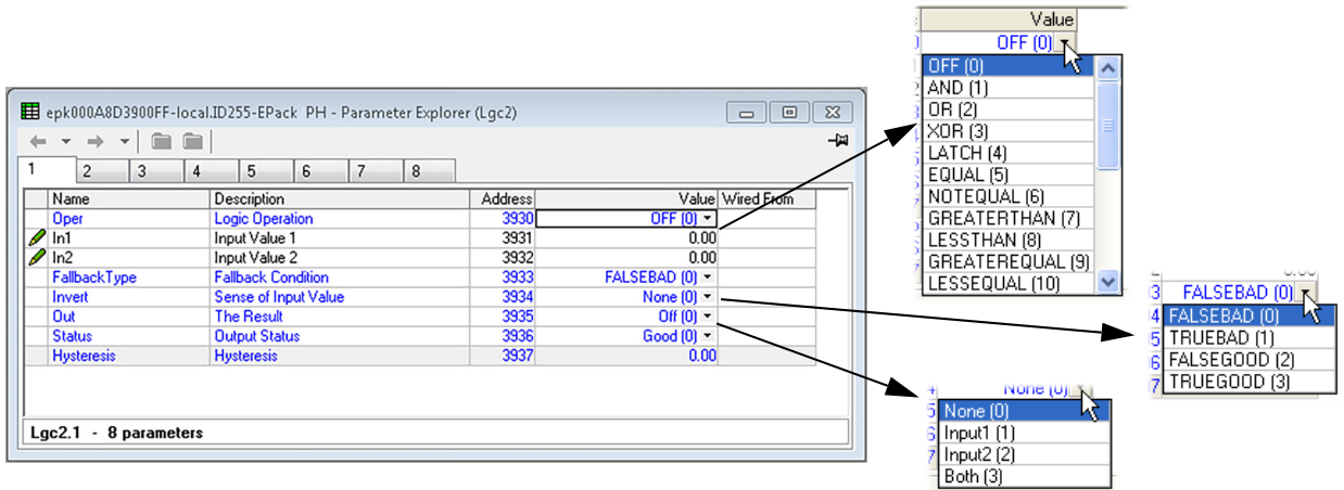
그림 105 Lgc2 페이지(Lgc2 1)
