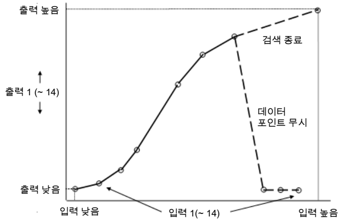
그림 110 선형화 예시
