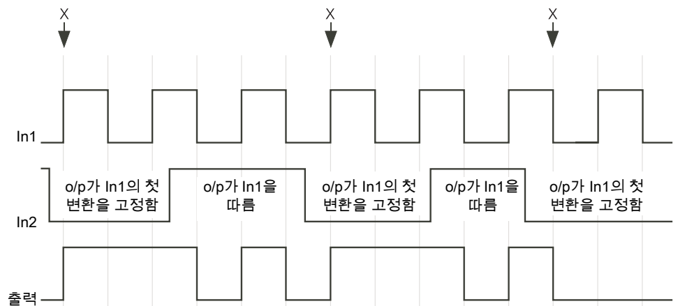
그림 106 히스테리시스
