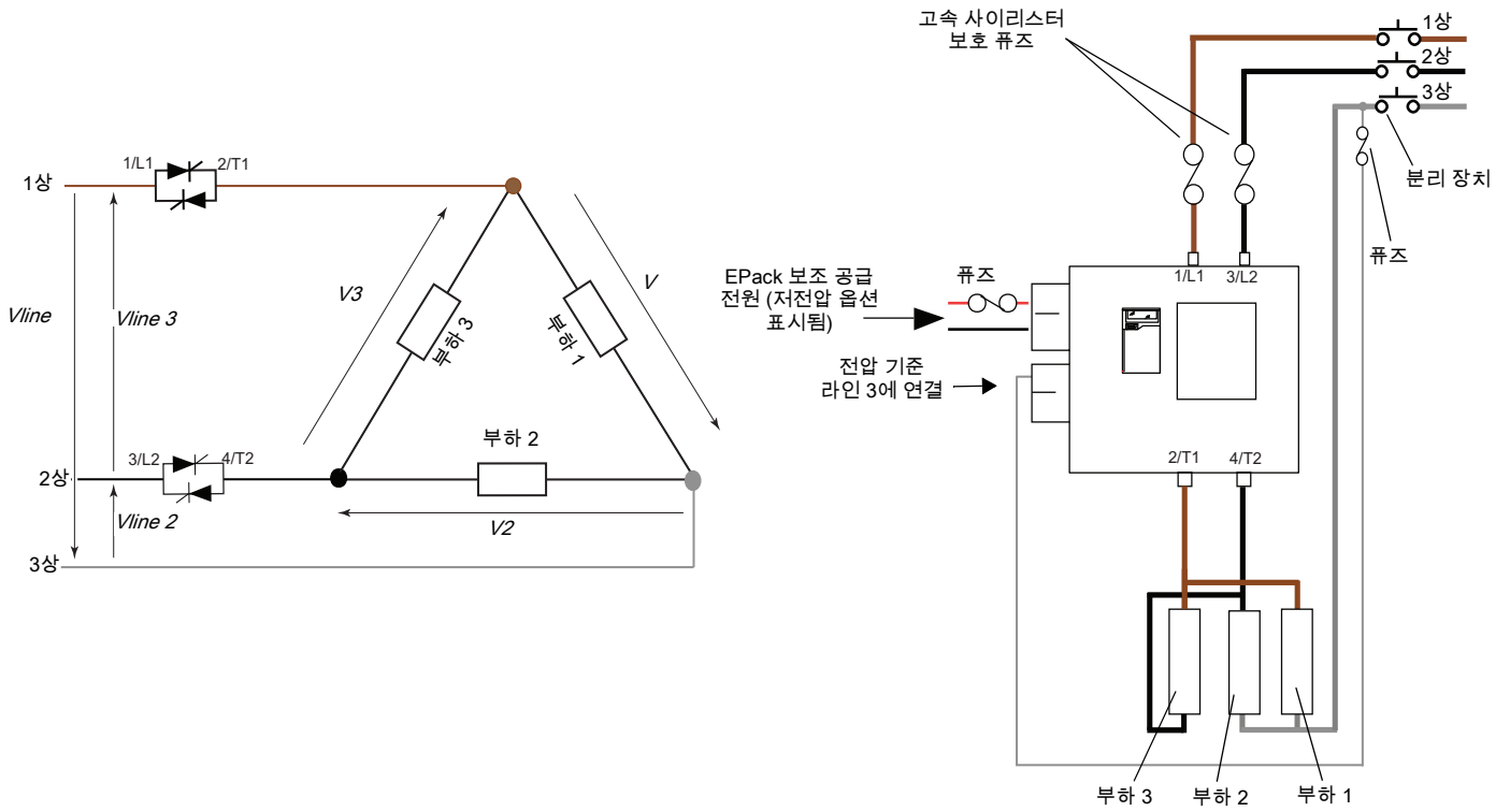
그림 10 2 phase 폐쇄 델타 배선 도해/부하 구성
