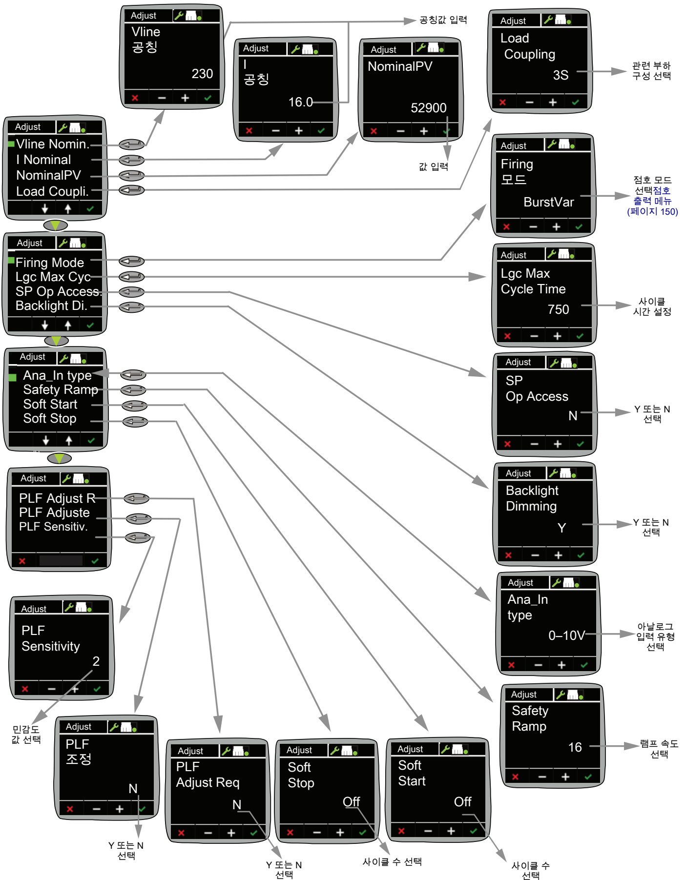
그림 56 조정 메뉴
