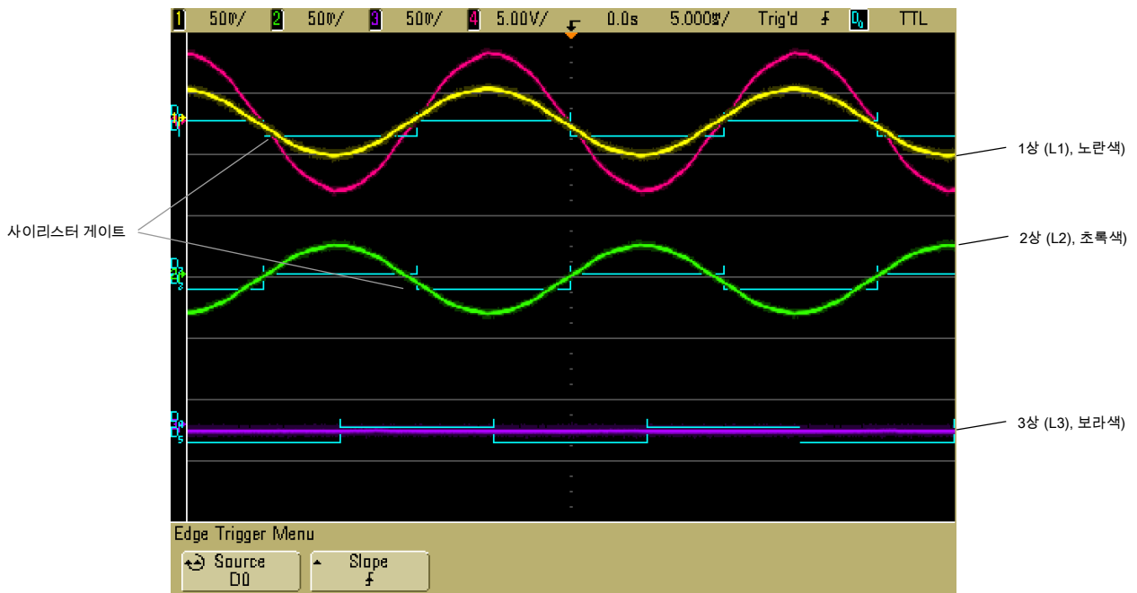
그림 93 ULM 옵션에서 불균형 부하(L3 부하 개방형 회로)인 파형이 자동으로 사이리스터 게이트와 나머지 1상 및 2상의 균형을 맞춥니다.
