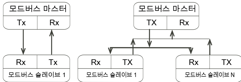
그림 35 단일 시리얼 링크 및 다분기 시리얼 링크
