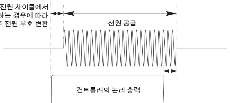
그림 17 논리 점호 모드
