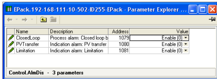
그림 77 알람 비활성화 페이지
