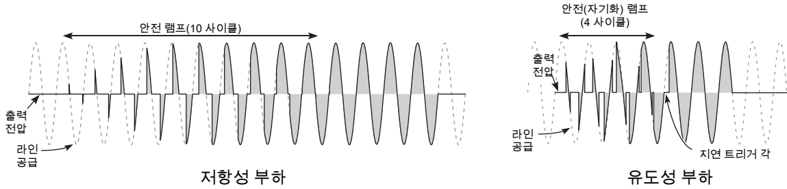
그림 95 안전 램프(버스트 점호) 예시
