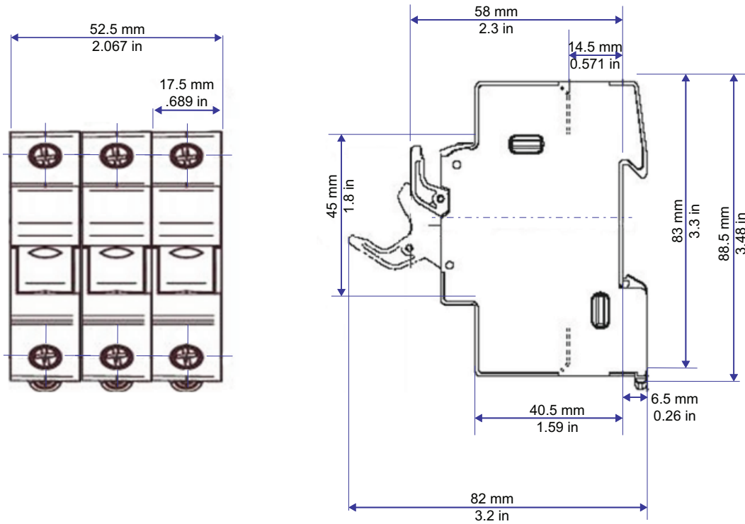
그림 150 퓨즈 홀더 치수: US103 (10x38mm)
