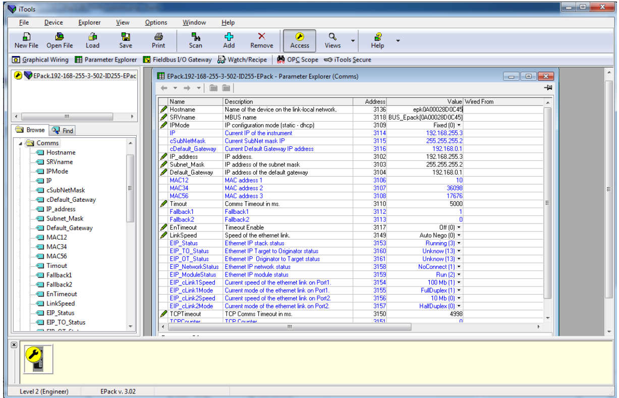
그림 26 이더넷/IP 사용자 통신 구성 매개변수
