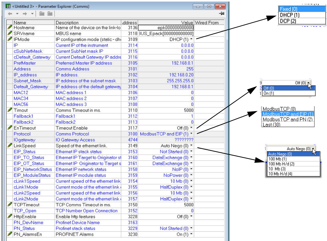
그림 77 iTools 통신 페이지
