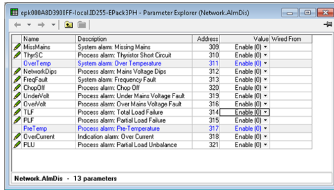
그림 123 네트워크 알람 페이지
