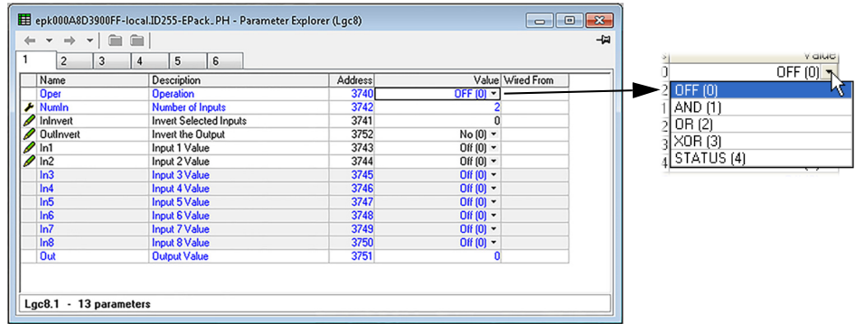
그림 114 Lgc8 구성 페이지
