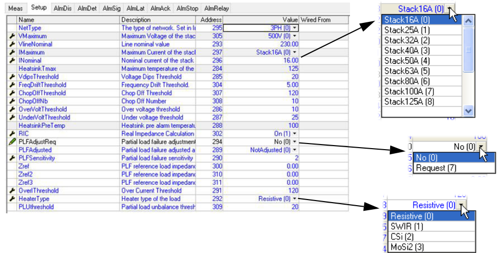
그림 122 네트워크 설정 메뉴 페이지
