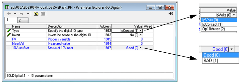
그림 103 iTools 디지털 입력 구성 페이지(디지털 입력 2 표시)
