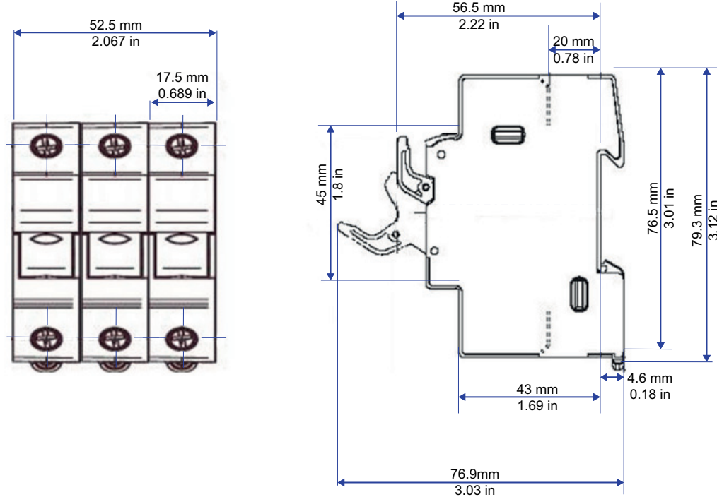
그림 151 퓨즈 홀더 치수: CUS103 (10x38mm)
