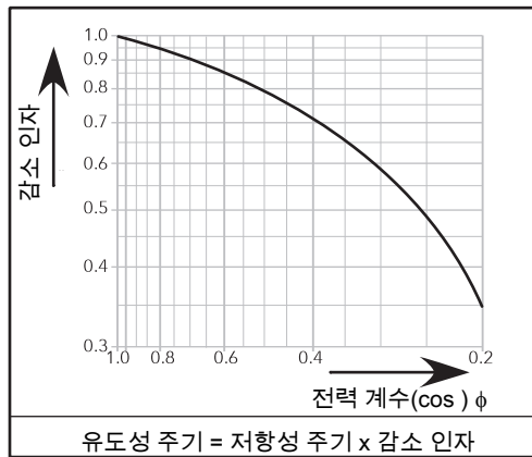
그림 159 릴레이 디레이팅 곡선
