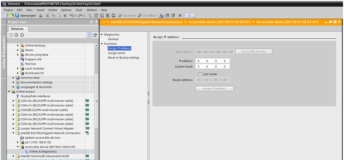
그림 47 “TIA 포털”을 통한 IP 구성 할당 및 장치 이름 할당
