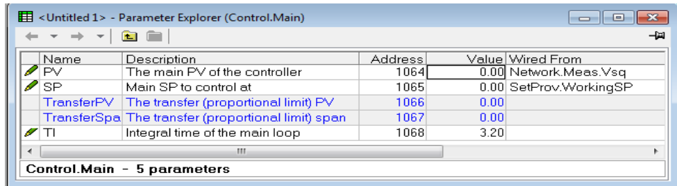
그림 80 제어 '주 전원' 메뉴
