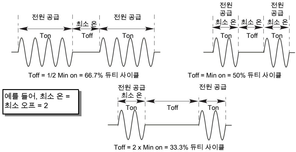
그림 21 버스트 가변 점호
