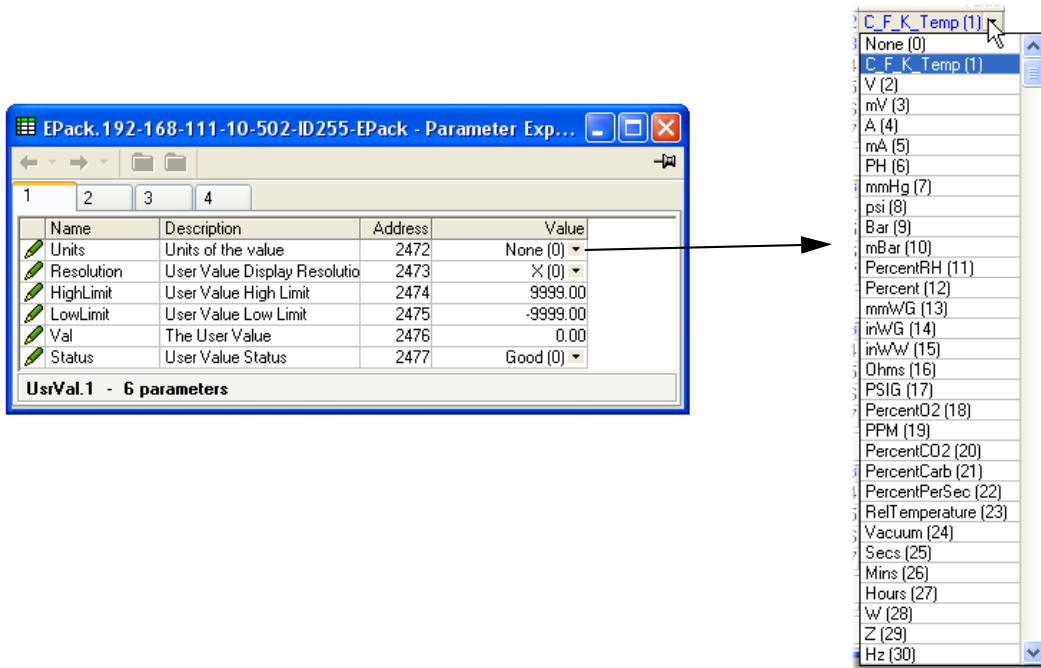
그림 129 상단 UseVal 페이지
