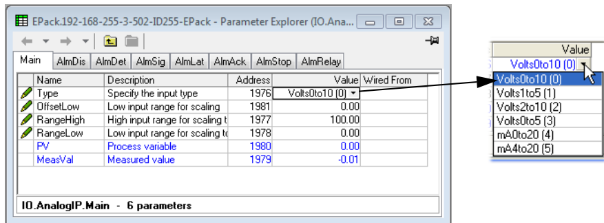
그림 101 iTools 아날로그 입력 페이지
