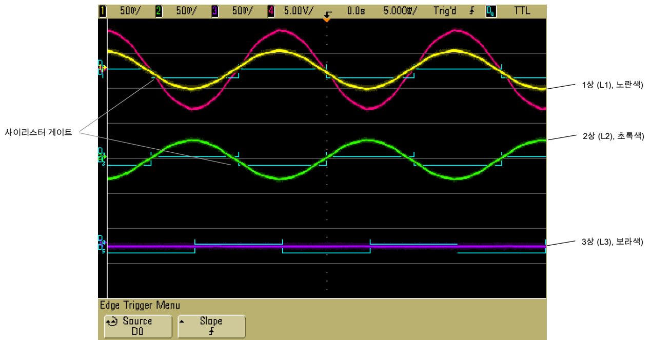
그림 99 ULM 옵션에서 불균형 부하(L3 부하 개방형 회로)인 파형이 자동으로 사이리스터 게이트와 나머지 1상 및 2상의 균형을 맞춥니다.
