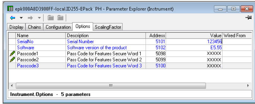
그림 108 기기 구성 페이지
