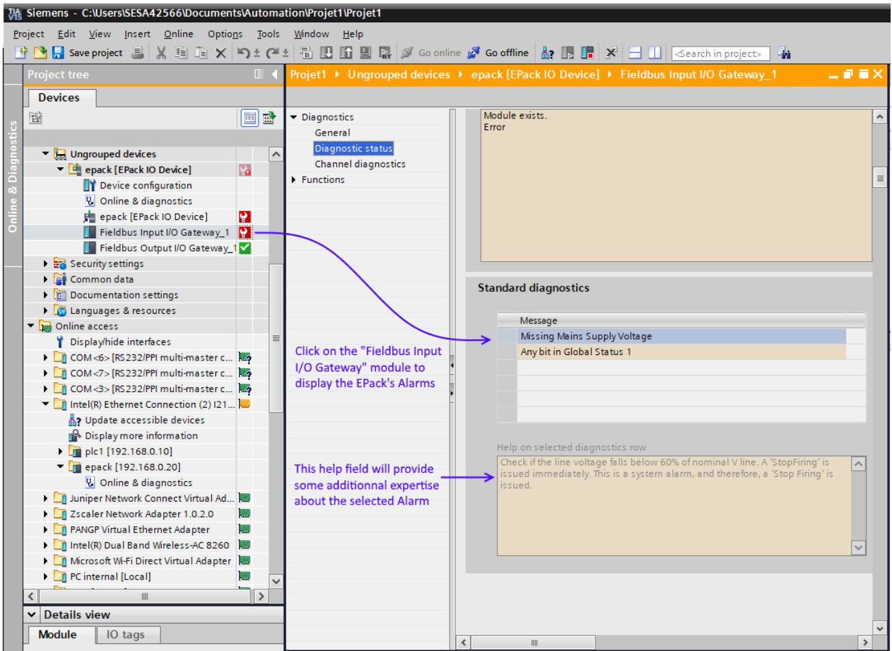
그림 56 E-Pack 알람 표시를 나타낸 TIA 포털 스크린샷
