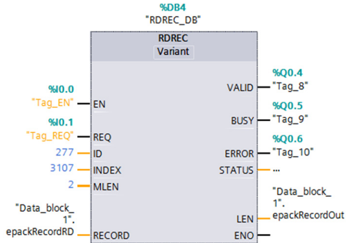
그림 54 STEP 7의 RDREC 기능 블록을 사용하여 하나의 EPack 매개변수 읽기
