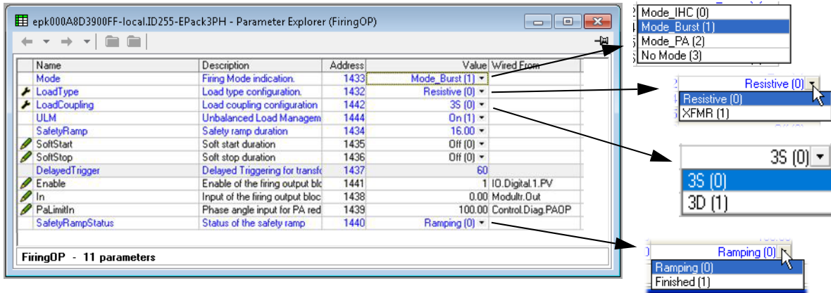
그림 94 iTools 구성 점호 출력 페이지
