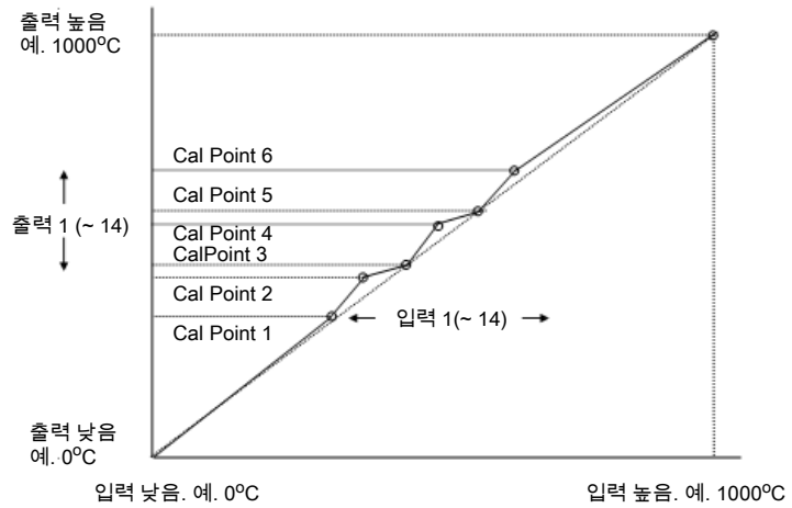
그림 118 센서 불연속 보상
