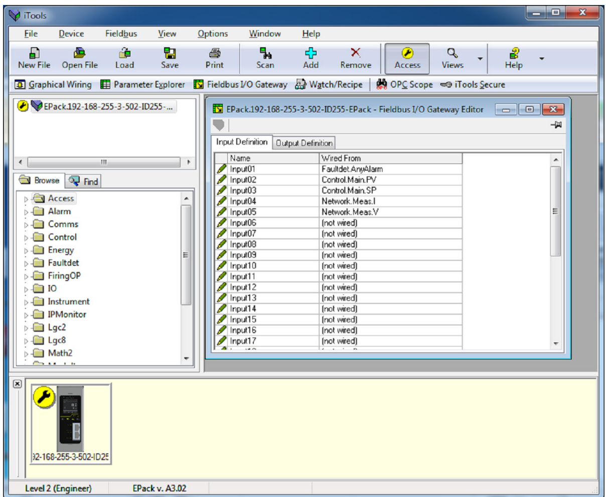
그림 27 iTools의 I/O(필드버스 I/O 게이트웨이) 에디터
