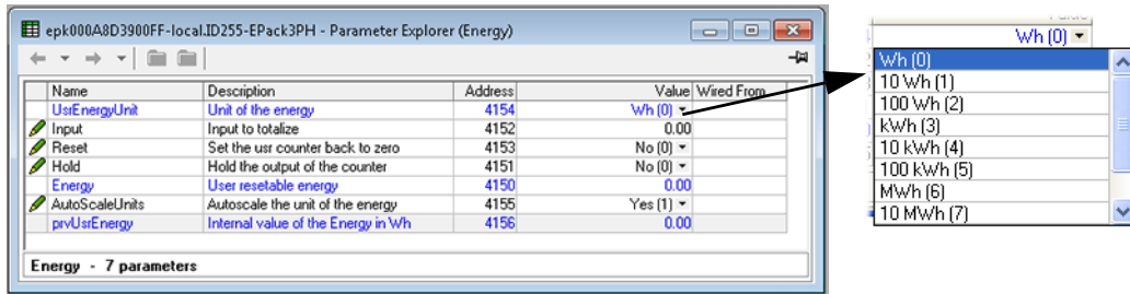
그림 92 에너지 구성 페이지
