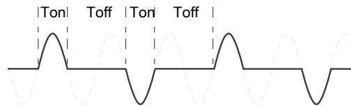
33% 듀티 사이클의 경우, T_{on} = 1 반주기, T_{off} = 2 반주기
