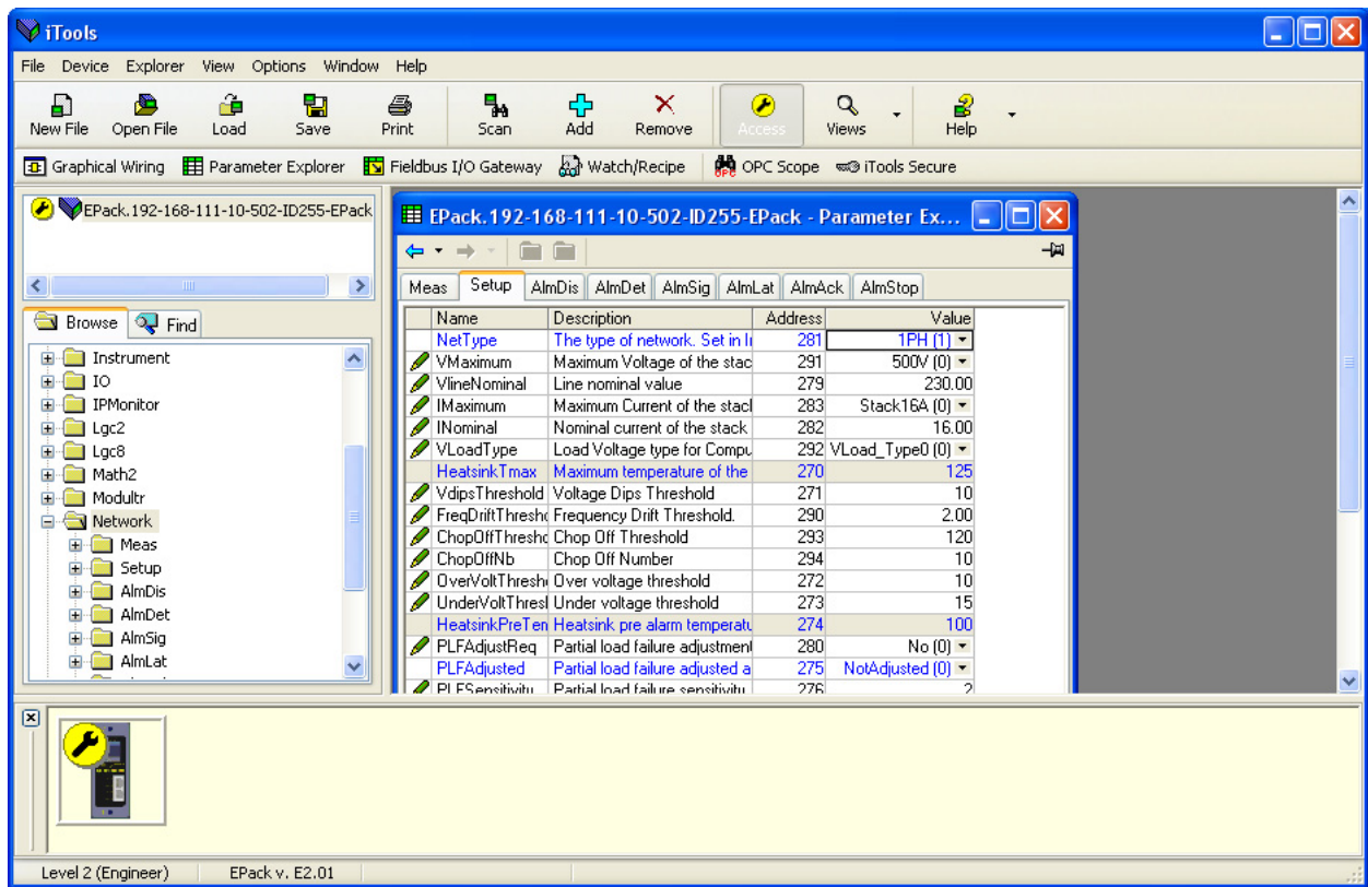
그림 142 매개변수 표 예시
