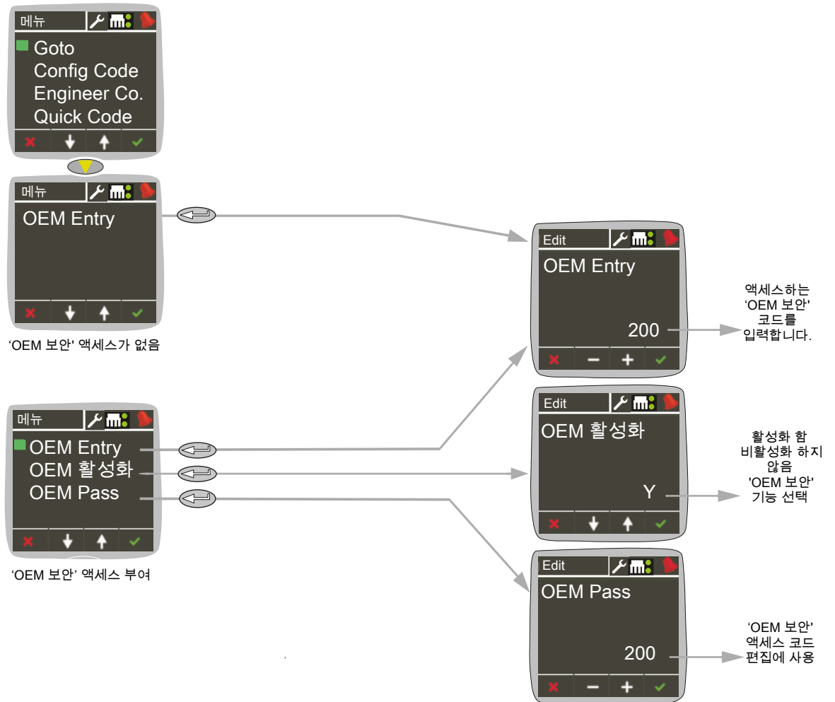
그림 73 액세스, 'OEM 보안' 메뉴
