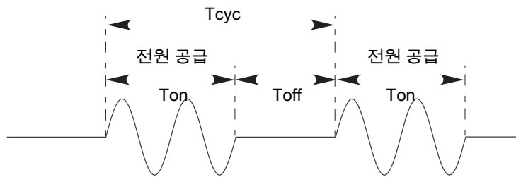
그림 20 버스트 고정 점호
