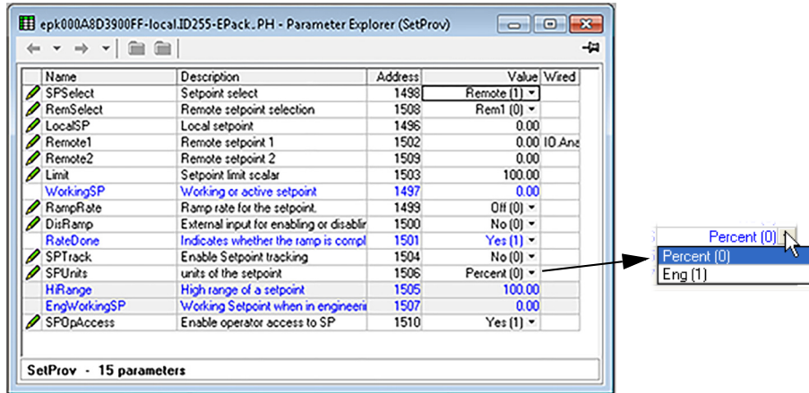
그림 125 SetProv 구성 페이지
