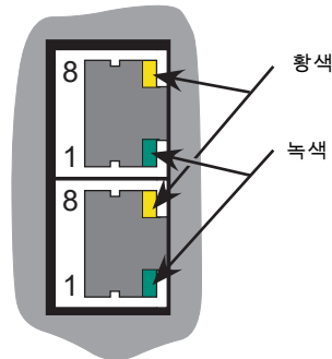
그림 15 EPack 핀 배치
