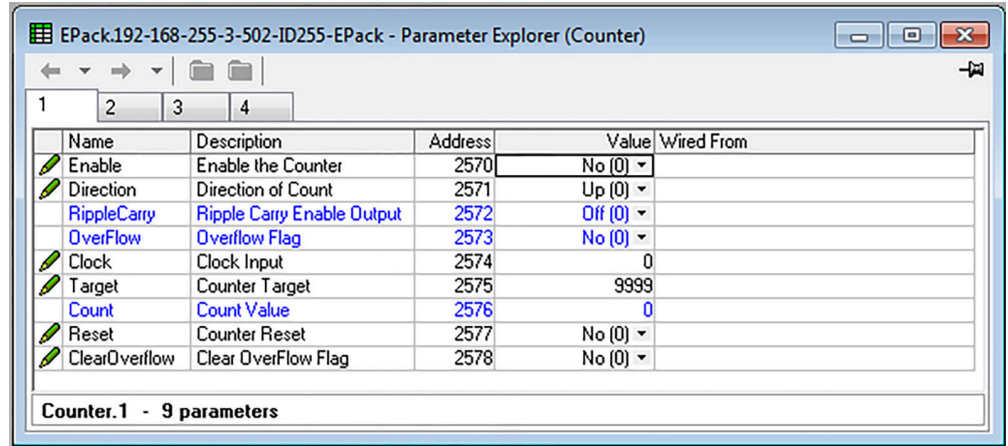
그림 90 iTools 카운터 페이지
