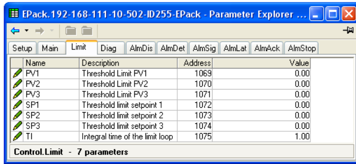
그림 81 제어 제한 메뉴
