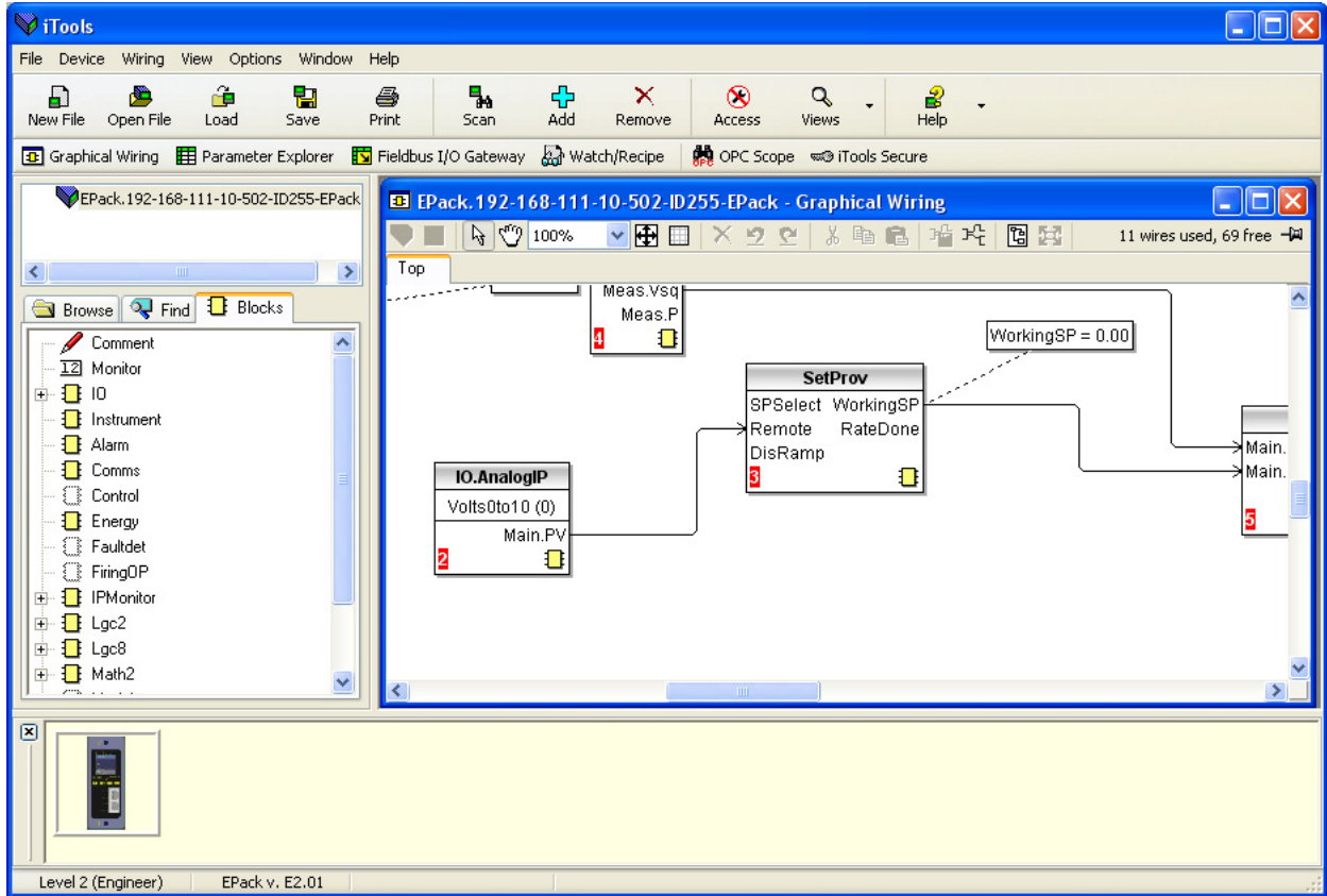
그림 133 그래픽 배선 에디터
