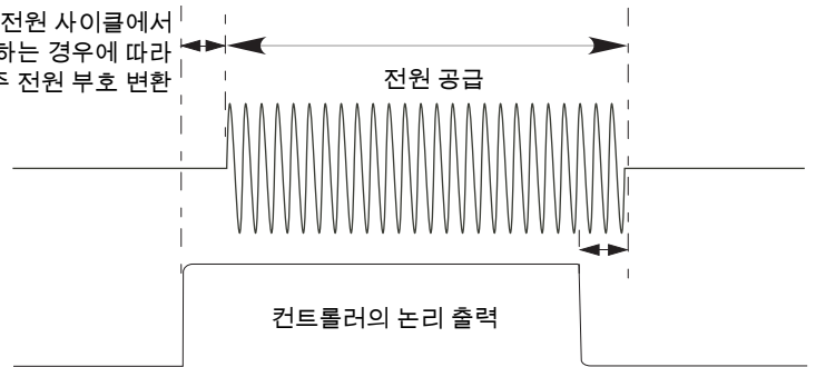
그림 19 논리 점호 모드
