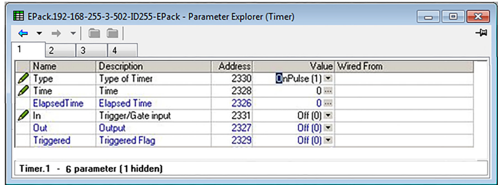
그림 126 iTools 타이머 구성
