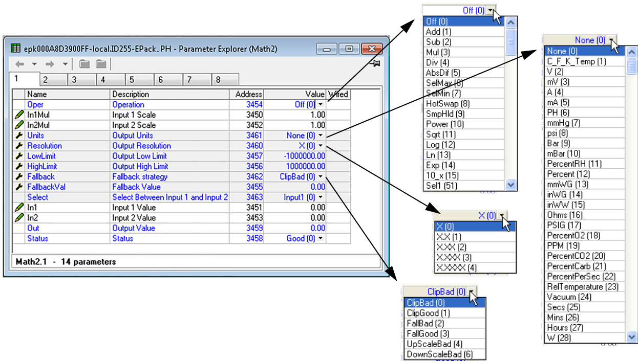
그림 119 Maths2 구성 페이지
