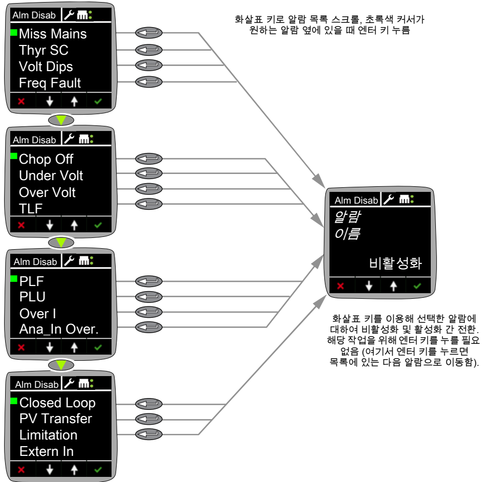
그림 66 알람 비활성화 메뉴
