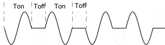
66% 듀티 사이클의 경우 T_{on} = 2 반주기, T_{off} = 1 반주기
