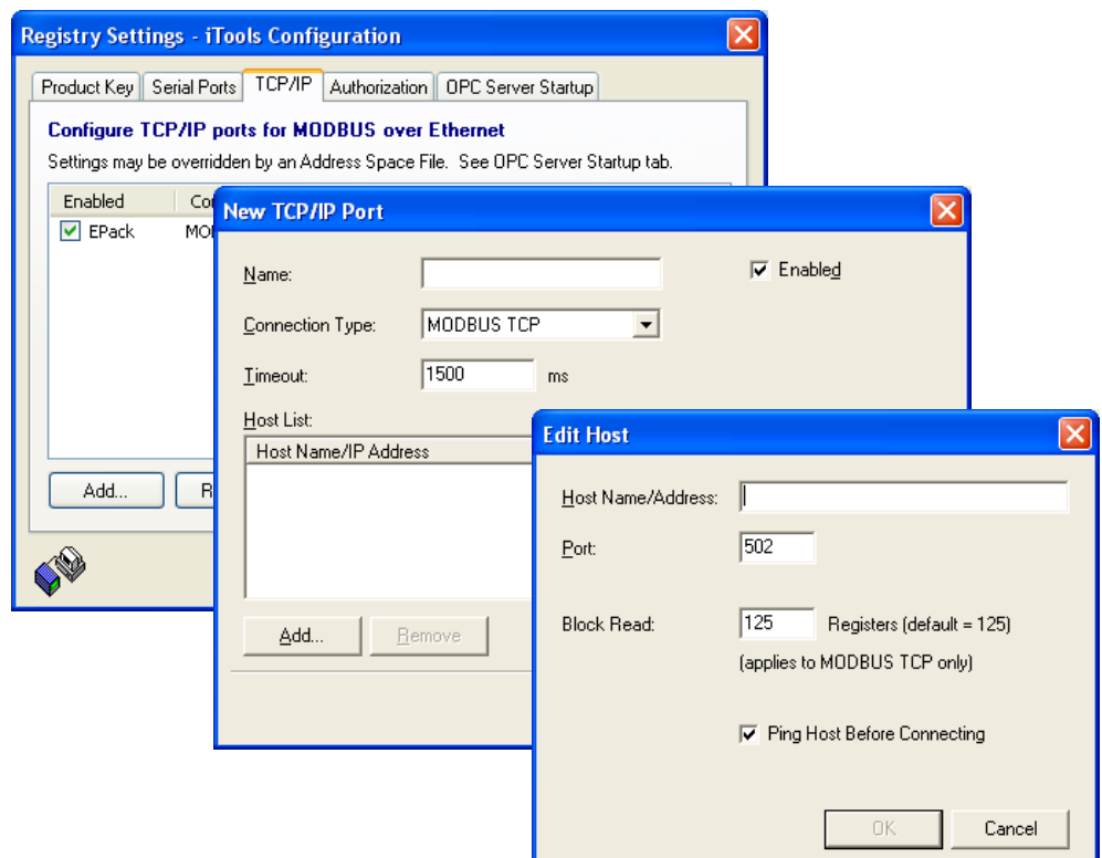
그림 131 새 이더넷 포트 추가
