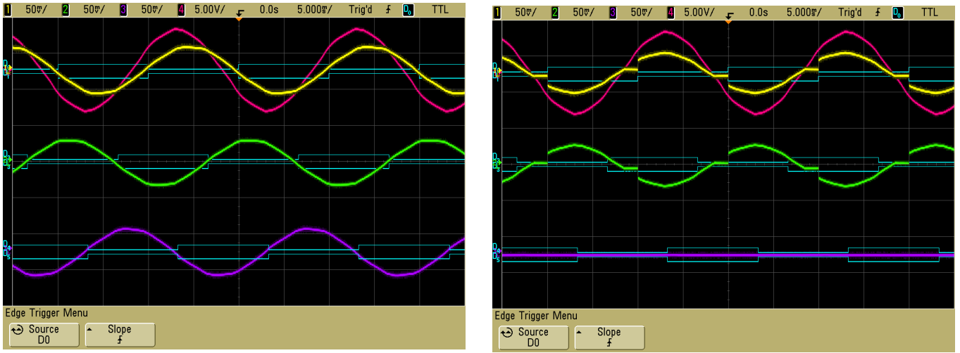
그림 98 파형: 왼쪽 균형 부하 및 오른쪽 불균형 부하(ULM 꺼짐)
