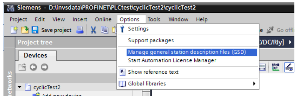
그림 50 EPack GSDML 파일을 STEP7로 로딩하기
