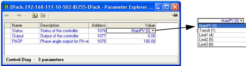
그림 82 iTools 진단 메뉴
