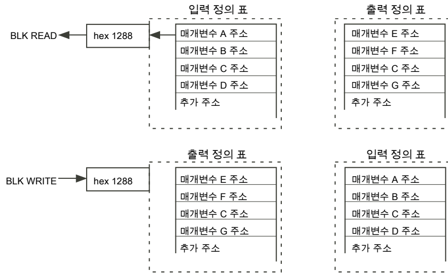
그림 148 블록 읽기 및 블록 쓰기(비교 3)
