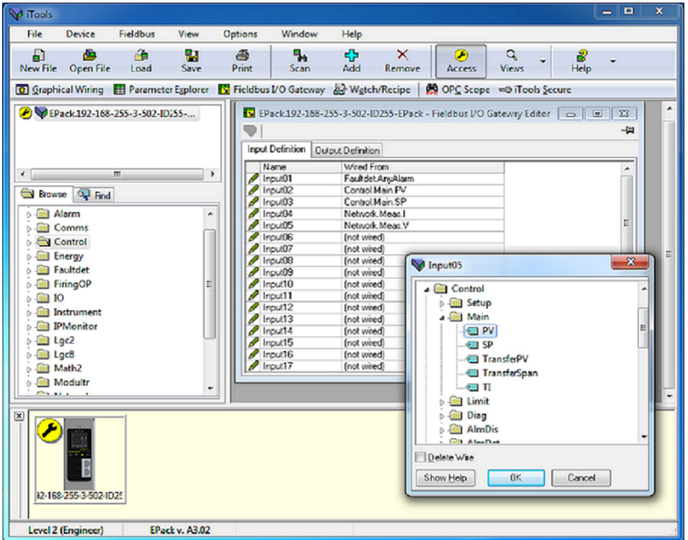
그림 28 입력값 선택 및 입력 목록의 예시
