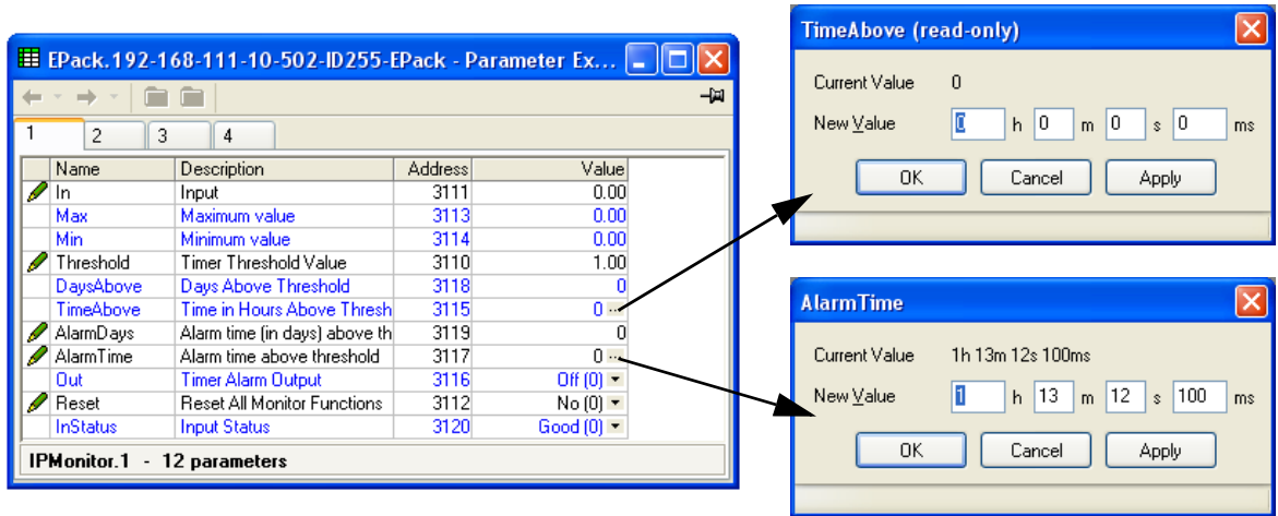
그림 110 iTools 입력 모니터 페이지(IPMon1)
