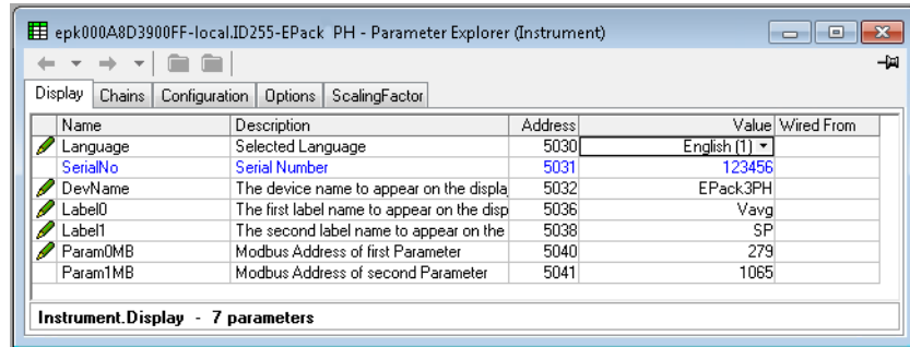
그림 105 상단 기기 구성 페이지
