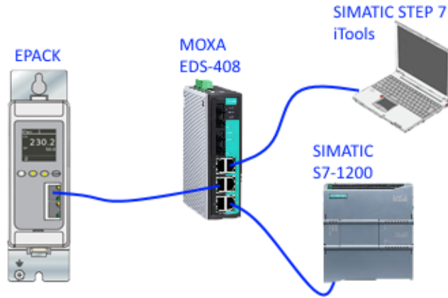
그림 44 구성 도구 연결
