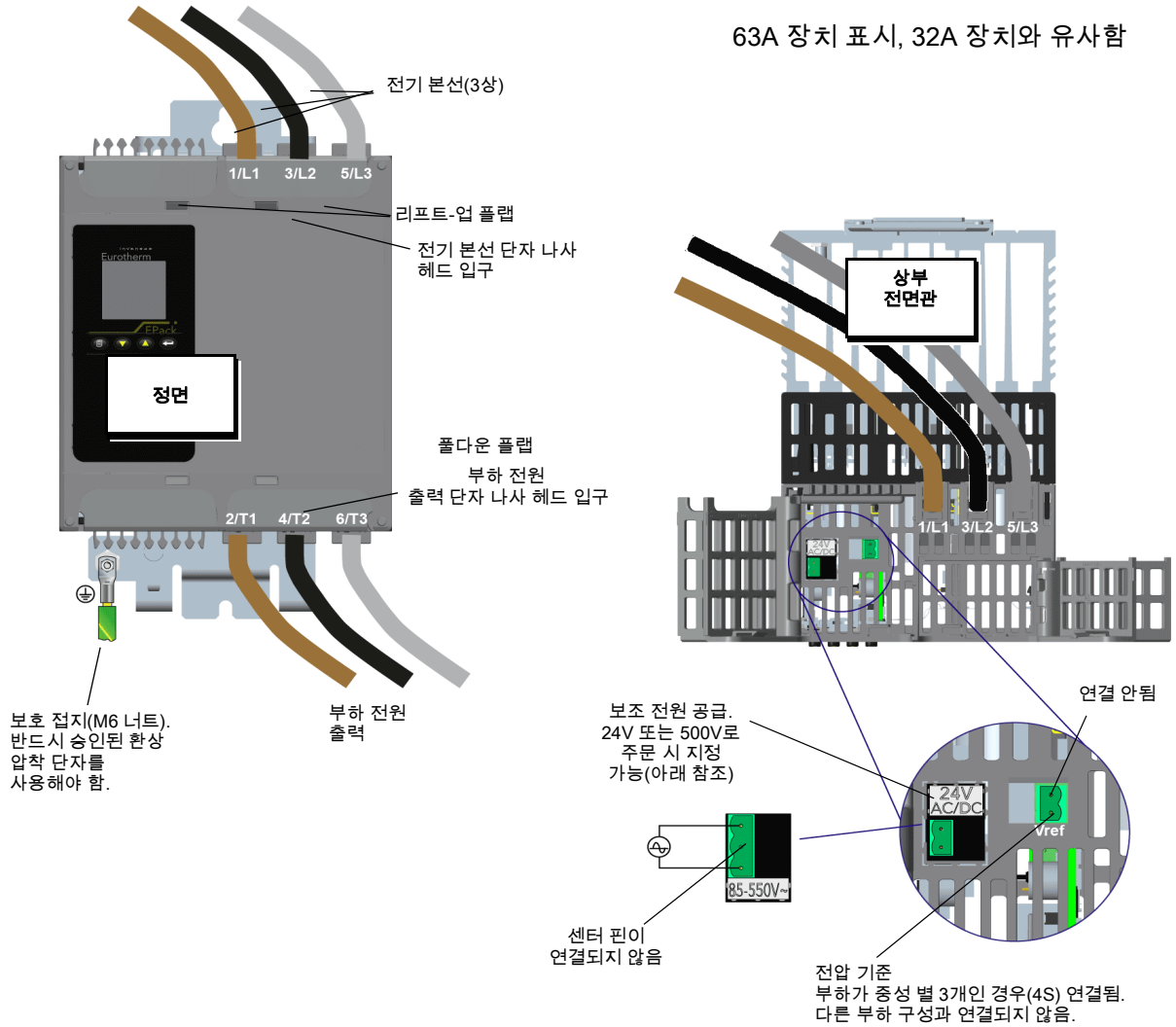
그림 8 공급 전원 및 부하 연결 세부 사항(16A ~ 63A 장치)
