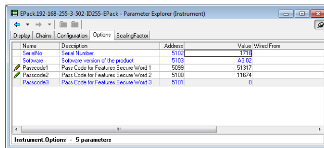
그림 157 기기 옵션 구성
