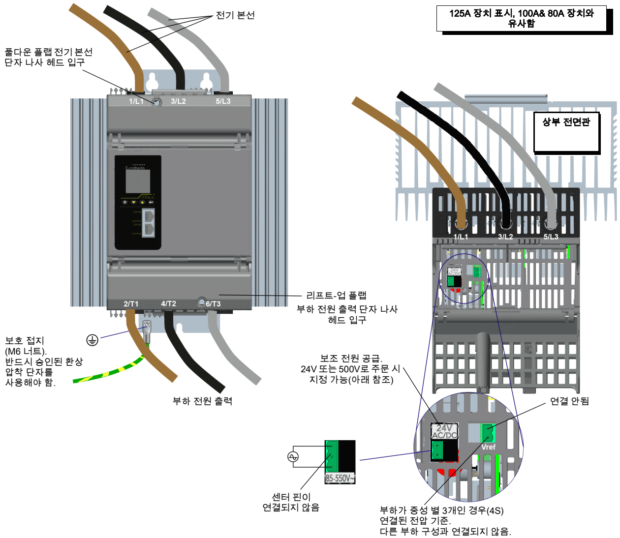
그림 9 공급 전원 및 부하 연결 세부 사항(80A ~ 125A 장치)(125A 표시). 기본적인 배선 세부 사항은 그림 9을 참조하십시오.
