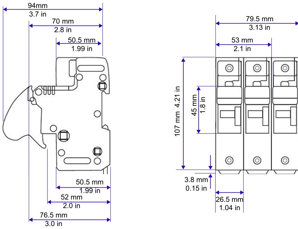
그림 152 퓨즈 홀더 치수: US143 (14x51mm)
