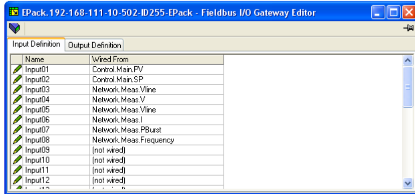
그림 146 일반적인 필드버스 게이트웨이 매개변수 목록
