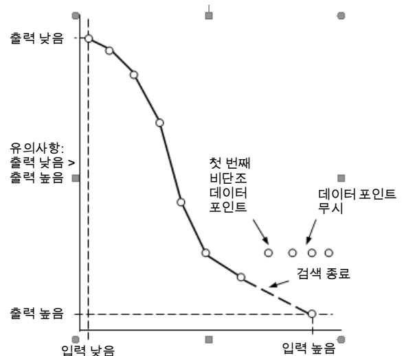
그림 117 비단조 데이터를 감지하는 경우 역곡선이 검색을 종료하는 방식
