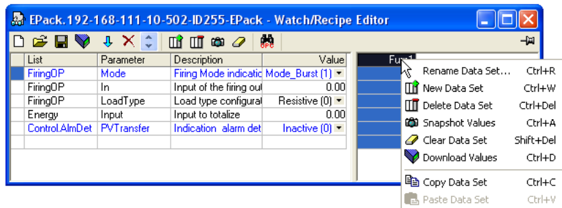
그림 149 와치/레시피 에디터 창(컨텍스트 메뉴 포함)
