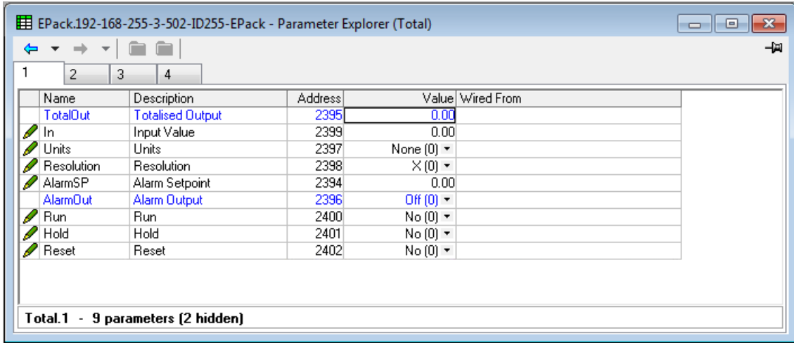
그림 128 iTools 통합기 페이지
