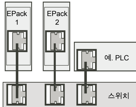
그림 43 PROFINET 배선 - 여러 개의 컨트롤러
