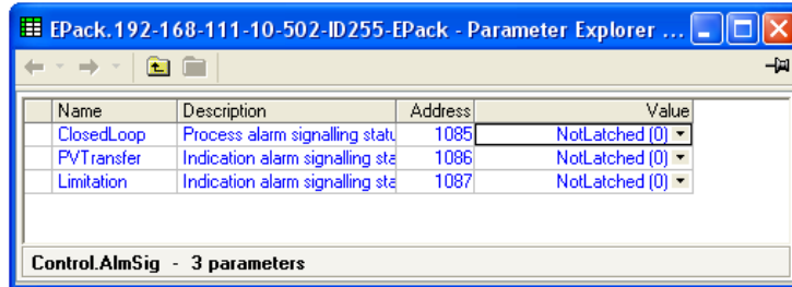
그림 85 제어 알람 신호 전송 페이지
