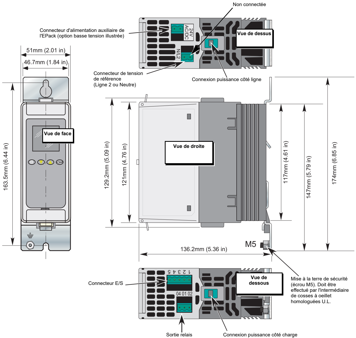
Figure 4 Détails de l'installation mécanique (produits 16 A à 32 A).
