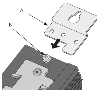
Figure 1 Installation de la fixation de montage en fond d'armoire (contrôleur 32 A présenté ; contrôleurs 63 A similaires)
