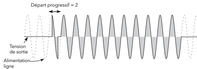
Figure 20 Exemple de démarrage progressif
