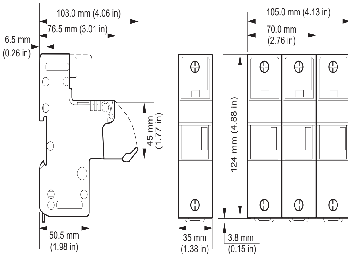
Figure 35 Dimensions du porte-fusible : US221 (22x58 mm)
