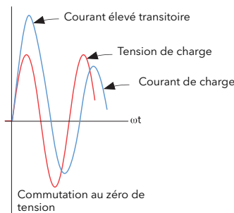
Figure 21 Définition du déclenchement retardé
