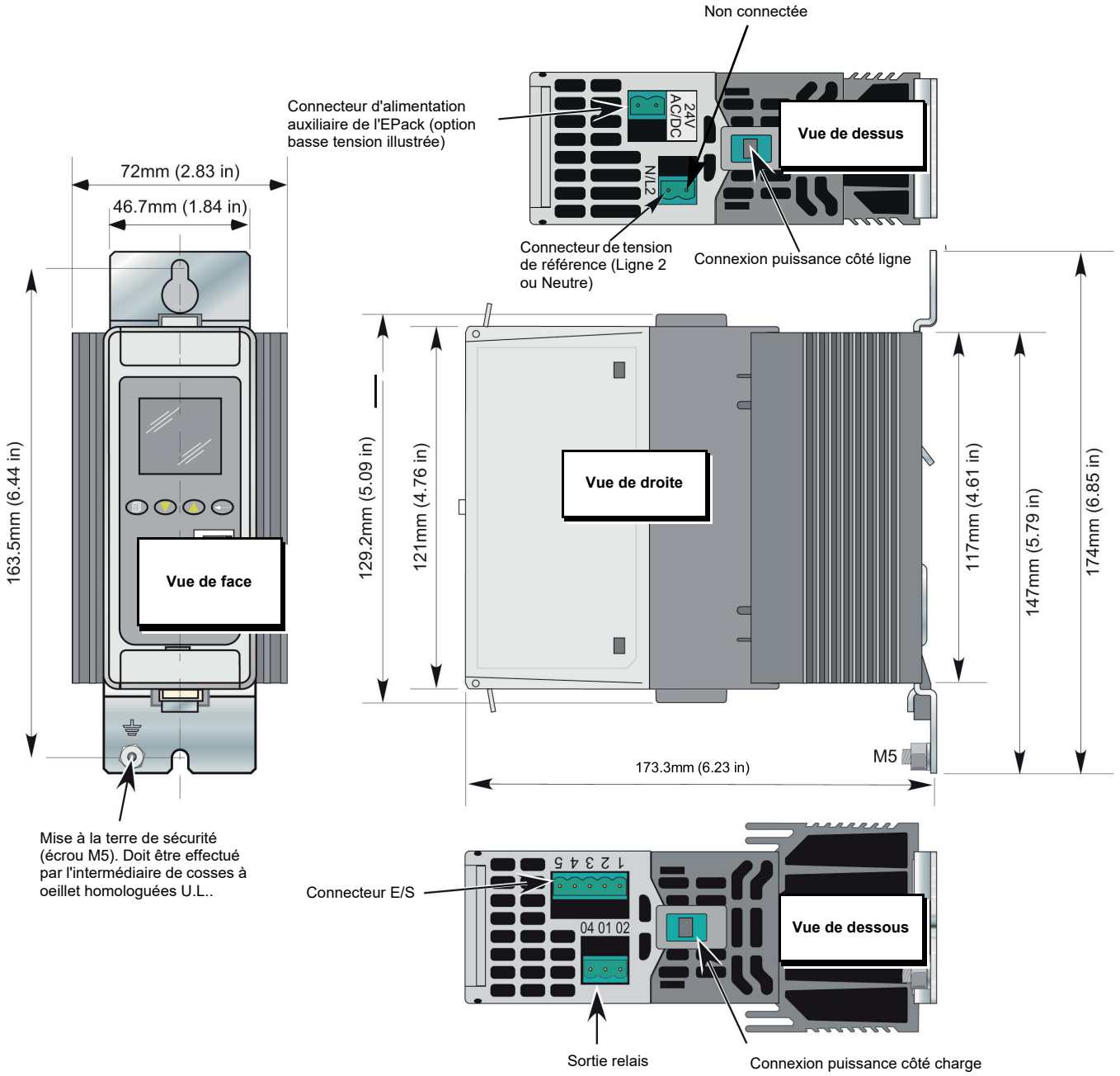
Figure 5 Détails de l'installation mécanique (produits 40 A à 63 A).
