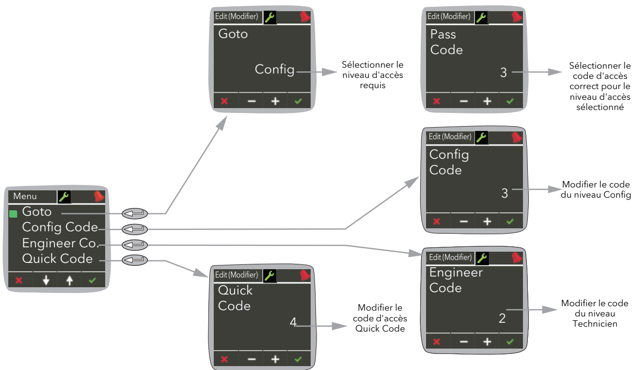
Figure 31 Menu Access (Accès)
