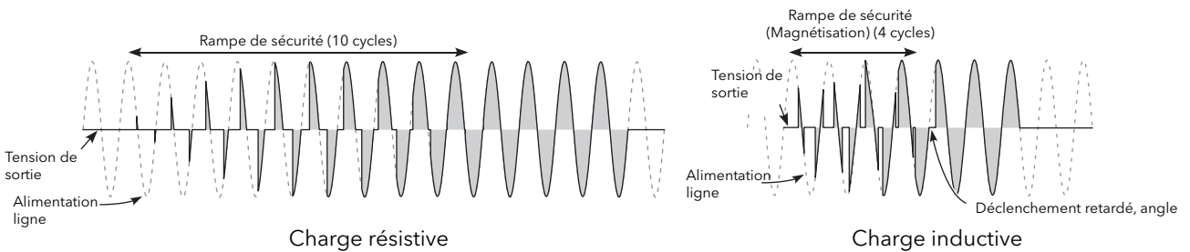
Figure 19 Exemples de rampe de sécurité (en train d'ondes)
