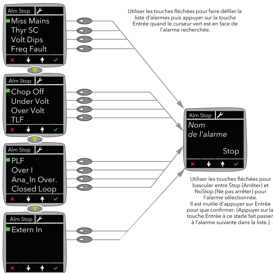
Figure 27 Menu Alarm Stop (Arrêt des alarmes)
