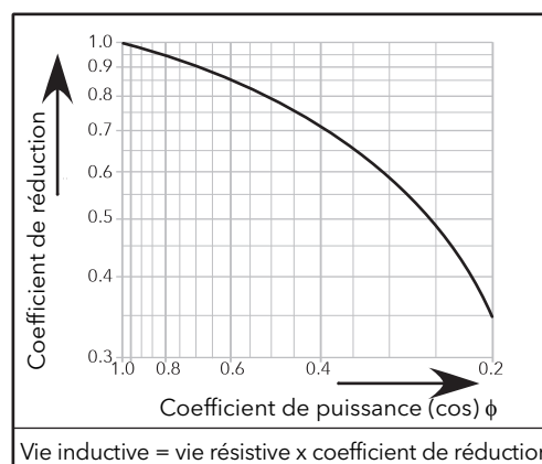
Figure 37 Courbes de déclassement relais
