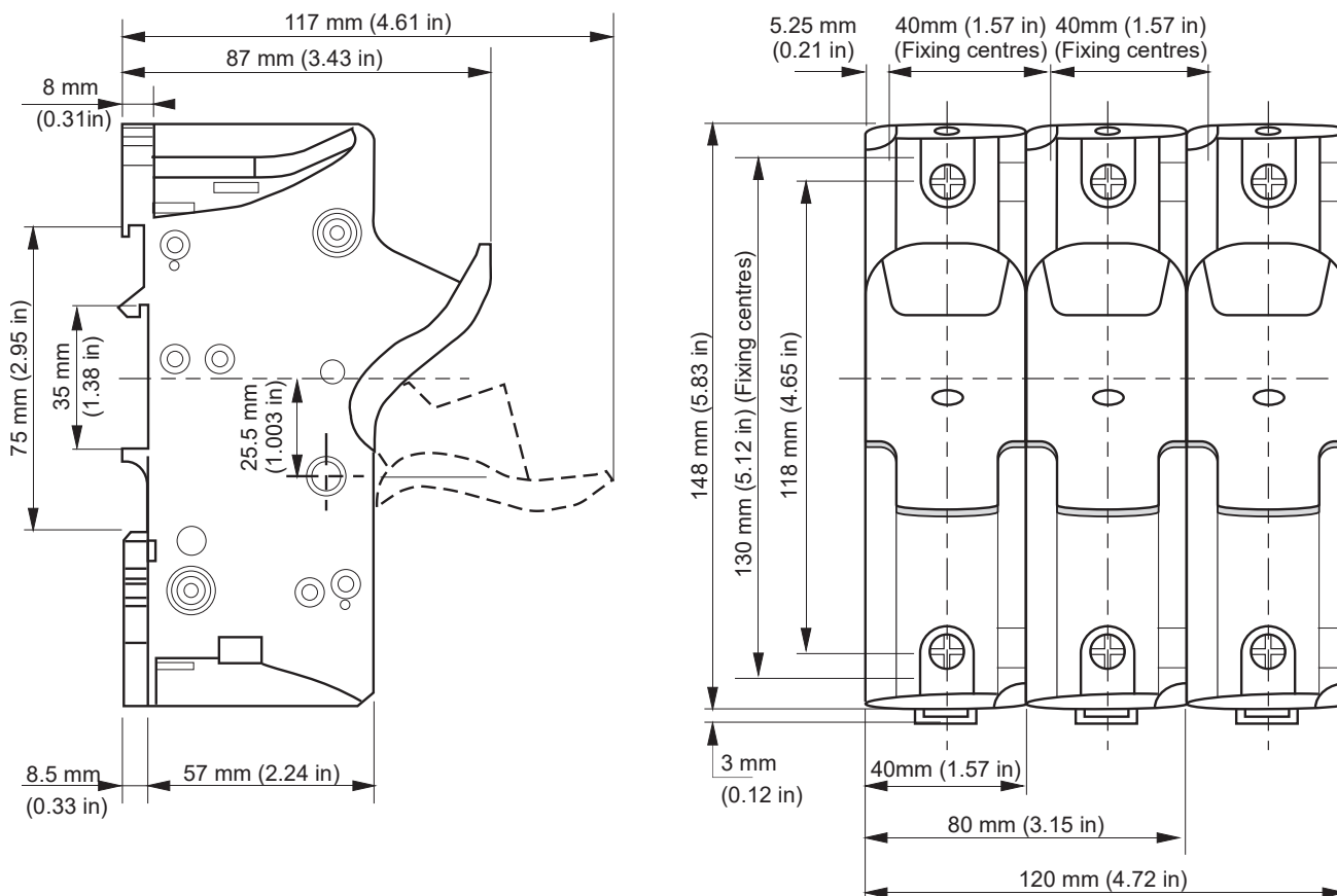
Figure 36 Dimensions des porte-fusibles : US271 (27x60 mm)
