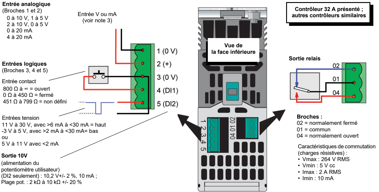
Figure 10 Détails E/S
