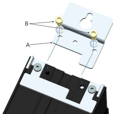
Figure 2 Montage en fond d'armoire du contrôleur 80 A/100 A illustré (modèle 125 A similaire)
