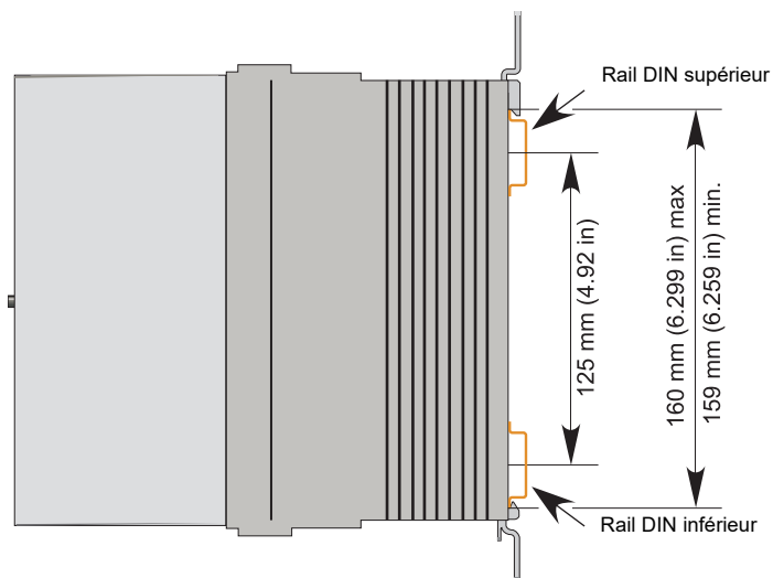
Figure 3 Détails de montage des rails DIN pour les produits 80 A, 100 A et 125 A
