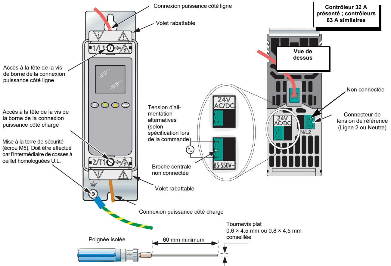
Tournevis/Clé dynamométrique, détails de l'embout pour la terminaison de ligne et de charge
