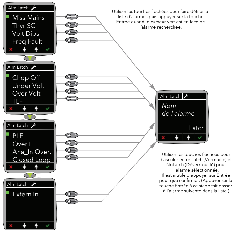
Figure 26 Menu Alarm Latch (Verrouillage des alarmes)
