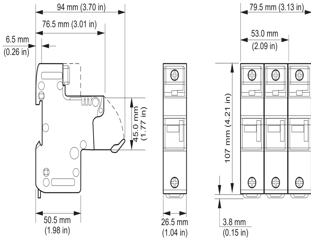
Figure 34 Dimensions des porte-fusibles : US141 (14x51 mm)
