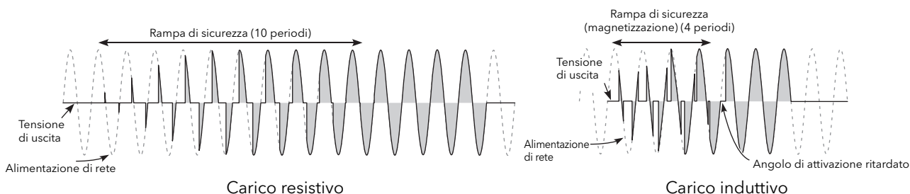
Figura 19 Esempi di rampa di sicurezza (accensione a treno di impulsi)
