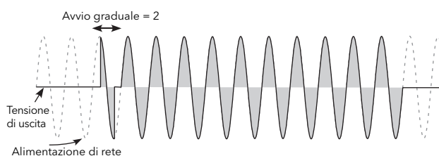
Figura 20 Esempio di avvio graduale
