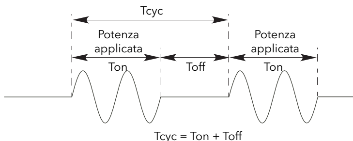
Figura 14 Modalità accensione fissa a treno di impulsi
