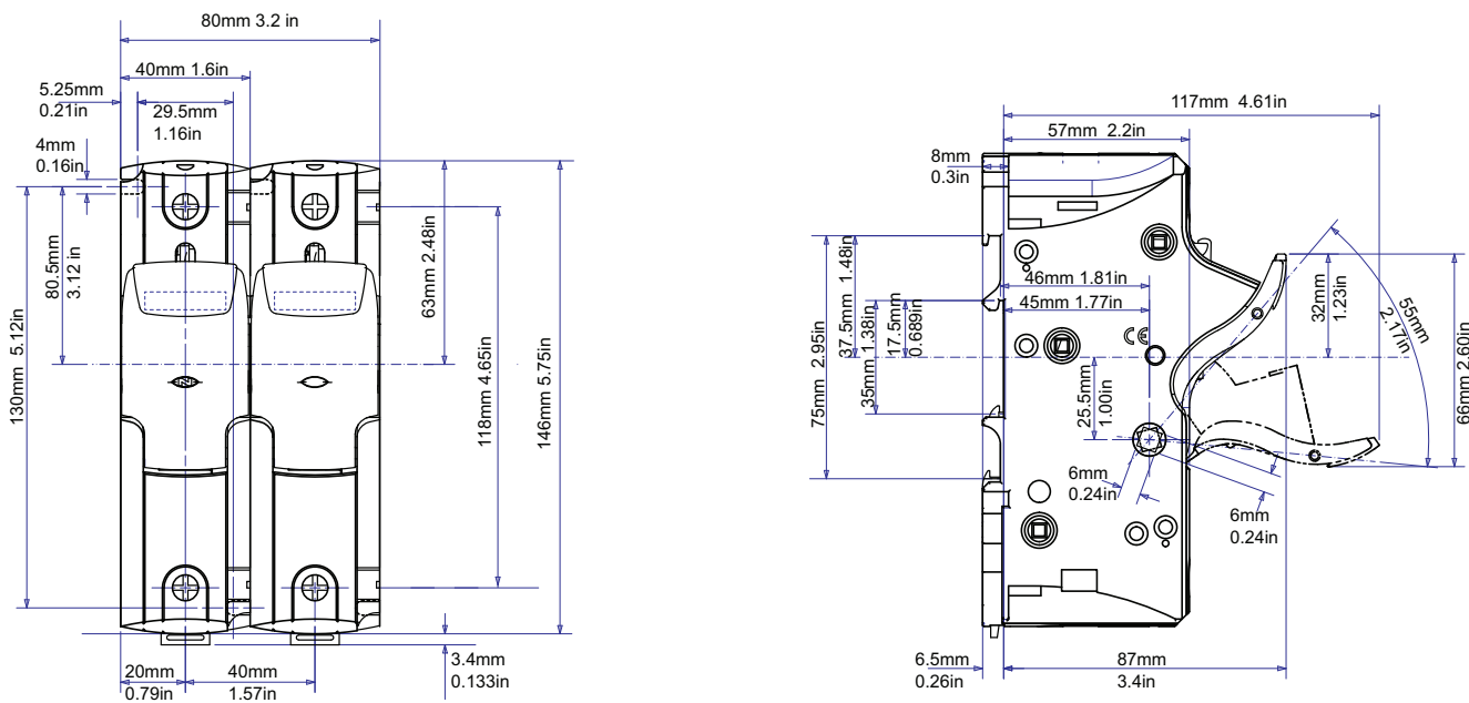
Figura 37 Dimensioni dei portafusibili: US222 (22x58 mm)
