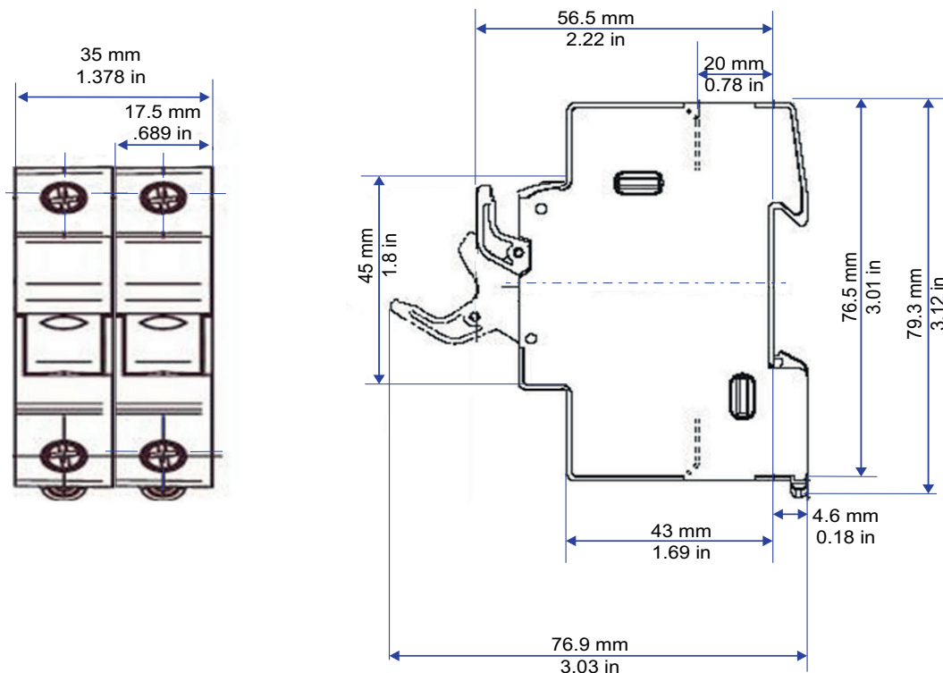
Figura 35 Dimensioni dei portafusibili: CUS102 (10x38 mm)
