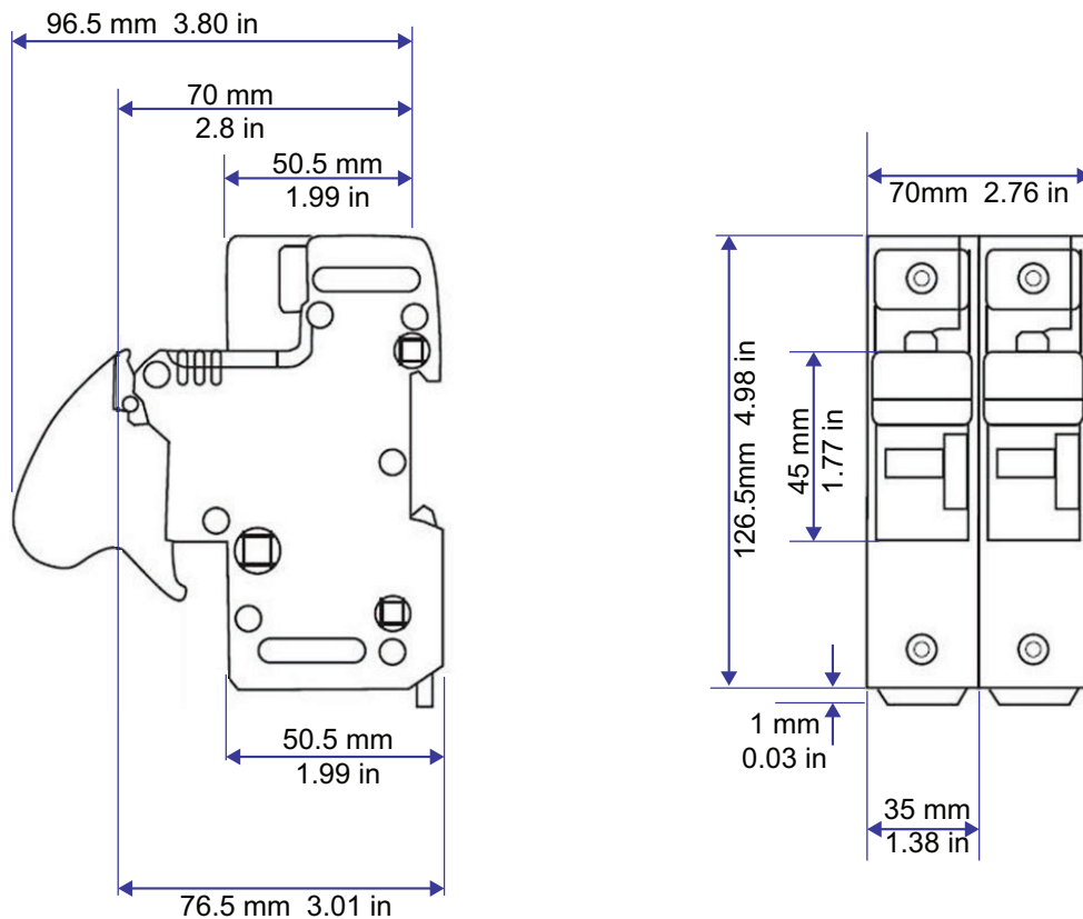
Figura 37 Dimensioni dei portafusibili: US222 (22x58 mm)
