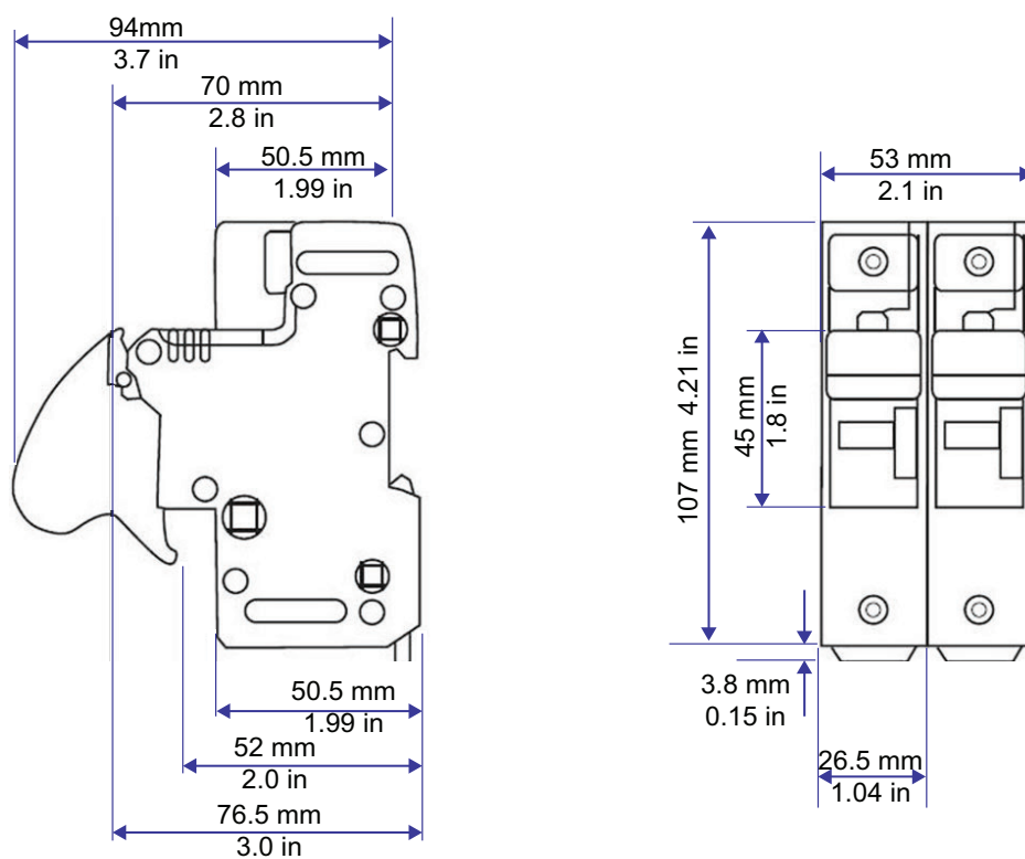
Figura 36 Dimensioni dei portafusibili: US142 (14x51 mm)
