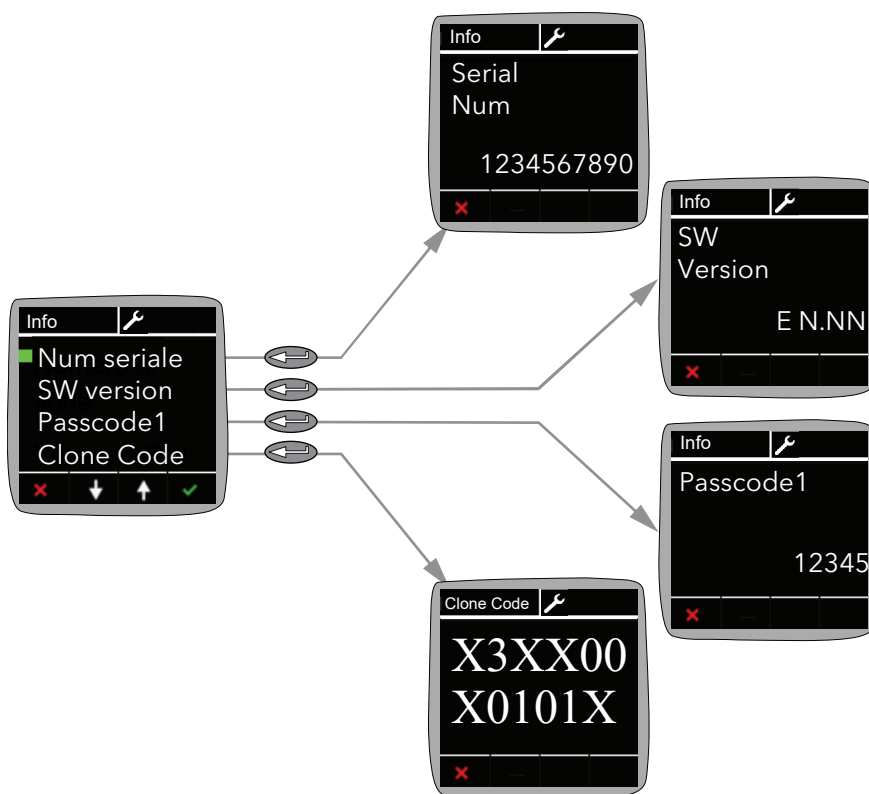
Figura 25 Menu Info
