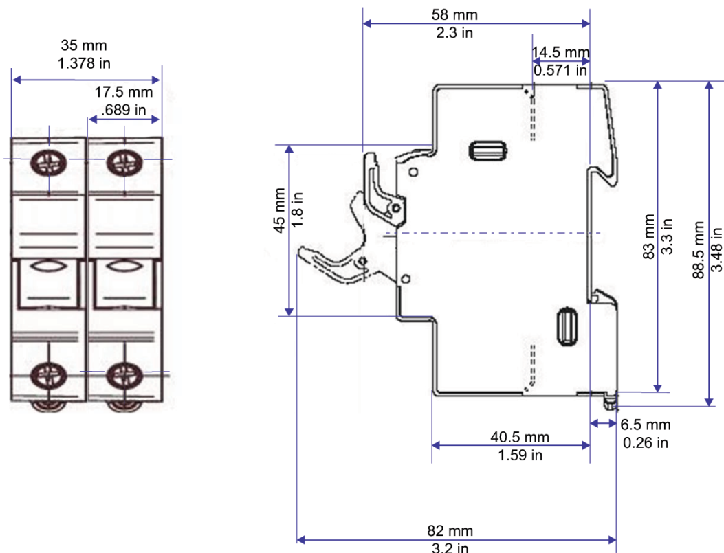
Figura 34 Dimensioni dei portafusibili: US102 (10x38 mm)
