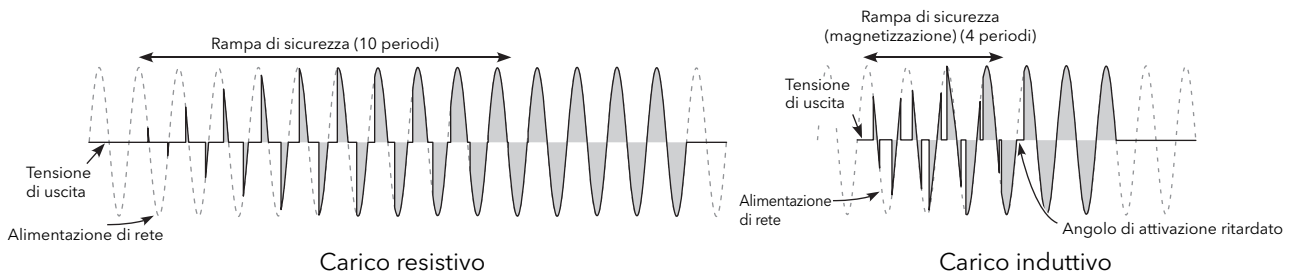
Figura 21 Esempi di rampa di sicurezza (accensione a treno di impulsi)
