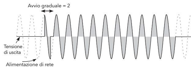
Figura 22 Esempio di avvio graduale
