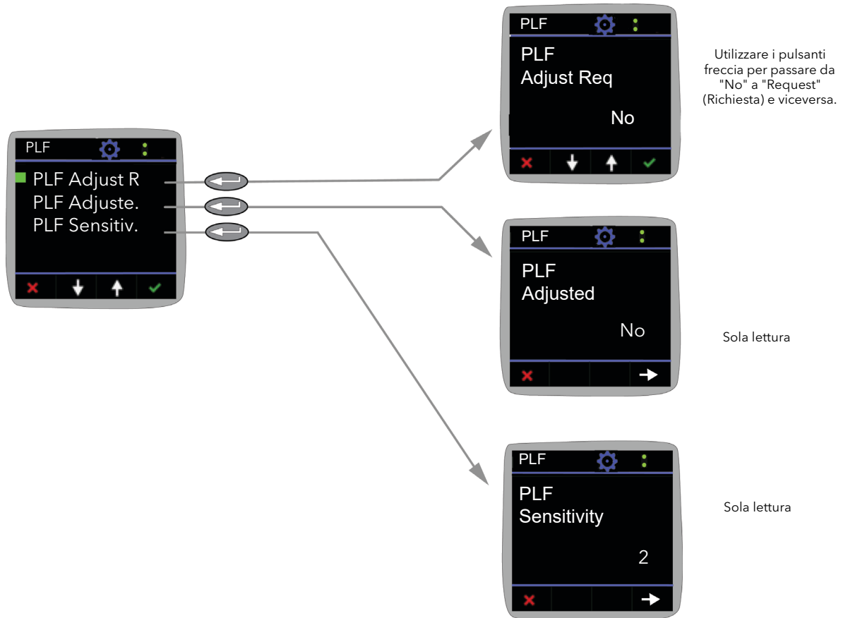
Figura 24 Menu PLF
