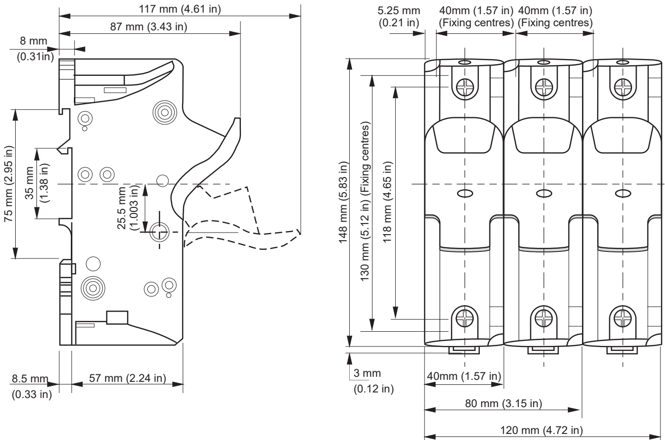
그림 36 퓨즈 홀더 치수: US271 (27x60mm)
