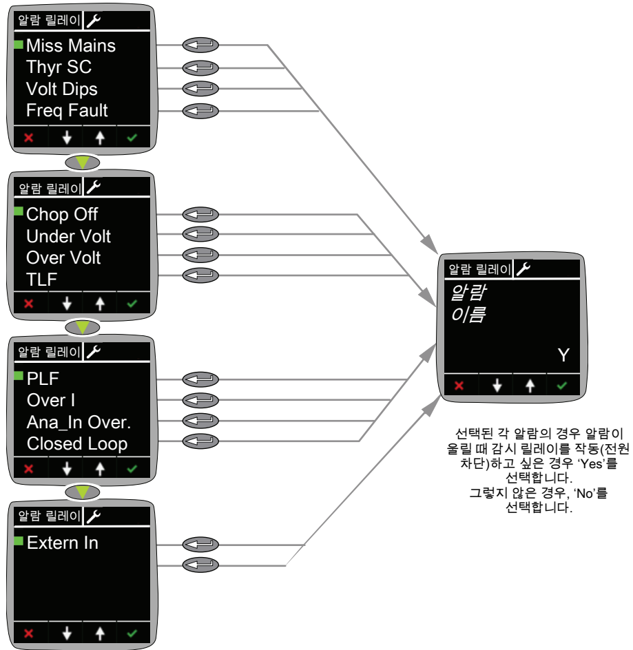
그림 28 알람 릴레이 메뉴
