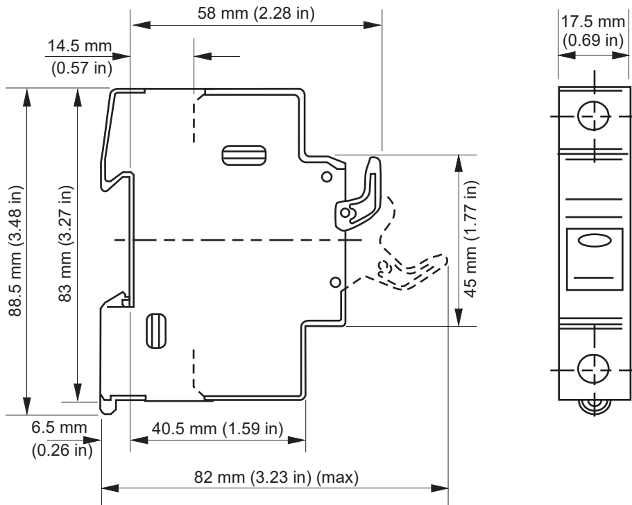
그림 32 퓨즈 홀더 치수: US101 (10x38mm)
