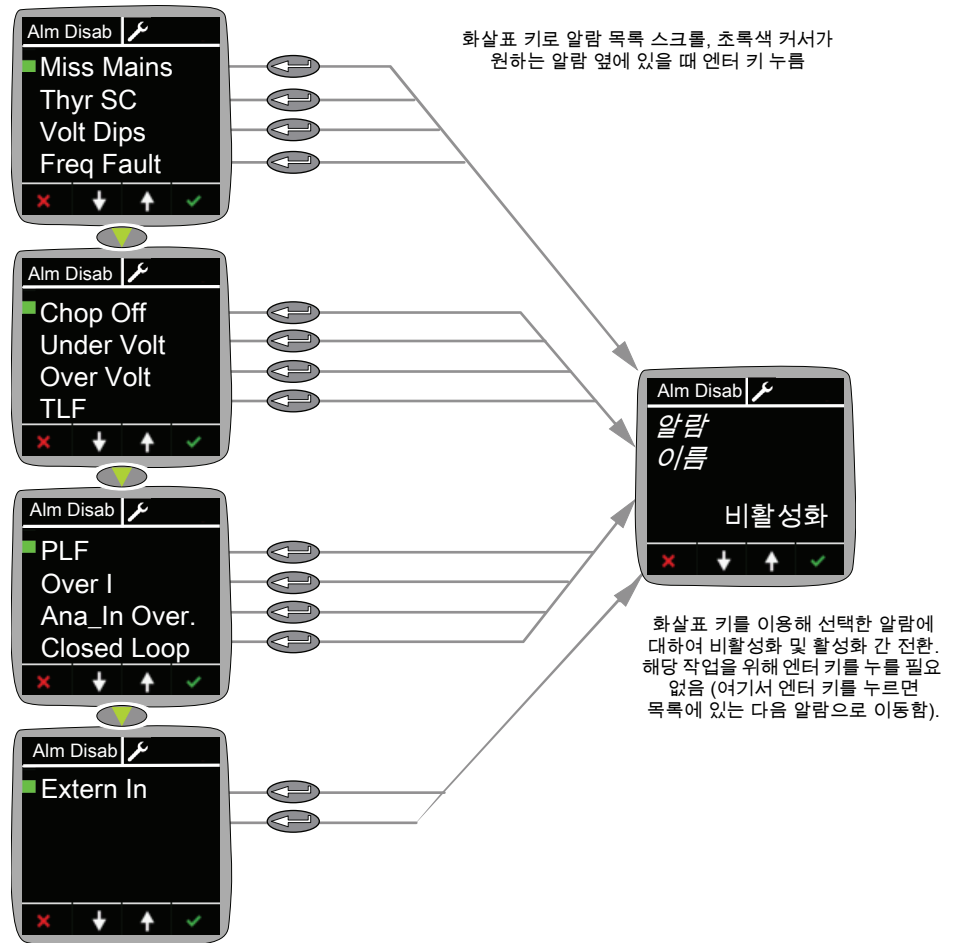
그림 25 알람 비활성화 메뉴
