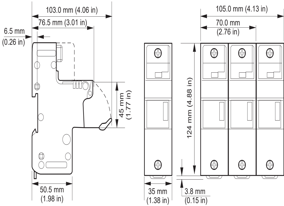
그림 35 퓨즈 홀더 치수: US221 (22x58mm)
