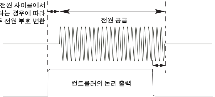
그림 13 논리 점호 모드
