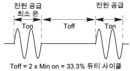
그림 15 버스트 가변 점호
