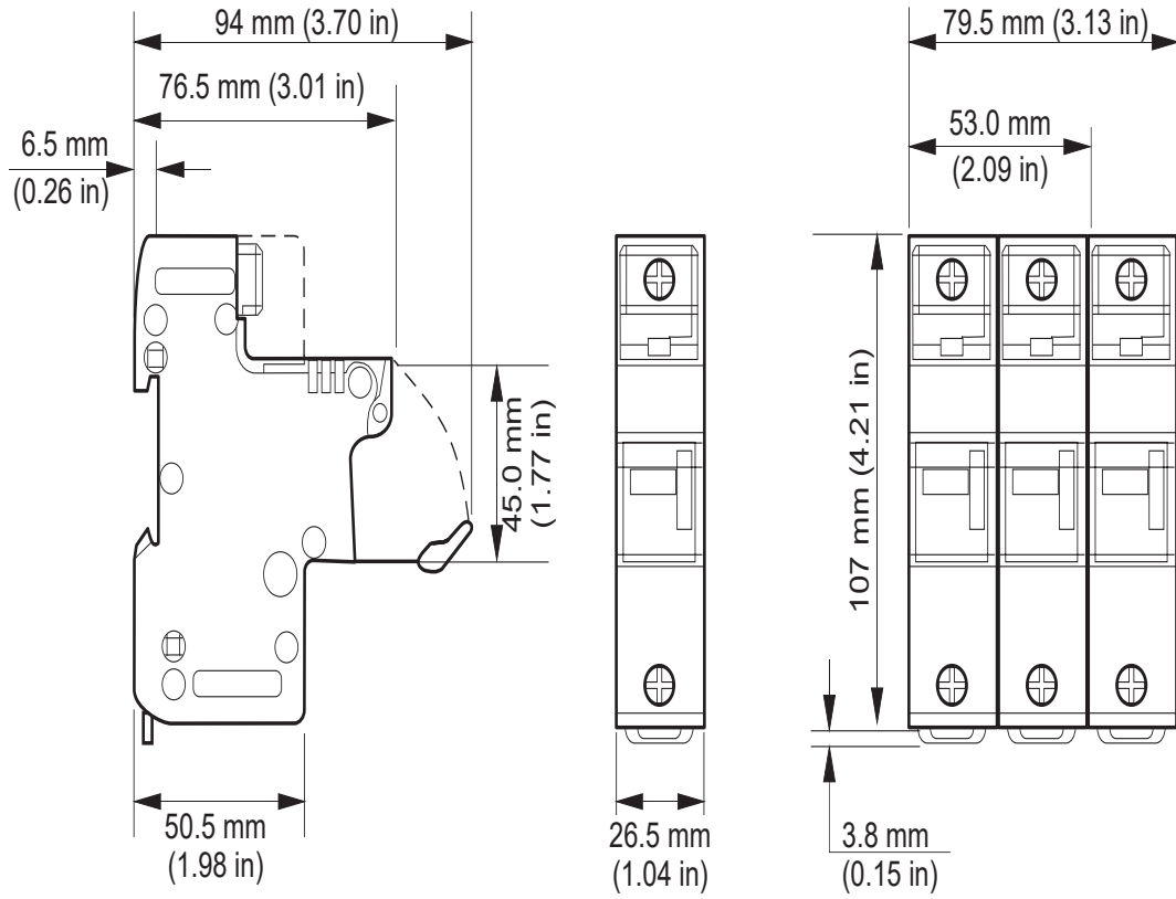
그림 34 퓨즈 홀더 치수: US141 (14x51mm)
