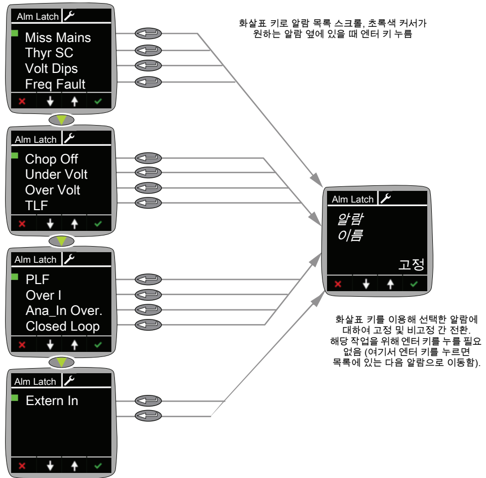
그림 26 알람 고정 메뉴
