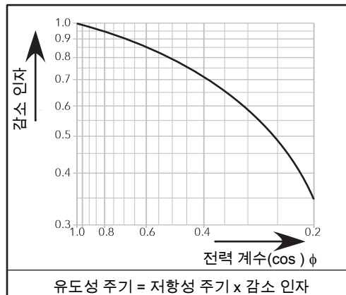
그림 37 릴레이 디레이팅 곡선
