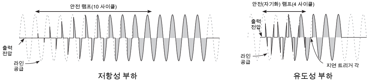
그림 19 안전 램프(버스트 접호) 예시
