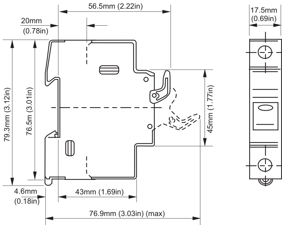
그림 33 퓨즈 홀더 치수: CUS101 (10x38mm)
