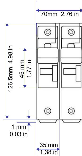
그림 37 퓨즈 홀더 치수: US222 (22x58mm)
