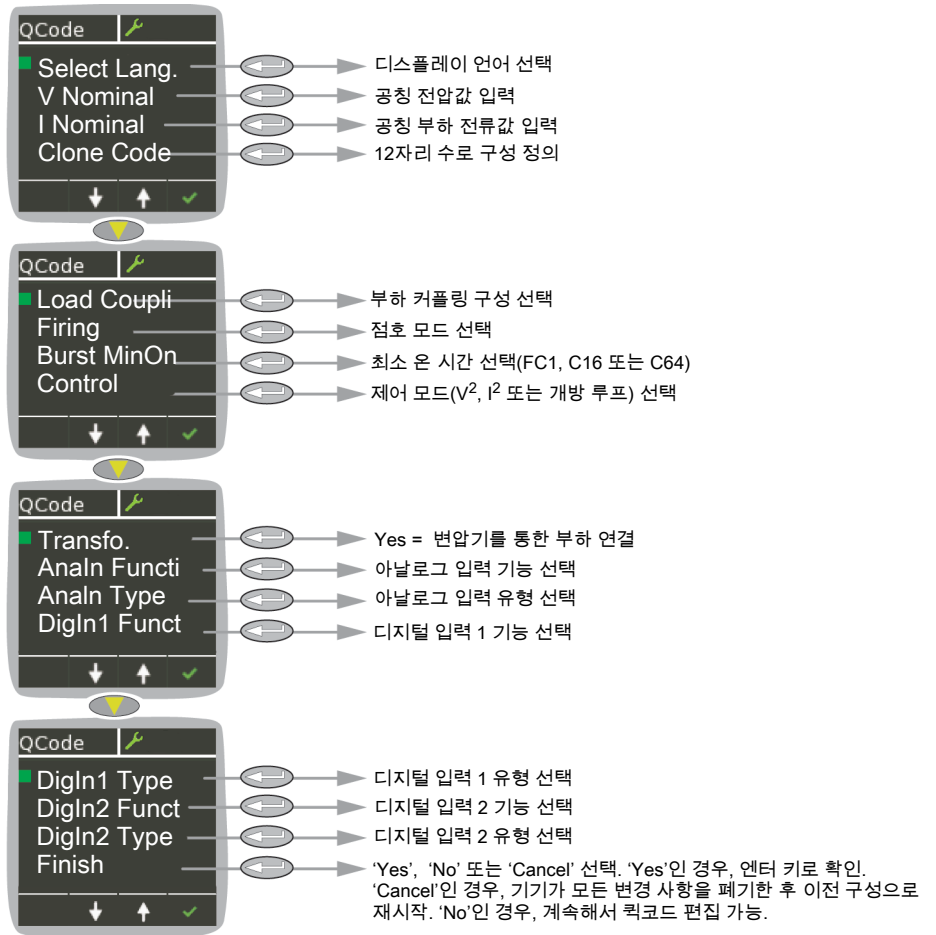
그림 14 일반적인 퀵코드 메뉴
