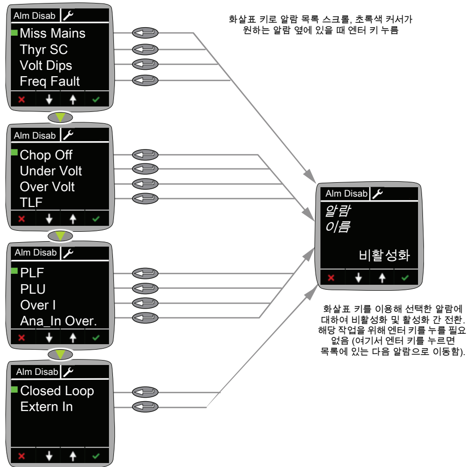
그림 27 알람 비활성화 메뉴
