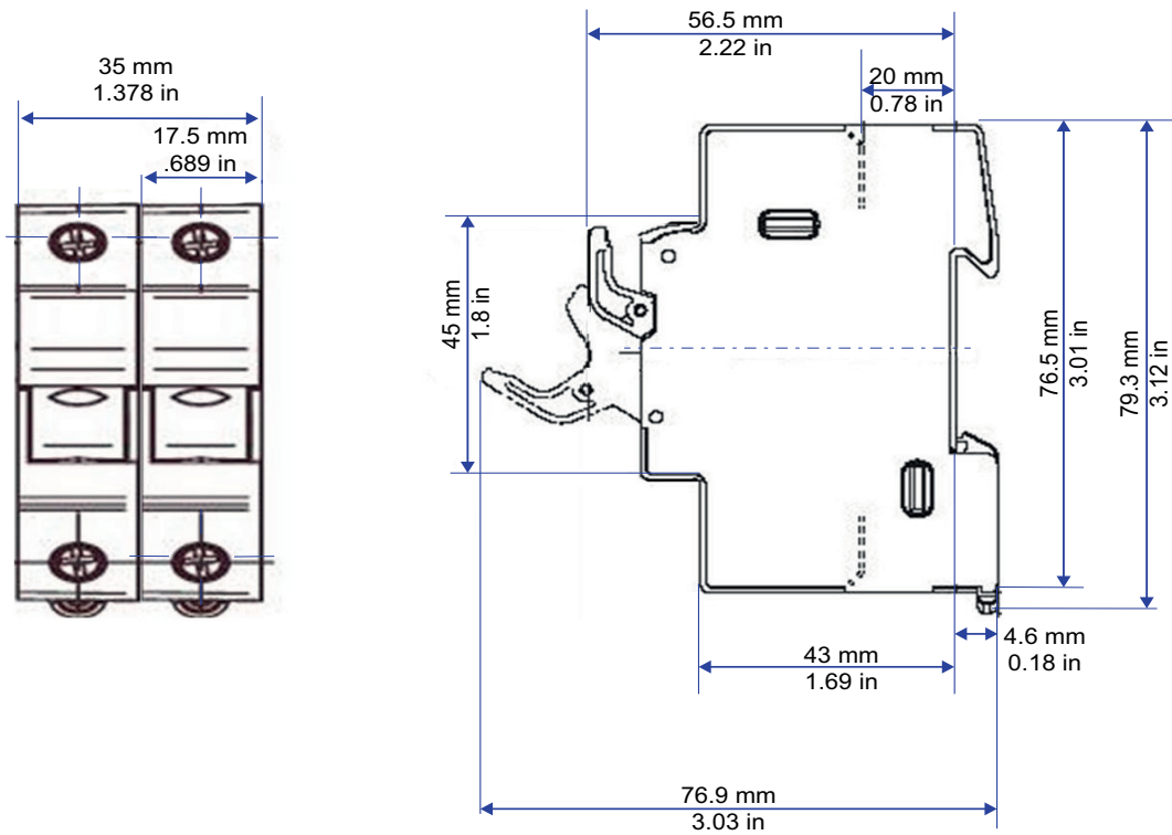
그림 35 퓨즈 홀더 치수: CUS102 (10x38mm)
