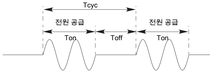
그림 16 버스트 고정 점호
