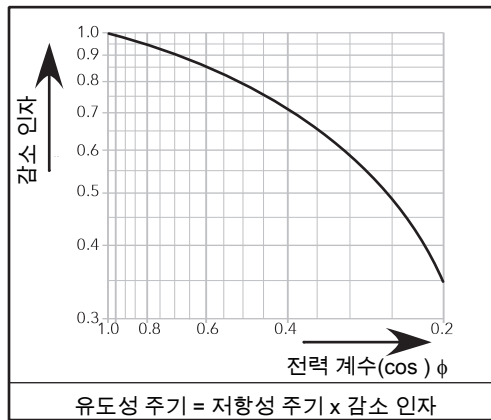
그림 40 릴레이 디레이팅 곡선
