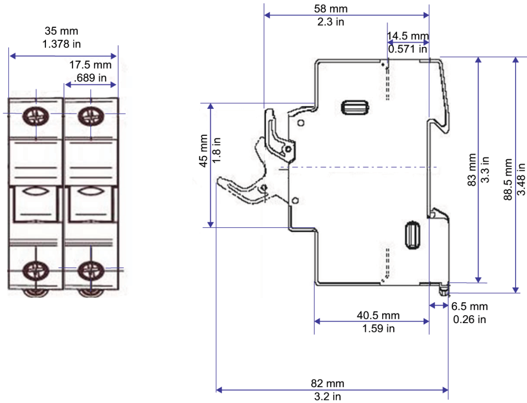
그림 34 퓨즈 홀더 치수: US102 (10x38mm)
