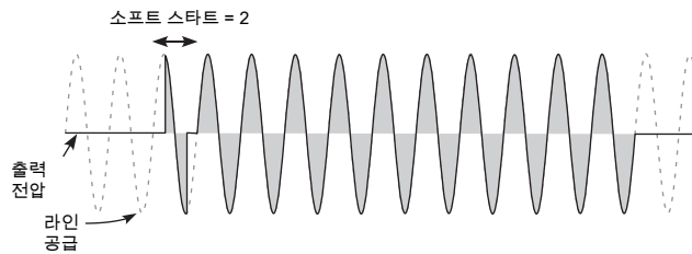
그림 22 소프트 스타트 예시
