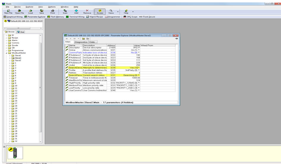
6. 将“Search device”参数值设置为“是”，检查设备是否在线。搜索状态不应为“Searching（搜索）（0）”。
